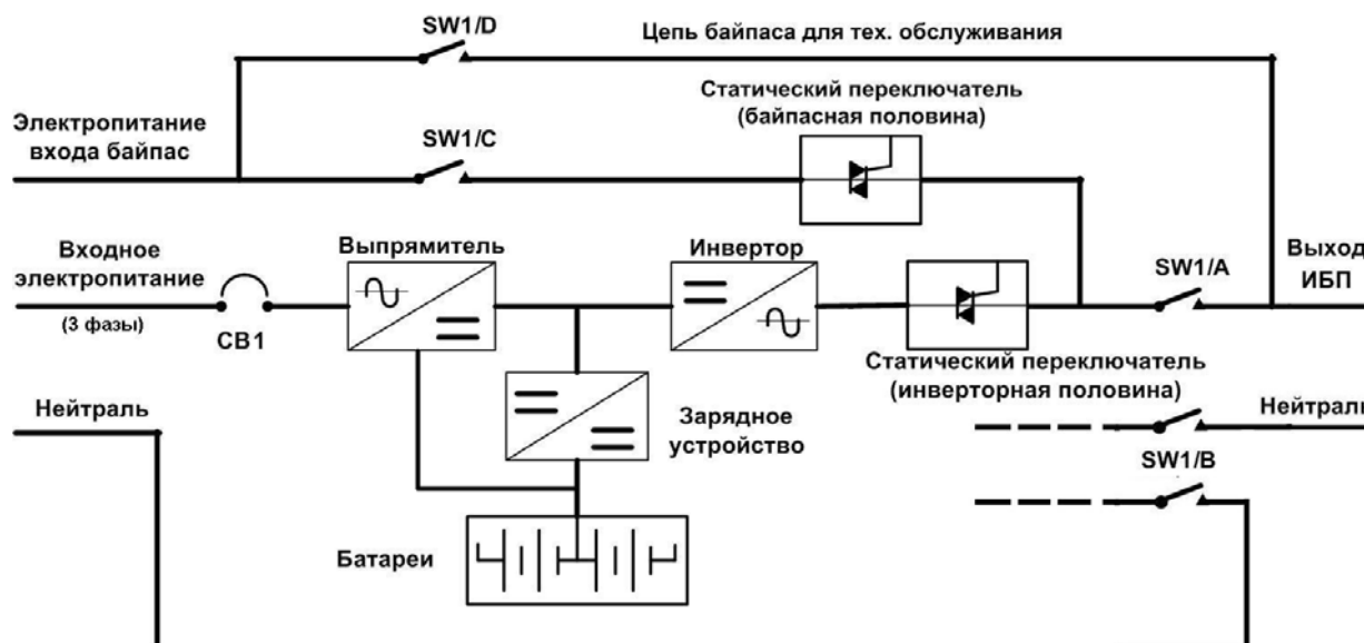
Рисунок 28 - Блок-схема одиночного модуля ИБП с раздельным подключением по входу
