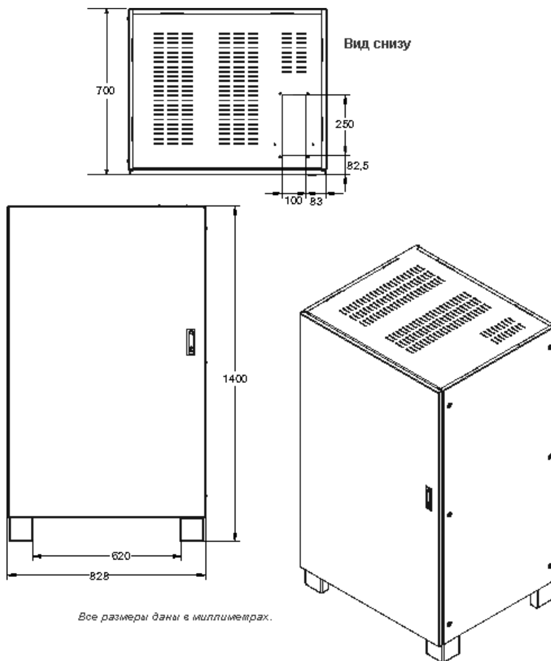
Рисунок 8 – Габаритные размеры батарейного шкафа и место подвода проводников
