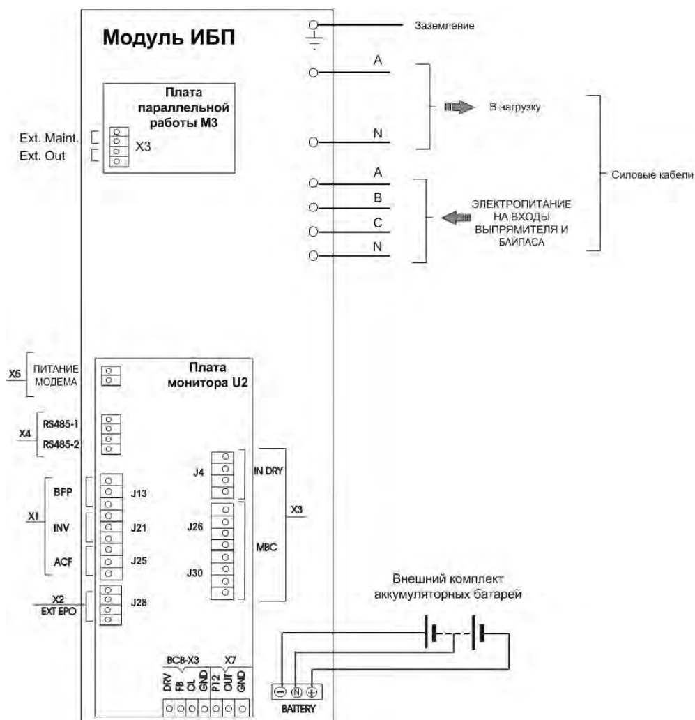
Рисунок 21 - Электрические соединения
