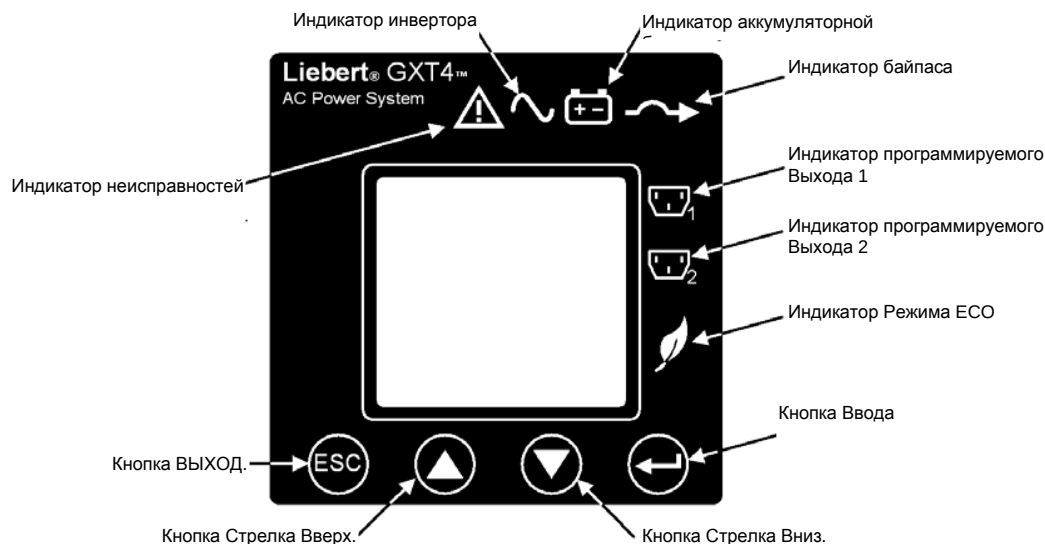
Рис. 12 Панель управления и индикации
