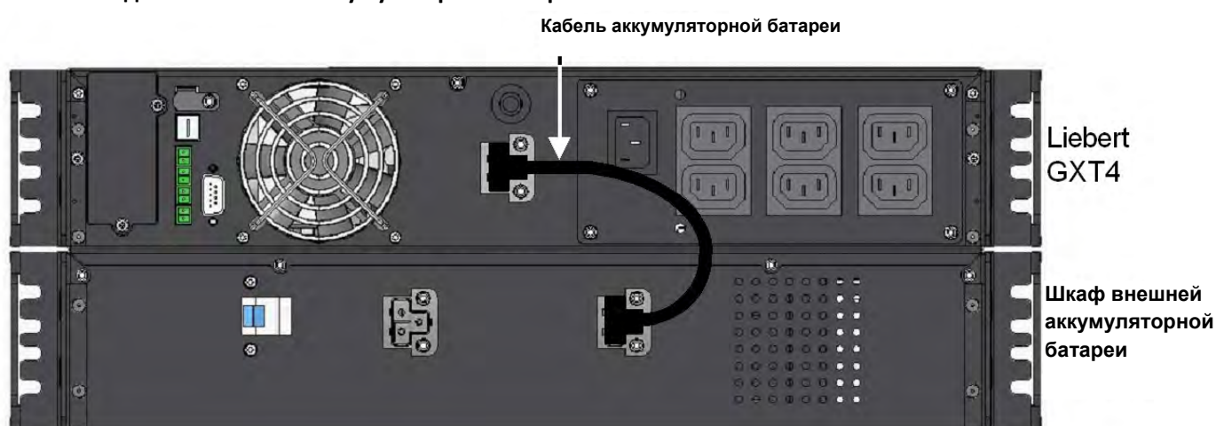
Рис.11 Соединение кабеля аккумуляторной батареи
