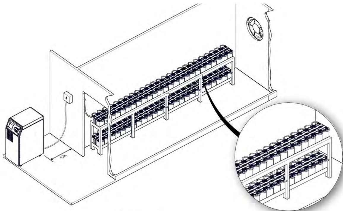
Örnek Akü Odası Uygulaması 3L1020R010R0
