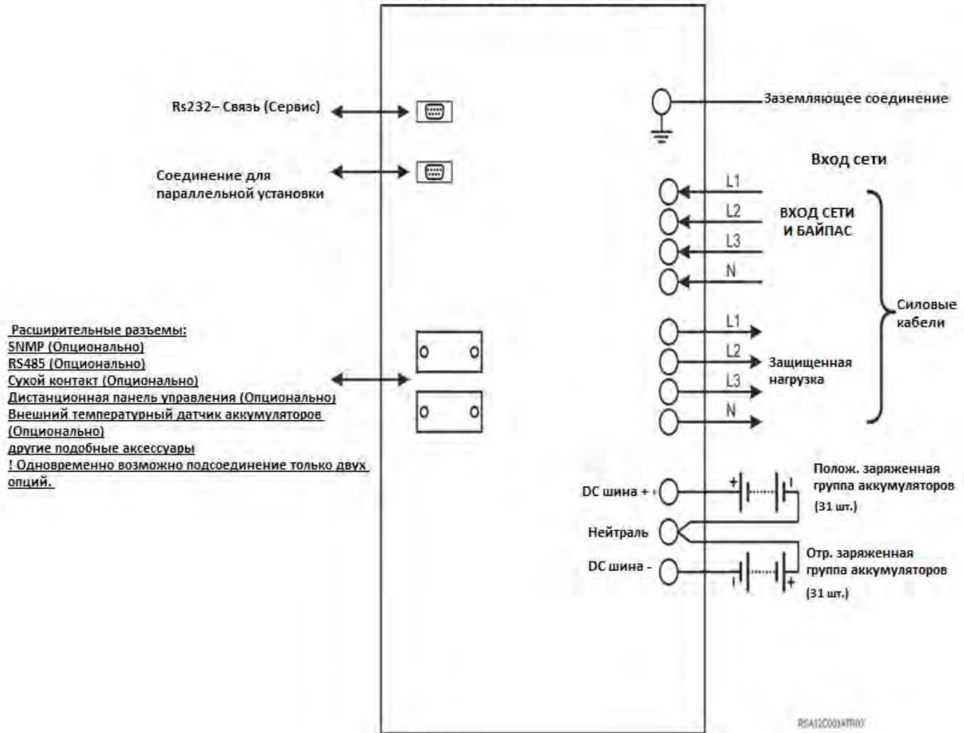
Электрические соединения ИБП Voxer
