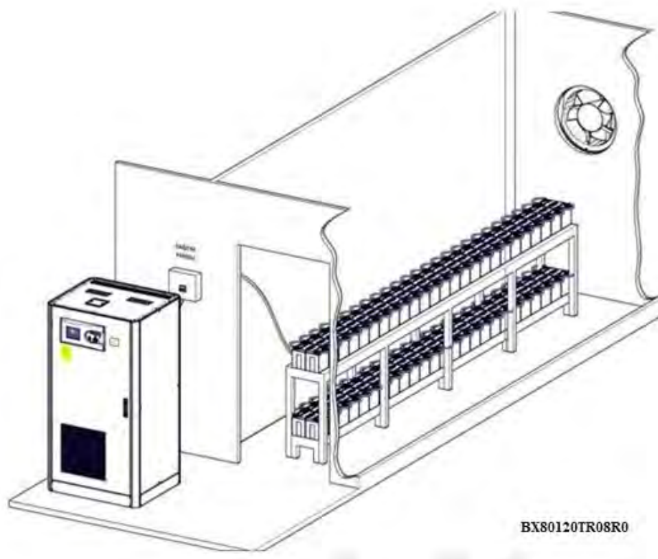
Пример применения помещения для аккумуляторов
