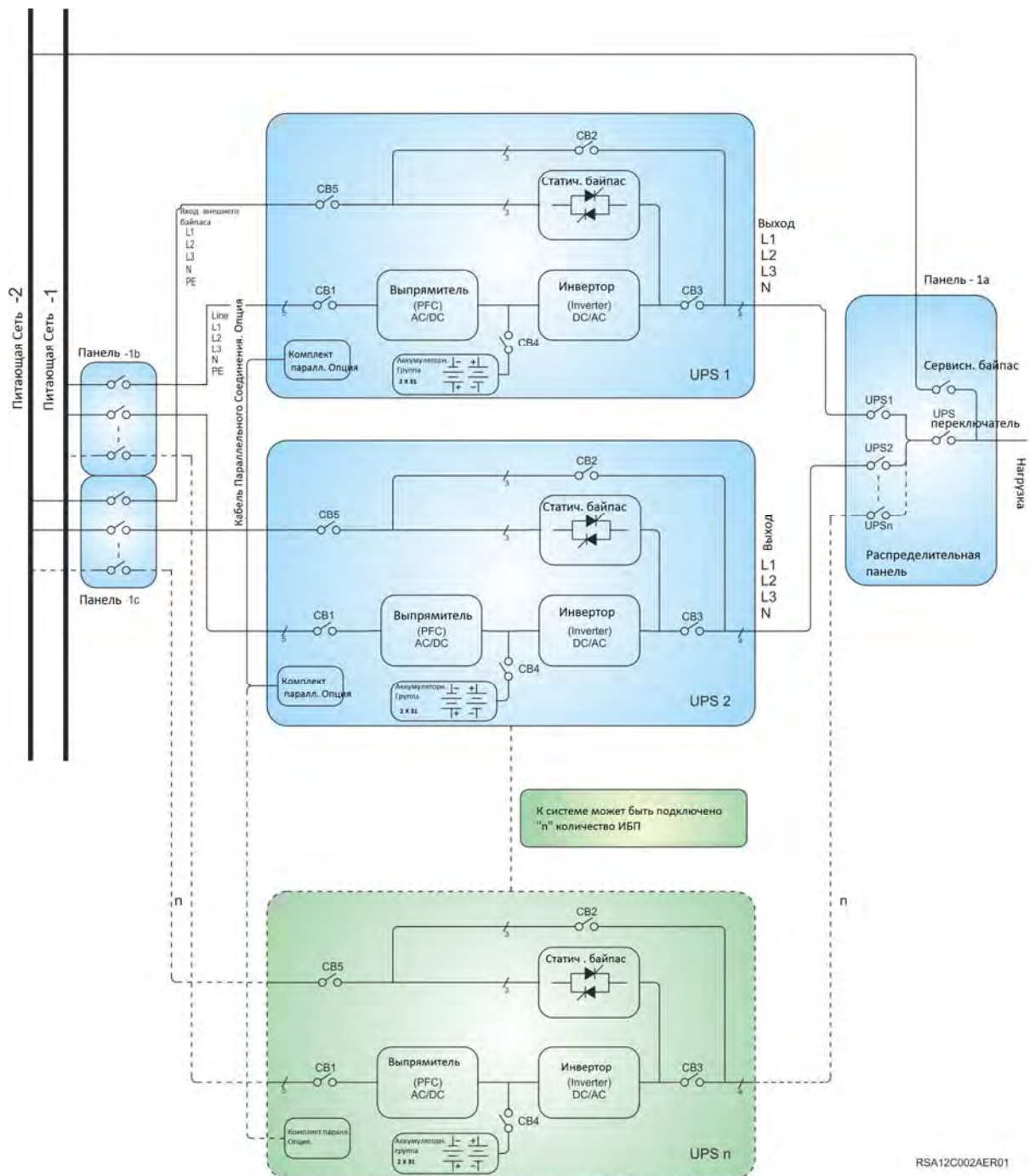
Схема опционального соединения
