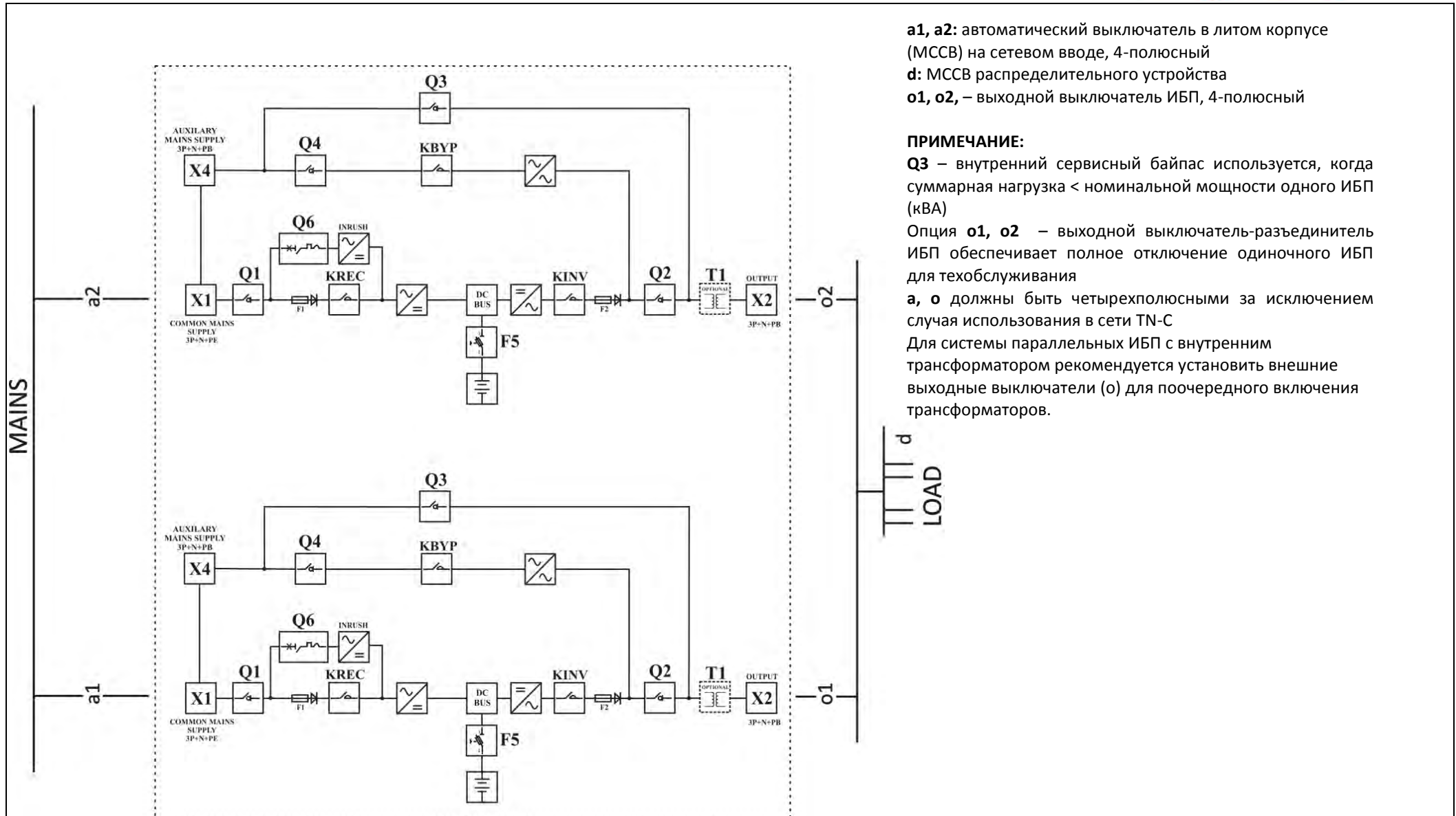
Конфигурация с резервированием 1+1 с двумя параллельными ИБП (10-60 кВА) и одним вводом от распределительного устройства
