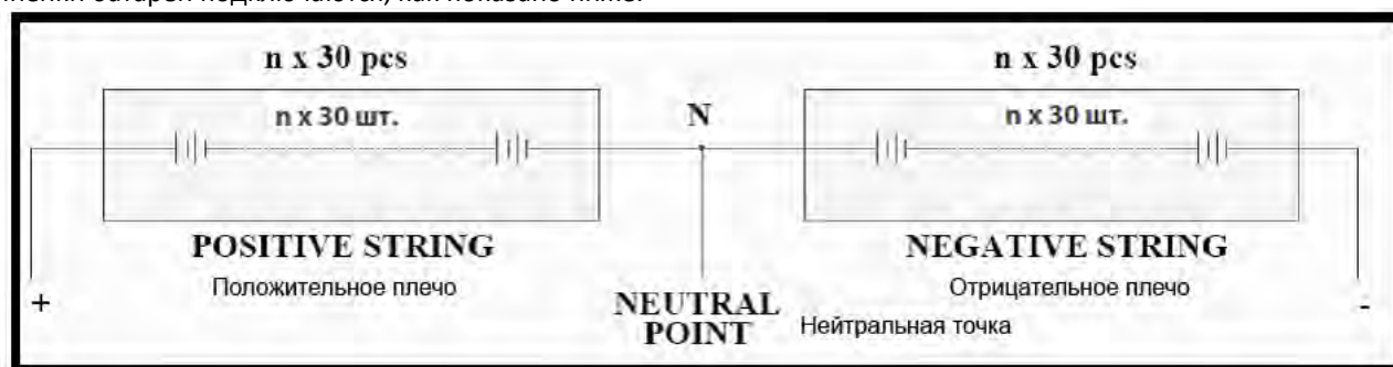
Два плеча и нейтральная точка
