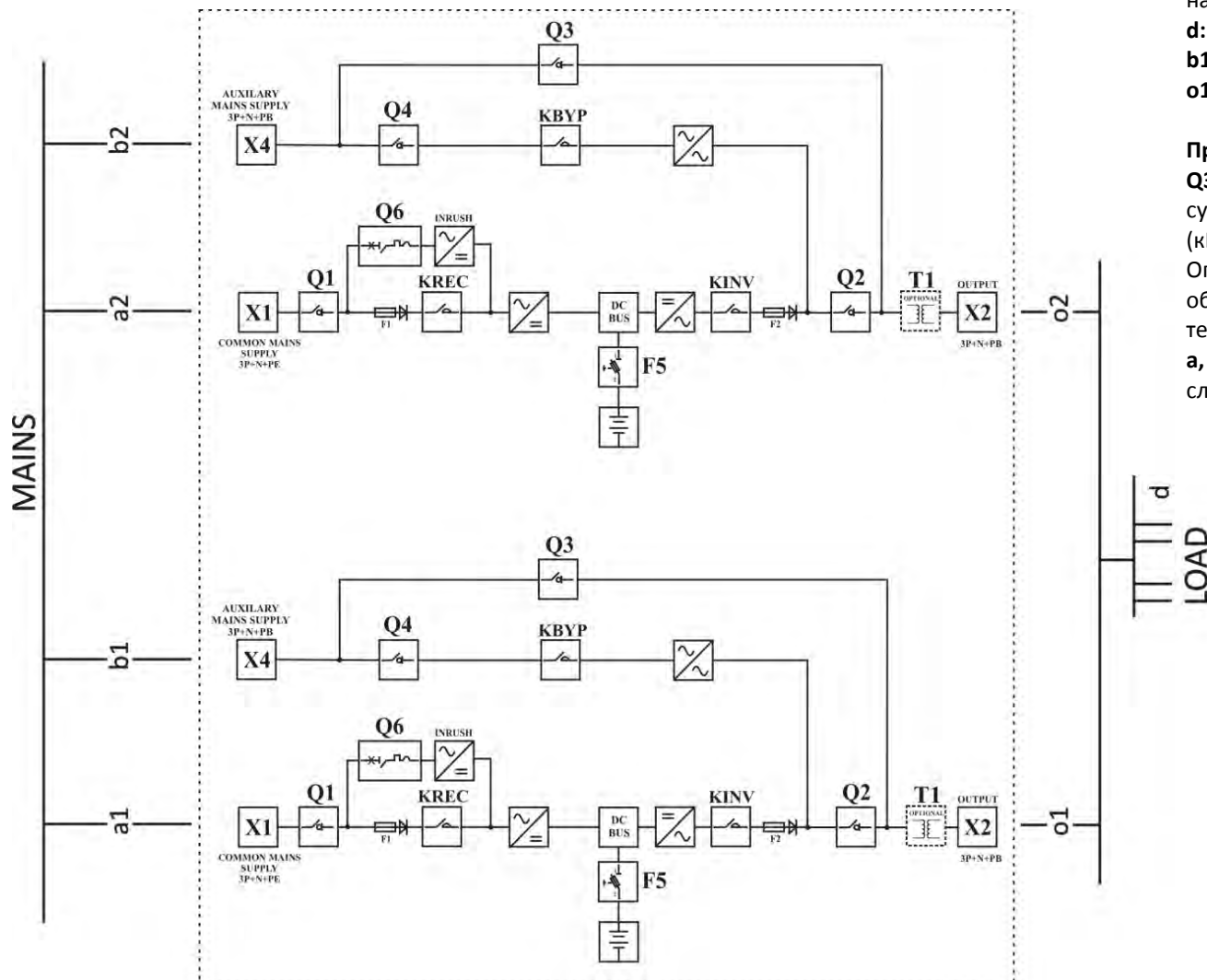
Конфигурация с резервированием 1+1 с двумя параллельными ИБП (10-60 кВА) и двумя вводами от распределительного устройства
