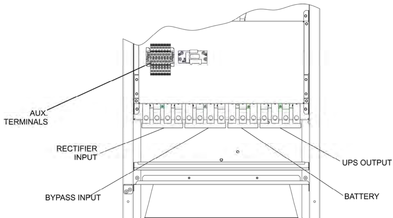
Figura 8bis – Morsettiera KEOR HPE 125-160 kVA
