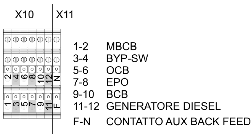
Figura 18 – Morsetti ausiliari KEOR HPE 60÷160 kVA
