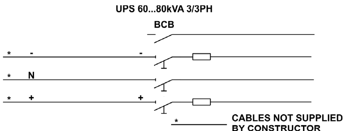
Illustration 9 – Câblage du porte-fusible BCB
