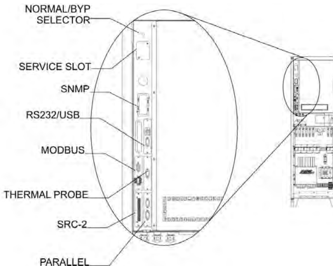
Illustration 19 – Position des interfaces de série du KEORHPE 60÷160 kVA
