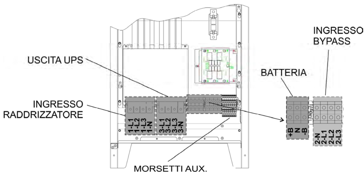
Figura 8 – Morsetti KEOR HPE 100 kVA
