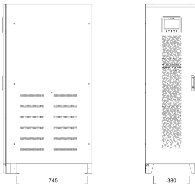
Illustration 2 – Manutention de l'ASI KEOR HPE 60÷160 kVA
