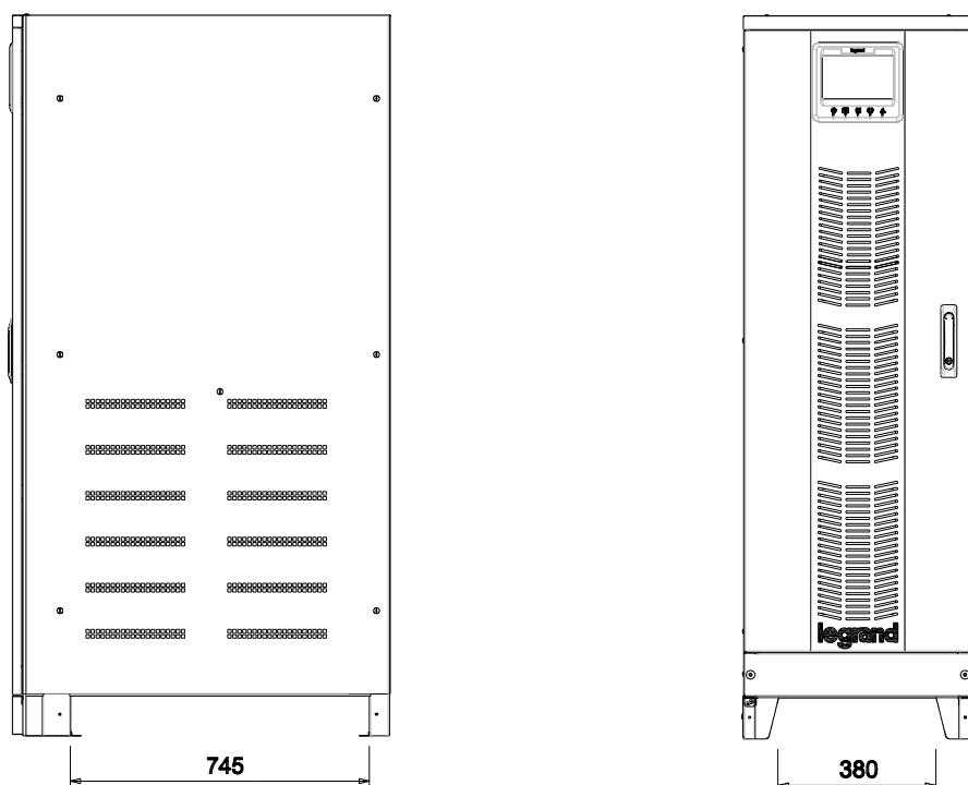
Figura 2 – Movimentazione UPS KEOR HPE 60÷160 kVA
