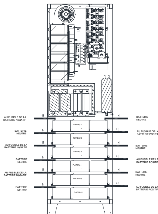
Illustration 13- 7/9/11Ah 12V batterie connexion vue frontale
