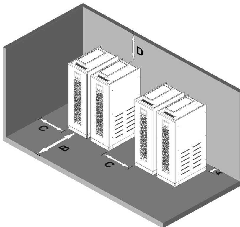
Illustration 5 – Dégagement minimum
