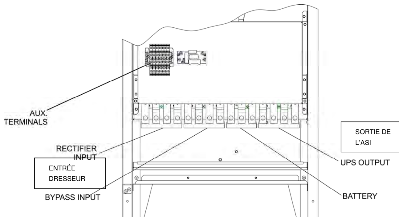
Illustration 8 bis – Borniers KEOR HPE 125-160 kVA
