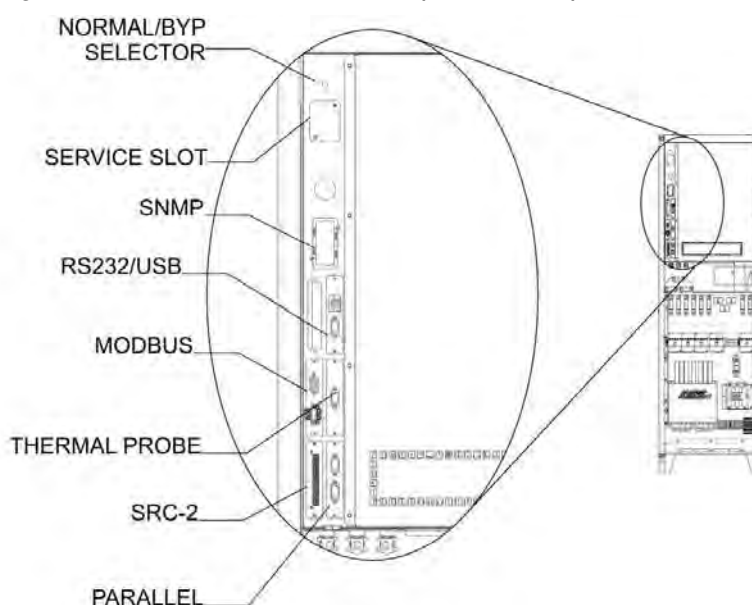
Figura 19 – Posizione schede di interfaccia
