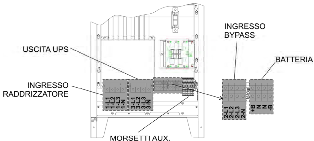
Figura 7 – Morsetti KEOR HPE 60-80 kVA
