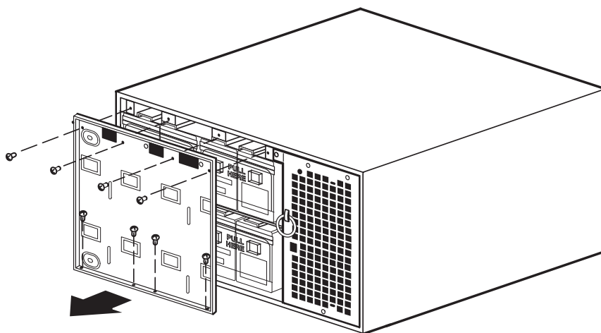
Рисунок 57. Снятие крышки аккумуляторов ИБП
