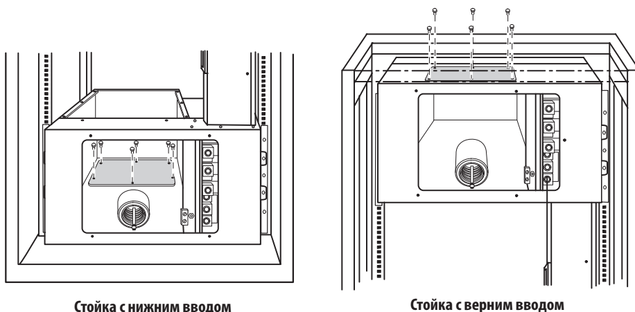
Рисунок 7. Удаление посадочной пластины кабелепровода
