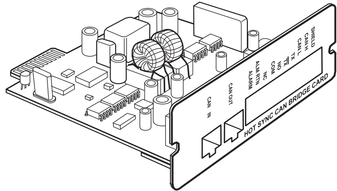
Рисунок 33. Плата Powerware Hot Sync CAN Bridge
