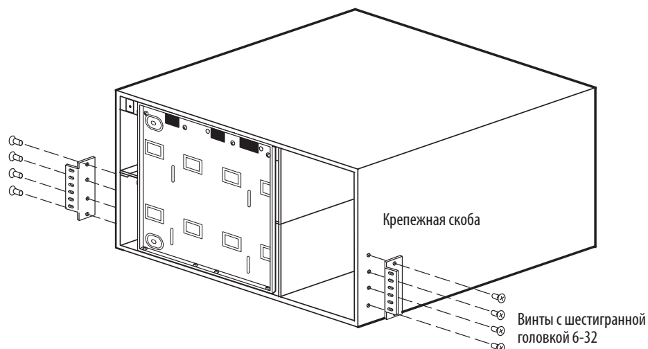
Рисунок 22. Установка крепежных скоб ИБП
