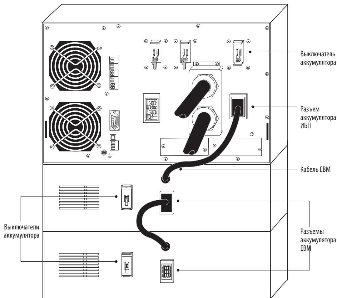
Рисунок 29. Типовая установка EBM
