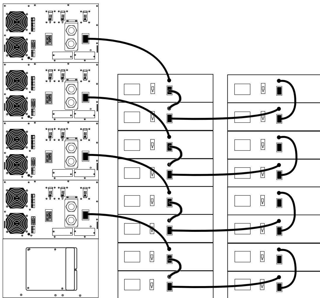
Рисунок 31. Пример установки ЕВМ в большой параллельной система
