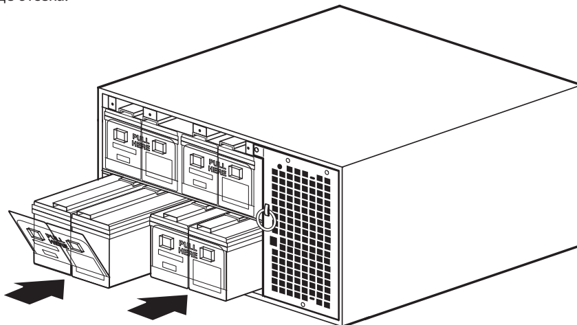
Рисунок 58. Установка аккумуляторных отсеков ИБП
