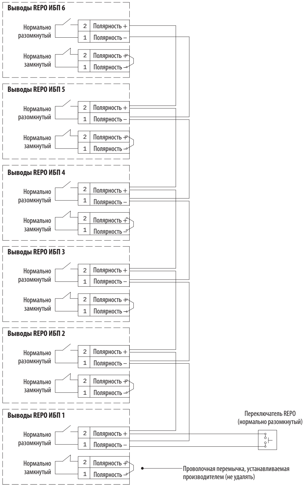
Рисунок 54. Подключение нормально разомкнутого REPO в параллельной системе
