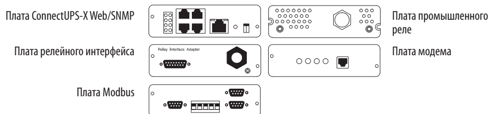
Рисунок 50. Дополнительные платы X-Slot
