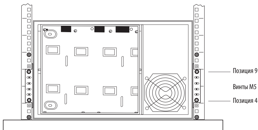
Рисунок 23. Прикрепление передней части ИБП
