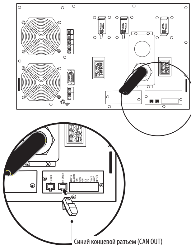
Рисунок 35. Установка синего концевой разъема (последний ИБП)
