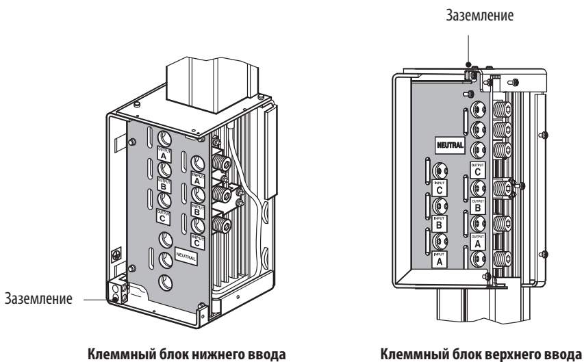
Рисунок 8. Клеммный блок шины BladeUPS
