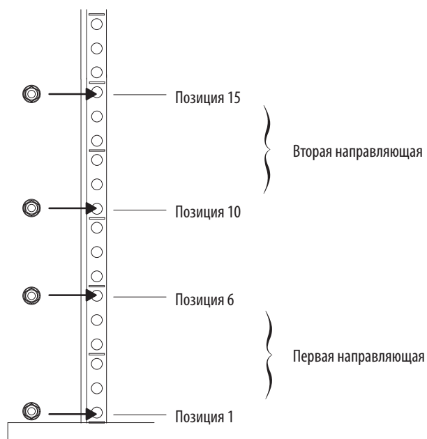
Рисунок 10. Положения винтов передней направляющей для ЕВМ
