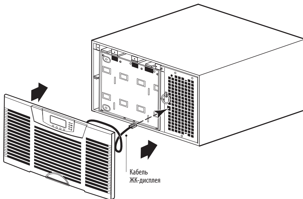
Рисунок 59. Установка передней крышки ИБП
