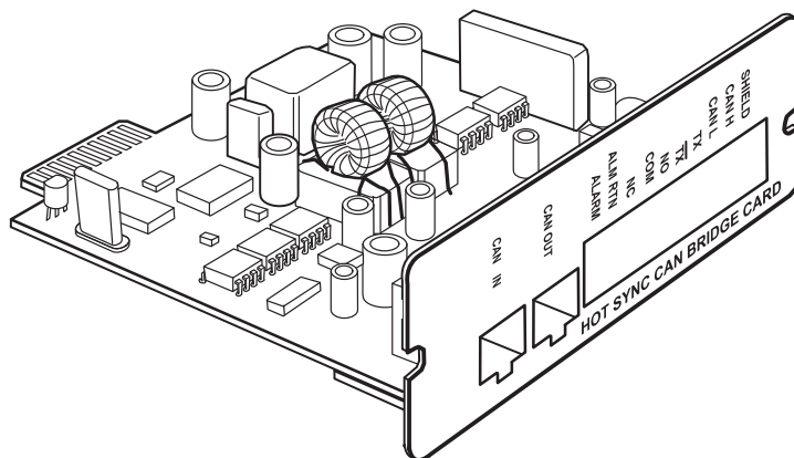
Рисунок 41. Плата Powerware Hot Sync CAN Bridge
