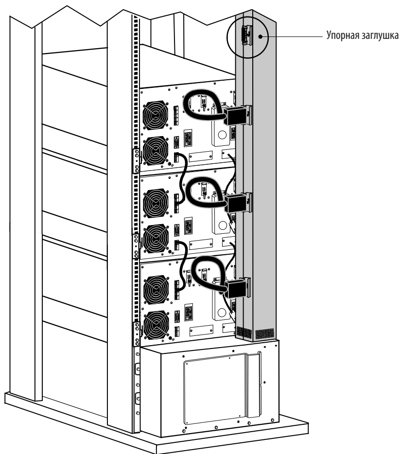
Рисунок 37. Подключение нескольких ИБП к шине BladeUPS (показан нижний ввод)
