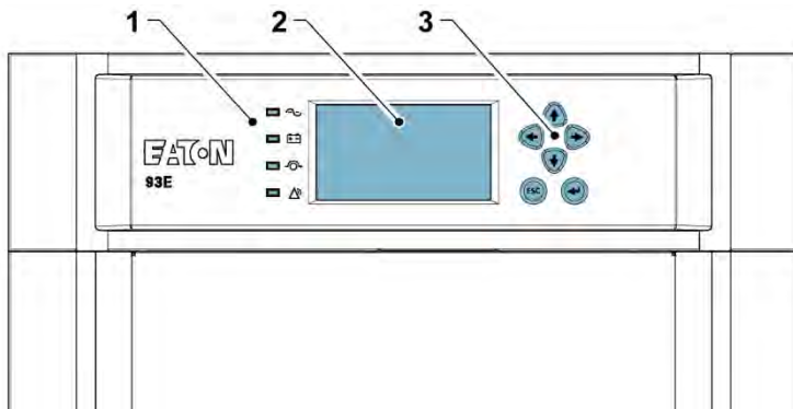
Рис. 38. Панель управления ИБП
