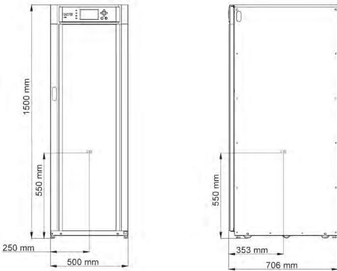
Рис. 12. Центр тяжести ИПБ шкафа (Eaton 93E на 40 кВА) с аккумуляторами
