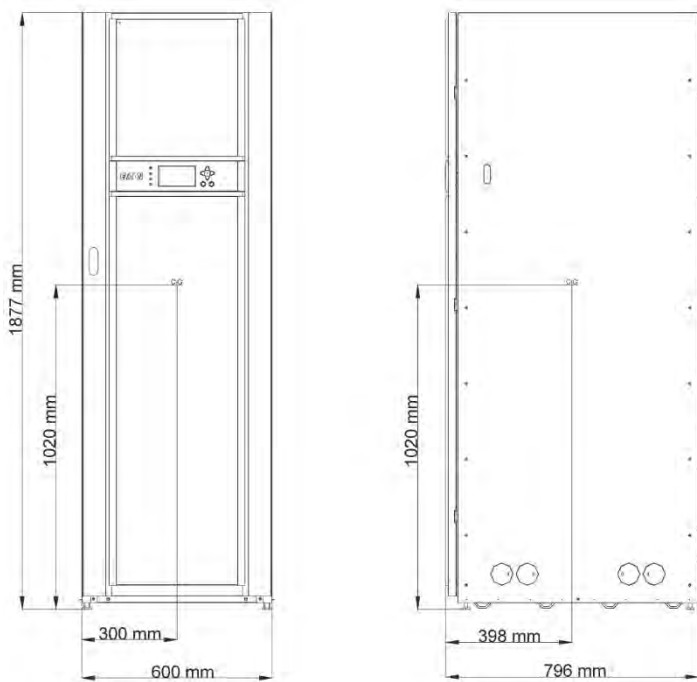
Рис. 14. Центр тяжести ИБП шкафа (Eaton 93E на 80 кВА)
