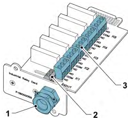
Рисунок 27. Реле
