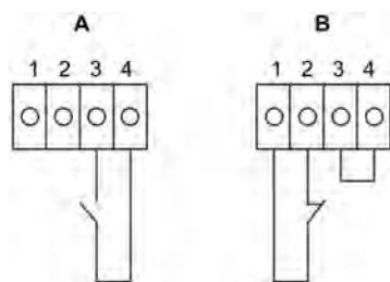
Рисунок 13. Соединения для выключателя EPO
