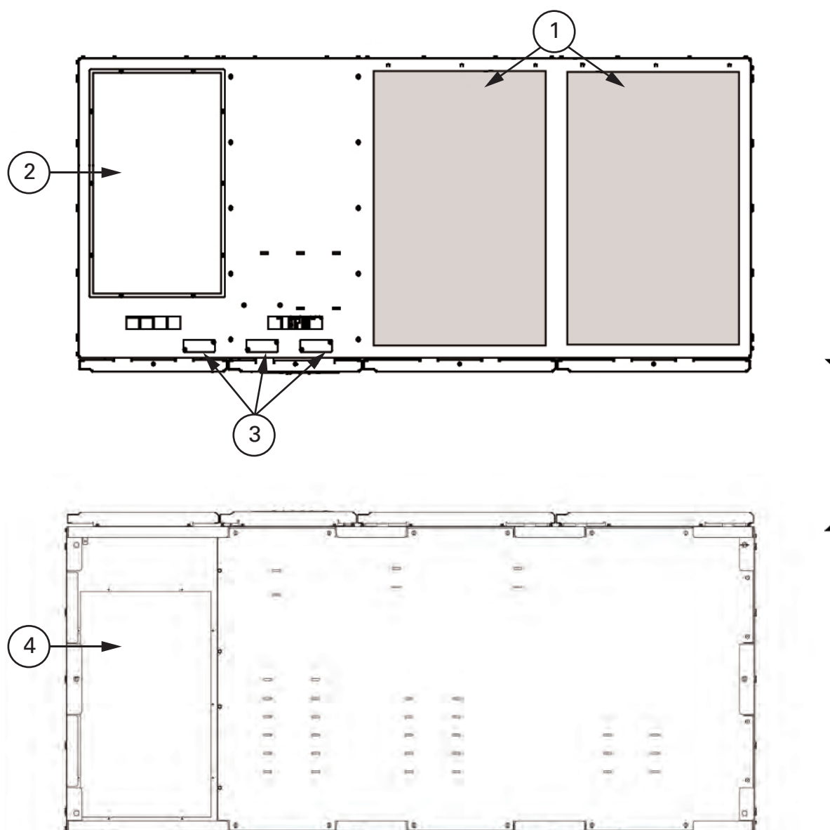
Рис. 4-4. Расположение входов проводки
