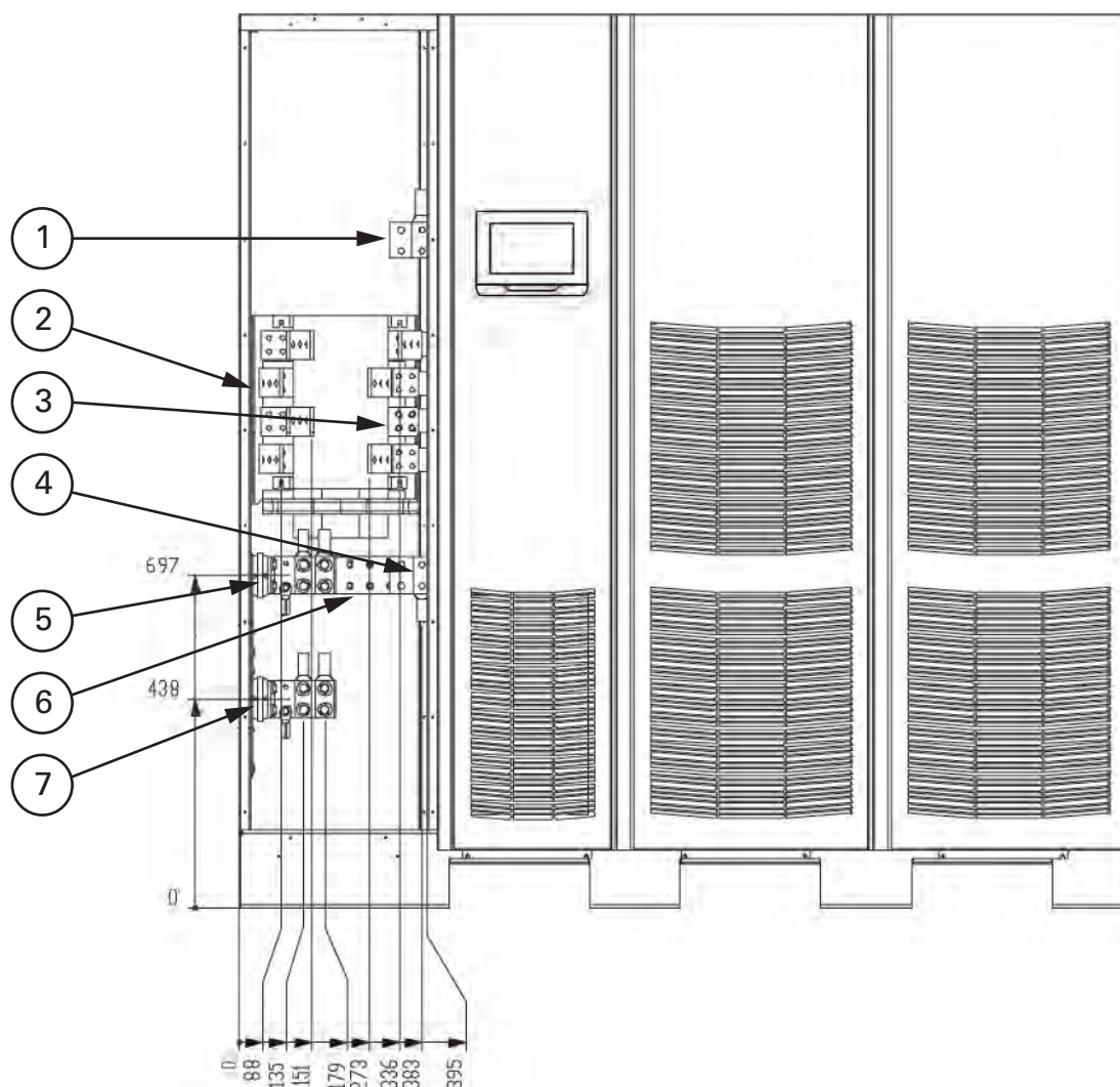
Рис. 4-7. Вид спереди
