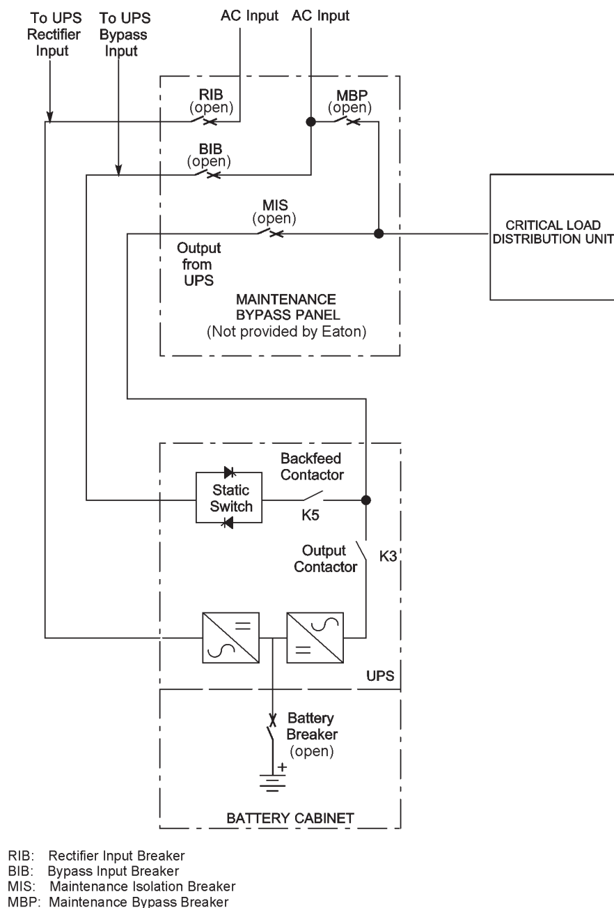
Рис. 6-10. Упрощенная схема ИБП с двойной подачей и панелью сервисного байпаса
