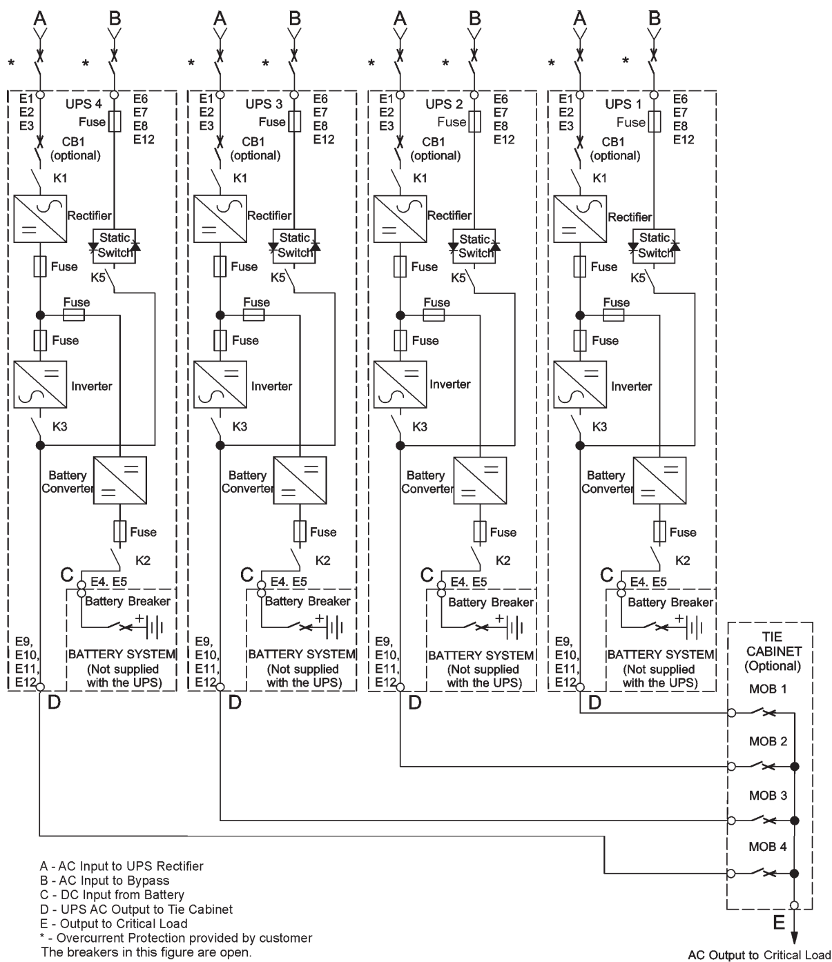
Рис. 6-16. Типовая система с распределенным байпасом (конфигурации 3+1 и 4+0)
