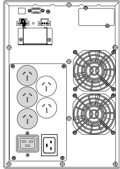
Рисунок 60. Модель PW9130G3000T-XLAU
