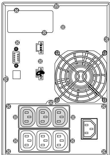
Рисунок 51. Модель PW9130i700T-XL
