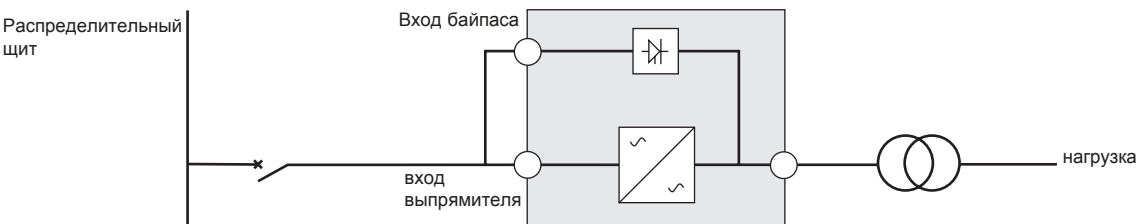
ИБП с общим вводом на вход выпрямителя и вход байпаса с трансформатором гальваноразвязки (Рис. 10)
