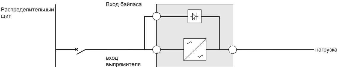
ИБП с Конфигурация ИБП с общим вводом на вход выпрямителя и на вход байпаса (Рис. 9)
