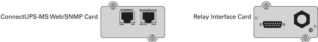
Рисунок 23. Дополнительные коммуникационные карты.
