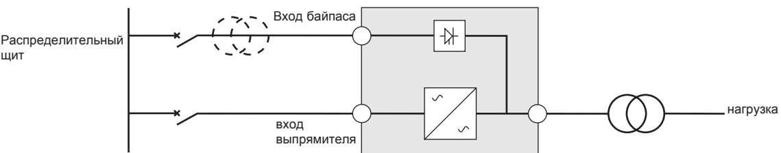
ИБП с отдельным входами байпаса и выпрямителя и с трансформатором гальваноразвязки (Рис. 12)
