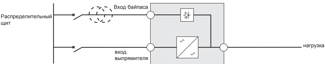
ИБП с отдельными входами байпаса и выпрямителя (Рис. 11)
