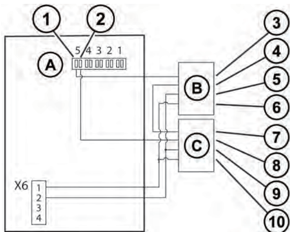
Рисунок 27. Проводка распределителя аккумулятора для модели ИБП 93PM 200 кВт
