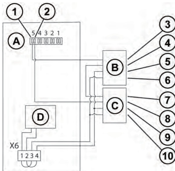
Рисунок 25. Проводка расцепителя аккумулятора для модели ИБП 93PM 50 кВт
