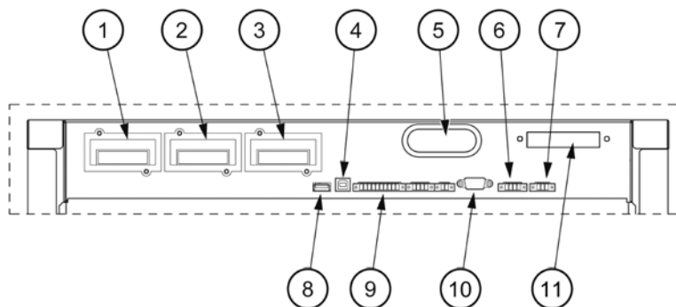
Рисунок 36. Интерфейсы связи
