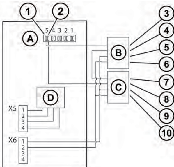
Рисунок 26. Проводка расцепителя аккумулятора для модели ИБП 93PM 100–150 кВт
