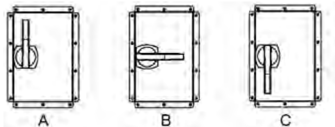
Рисунок 18. Положения переключателя MBS
