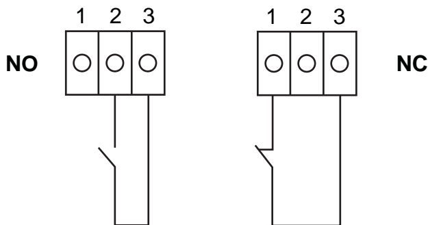
Рисунок 31. Подключения релейных контактов
