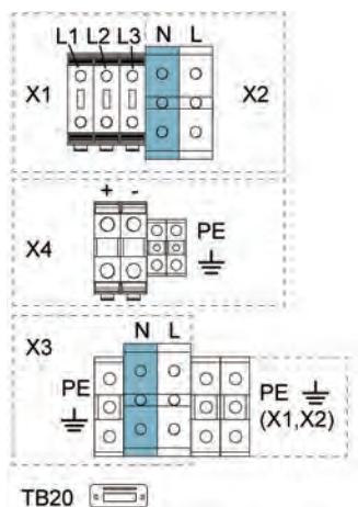
Рисунок 12. Зажимы силового кабеля в раме 91PS на 30 кВт с общим аккумулятором
