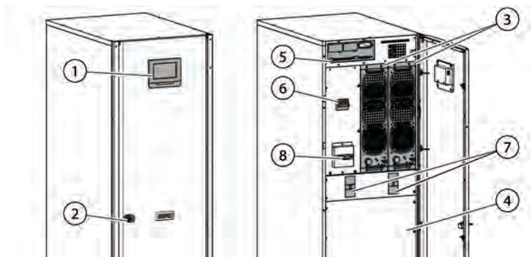
Рисунок 3. Внутренние компоненты рамы на 30/40 кВт
