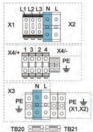
Рисунок 13. Зажимы силового кабеля в раме 91PS на 30 кВт с отдельным аккумулятором (опционально)
