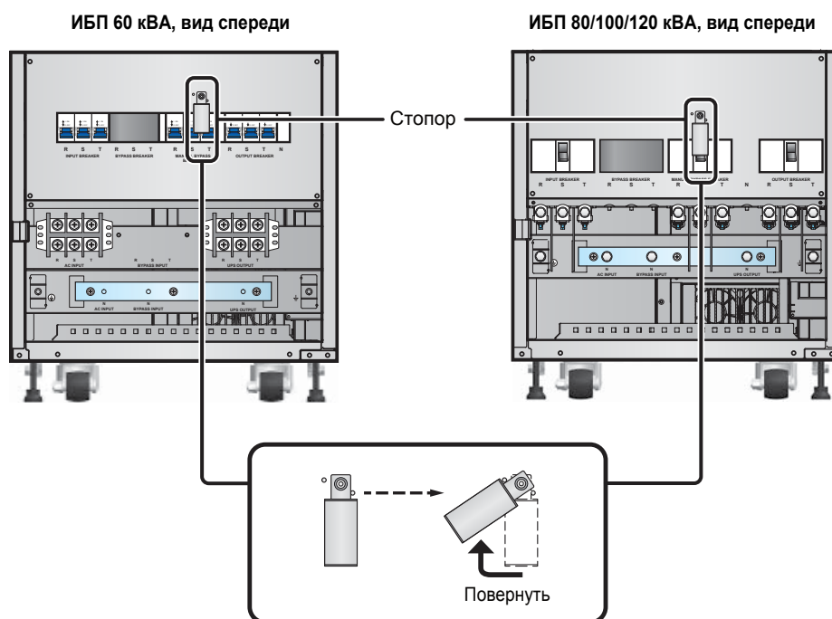
Рис. 7-1. Стопор ручного переключателя байпаса
