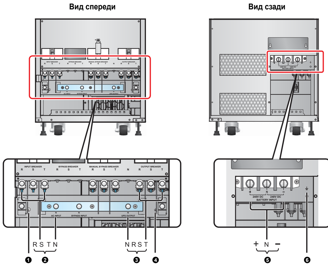
Рис. 6-8. Модель 100/120 кВА, блок зажимов
