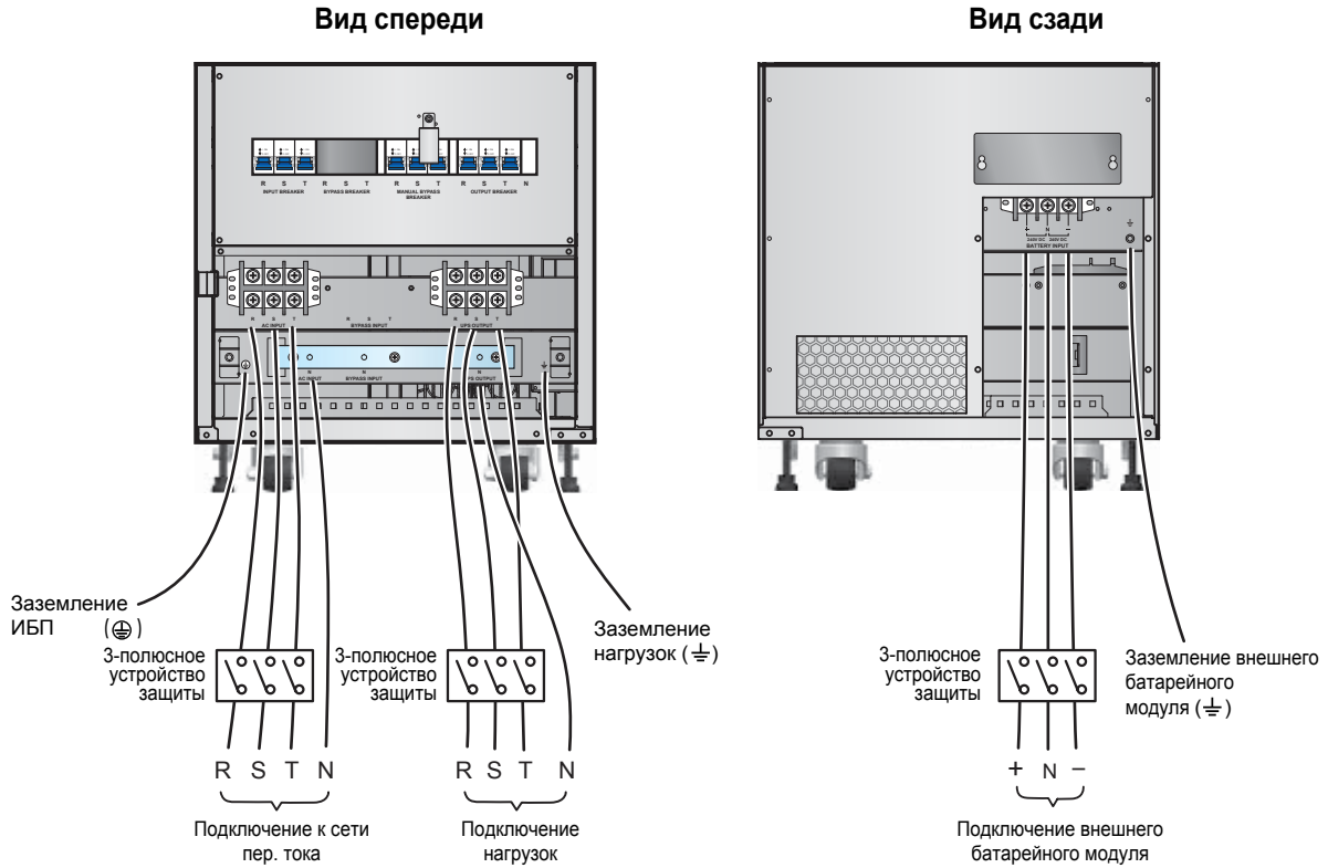
Рис. 6-9. Схема подключения одиночного ИБП 60 кВА в конфигурации с одним входом
