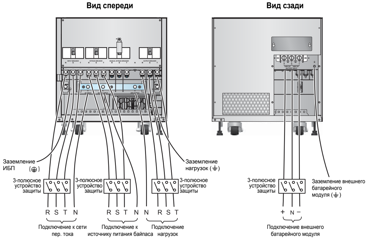
Рис. 6-12. Схема подключения одиночного ИБП 60 кВА в конфигурации с двумя входами
