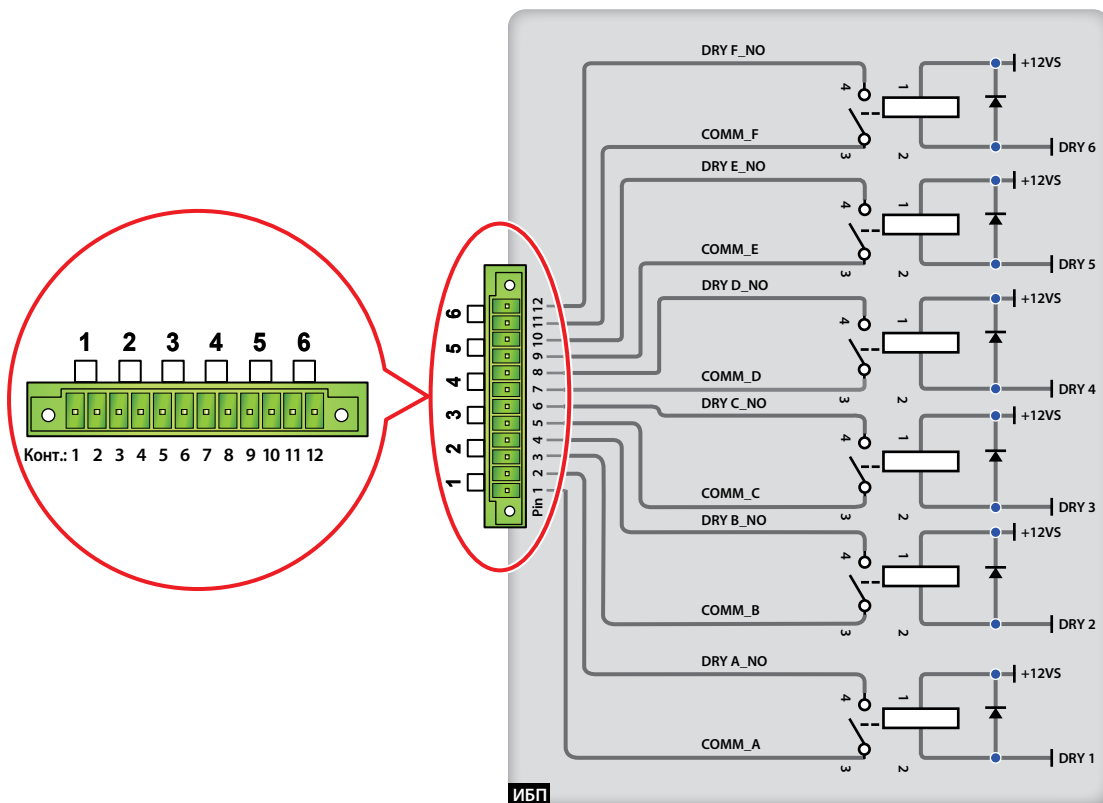
Рис. 5-9. Выходы с сухими контактами: назначение и подключение выводов
