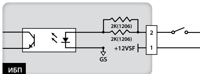
Рис. 5-5. Конфигурация порта REPO
