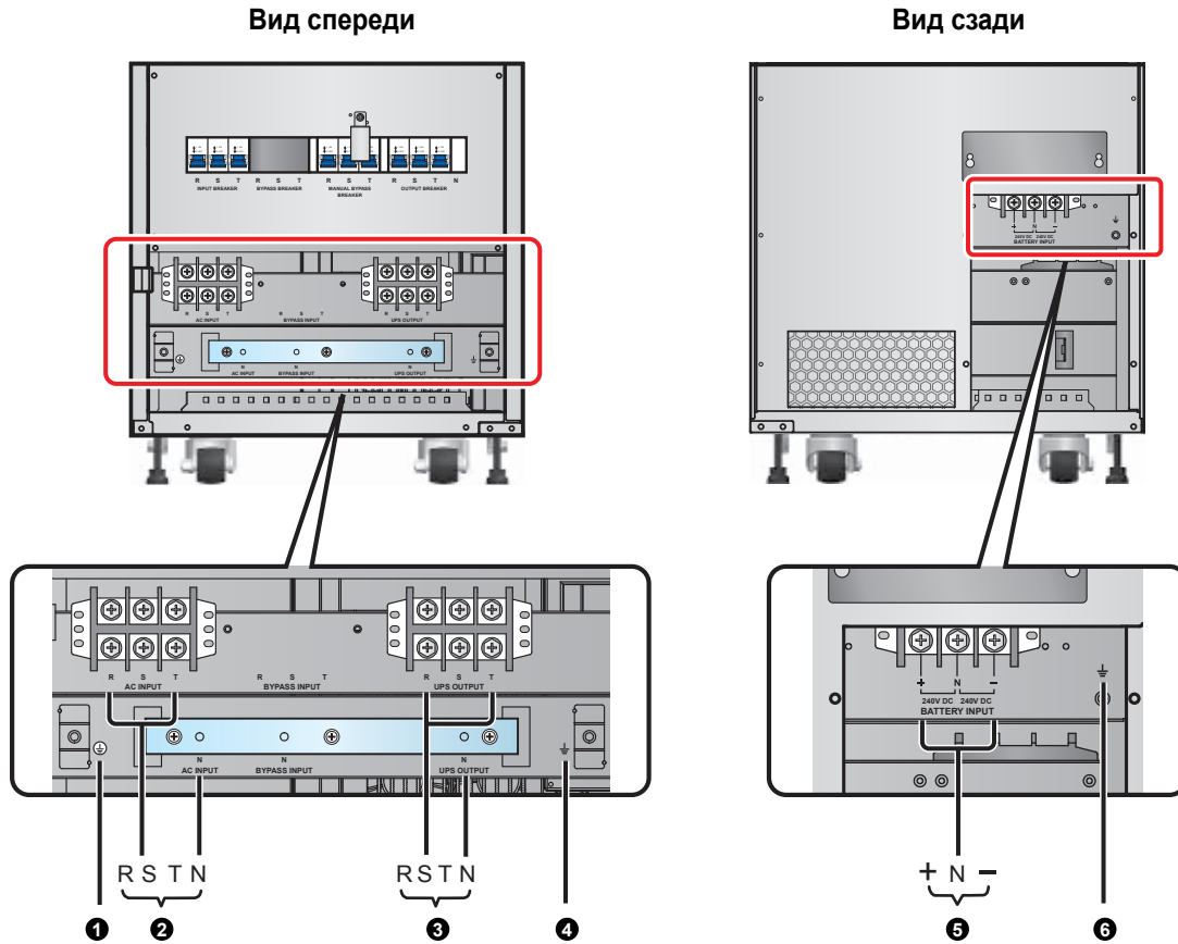
Рис. 6-6. Модель 60 кВА, блок зажимов
