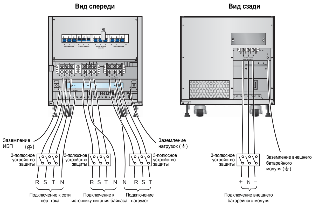
Рис. 6-14. Схема подключения одиночного ИБП 100/120 кВА в конфигурации с двумя входами
