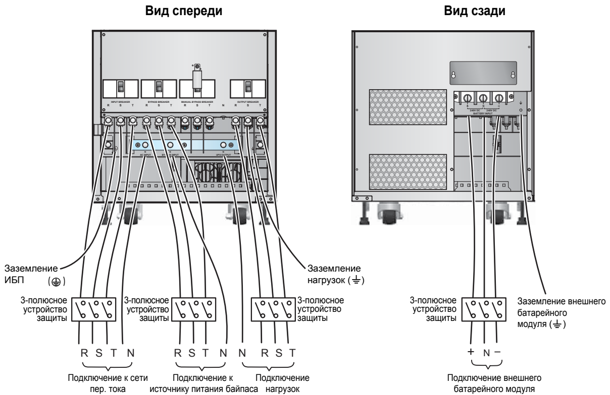
Рис. 6-13. Схема подключения одиночного ИБП 80 кВА в конфигурации с двумя входами
