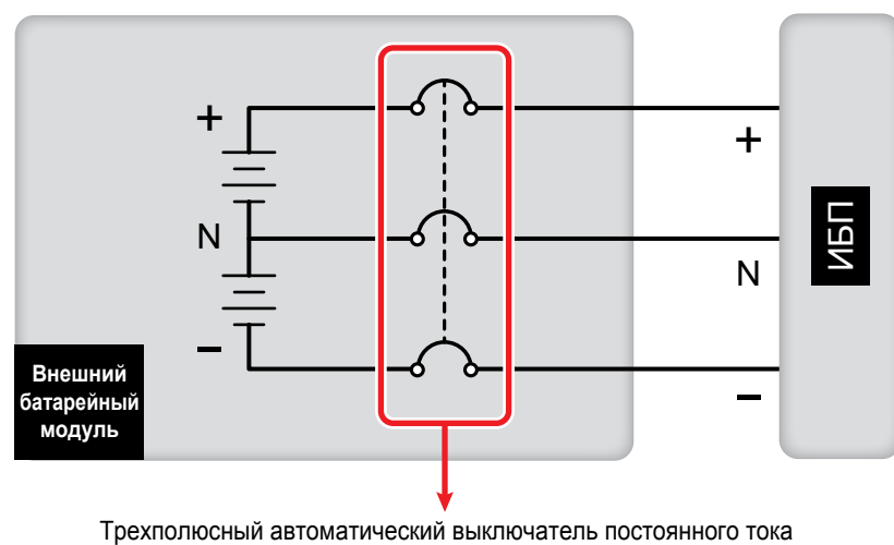
Рис. 6-20. Установка трехполюсного автоматического выключателя постоянного тока
