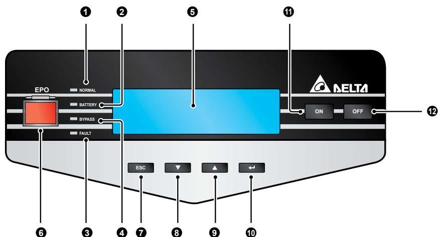
Рис. 3-4. Панель управления
