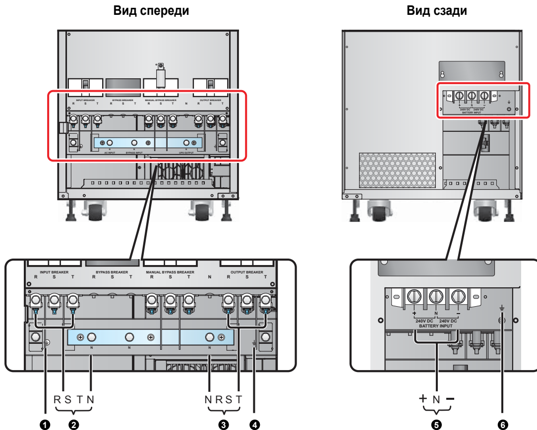
Рис. 6-7. Модель 80 кВА, блок зажимов
