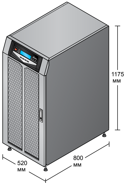
Рис. 3-1. Внешний вид и размеры ИБП 60/80 кВА
