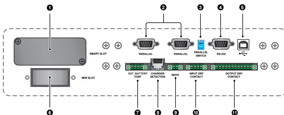
Рис. 5-2. Коммуникационные интерфейсы
