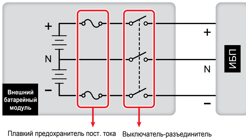
Рис. 6-18. Установка выключателя-разъединителя последовательно с плавким предохранителем постоянного тока
