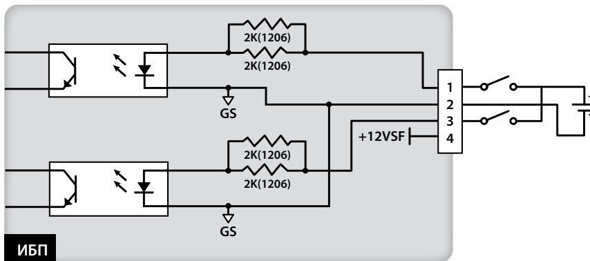
Рис. 5-8. Входы с сухими контактами, конфигурация II
