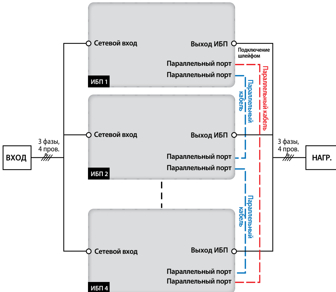
Рис. 6-15. Схема подключения в конфигурации с одним входом (параллельные ИБП)
