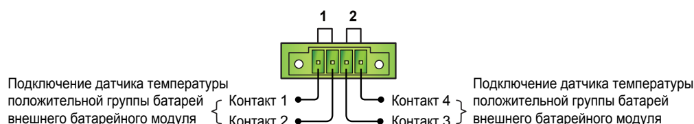
Рис. 5-5. Порты датчиков температуры внешнего батарейного модуля
