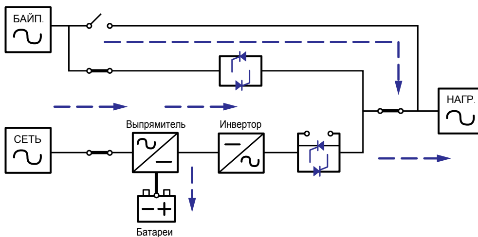
Рис. 4-3. Передача электроэнергии через ИБП в режиме готовности
