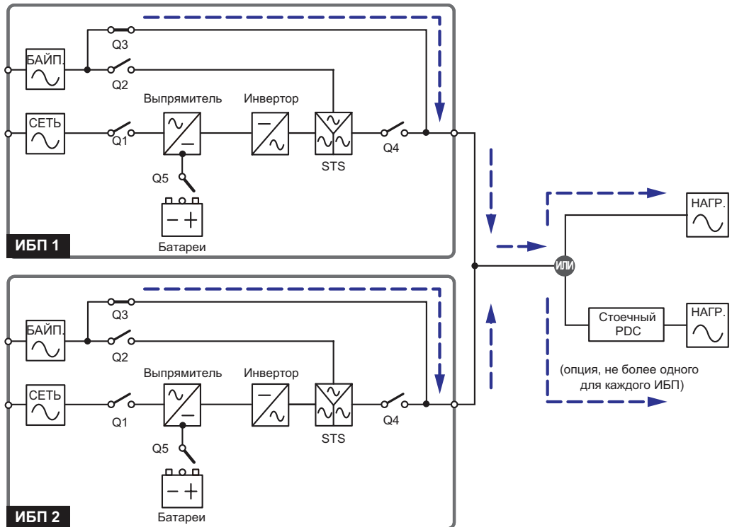
Рис. 3-9. Режим ручного байпаса (система с несколькими параллельными ИБП)
