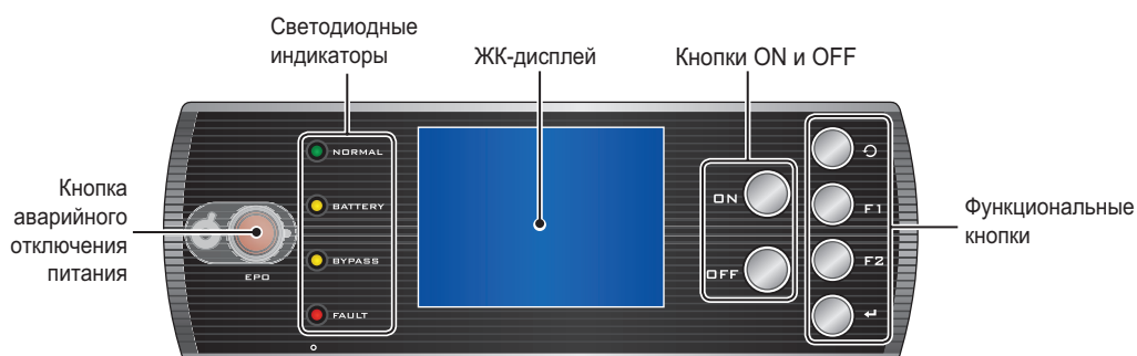
Рис. 7-2. Панель управления
