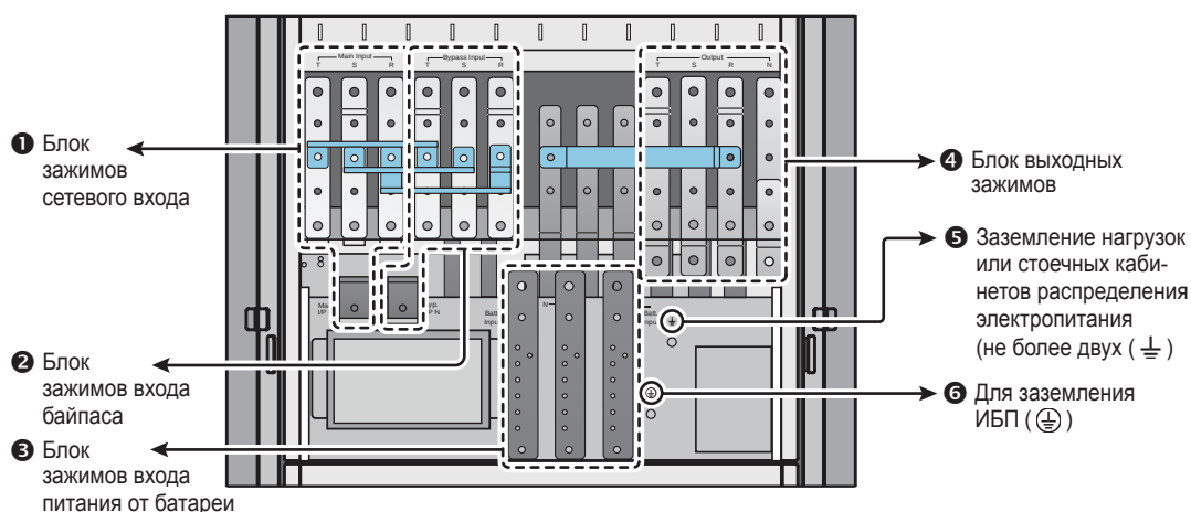
Рис. 5-6. Выводы ИБП
