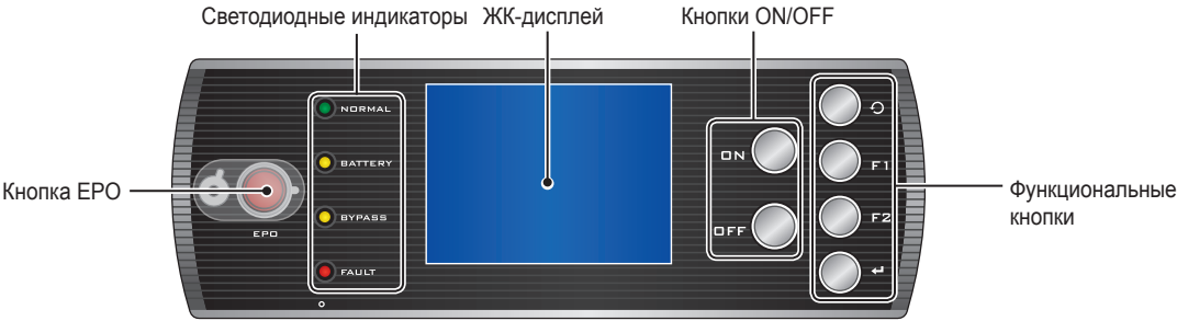
Рис. 2-8. Панель управления
