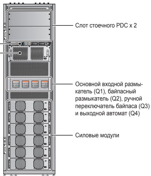
Рис. 2-5. Вид спереди с открытой дверцей
