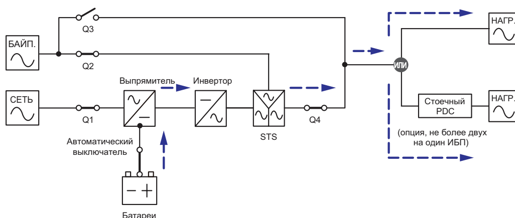
Рис. 3-2. Автономный режим работы, система с одним ИБП
