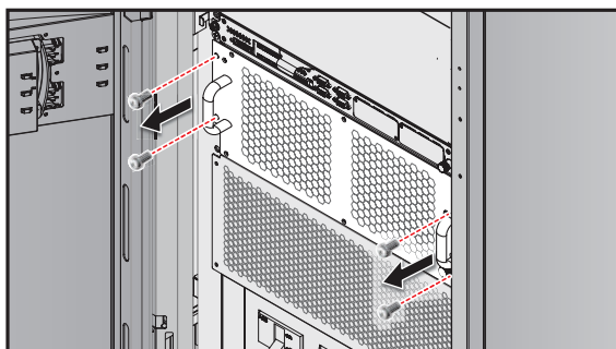
Рис. 5-28. Выкручивание винтов
