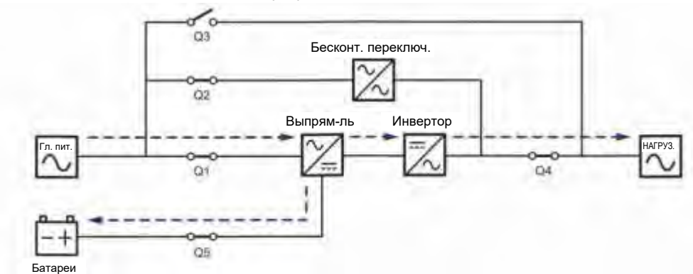
Рисунок 3-1: Схема режима двойного преобразования, подключение одного ИБП к одной линии
