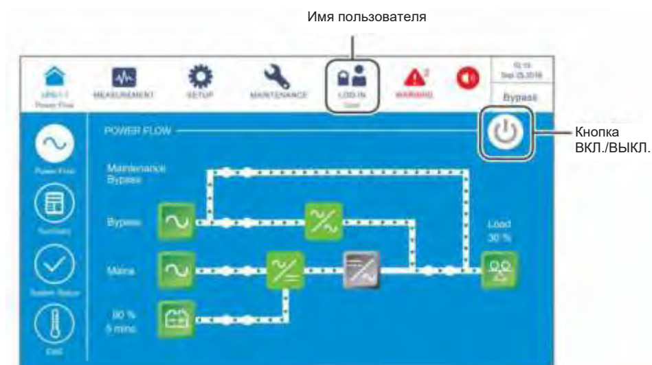
Рисунок 6-18: Экран режима байпаса: расположение кнопок имени пользователя и ВКЛ./ВЫКЛ.
