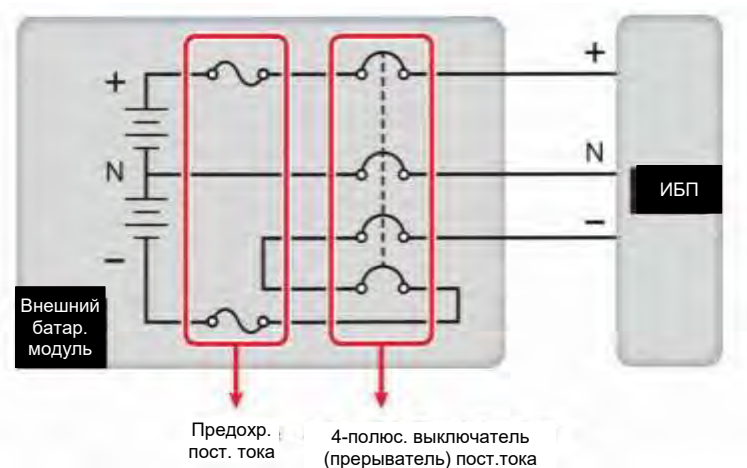
Рисунок 5-18: Установка 4-х полюсного автоматического выключателя или прерывателя постоянного тока с предохранителем
