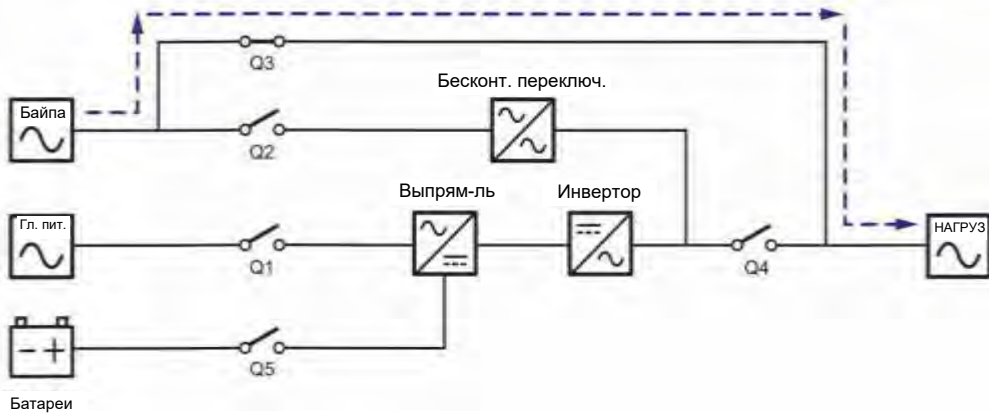
Рисунок 3-18: Схема ручного байпасного режима, подключение к двум линиям одного ИБП
