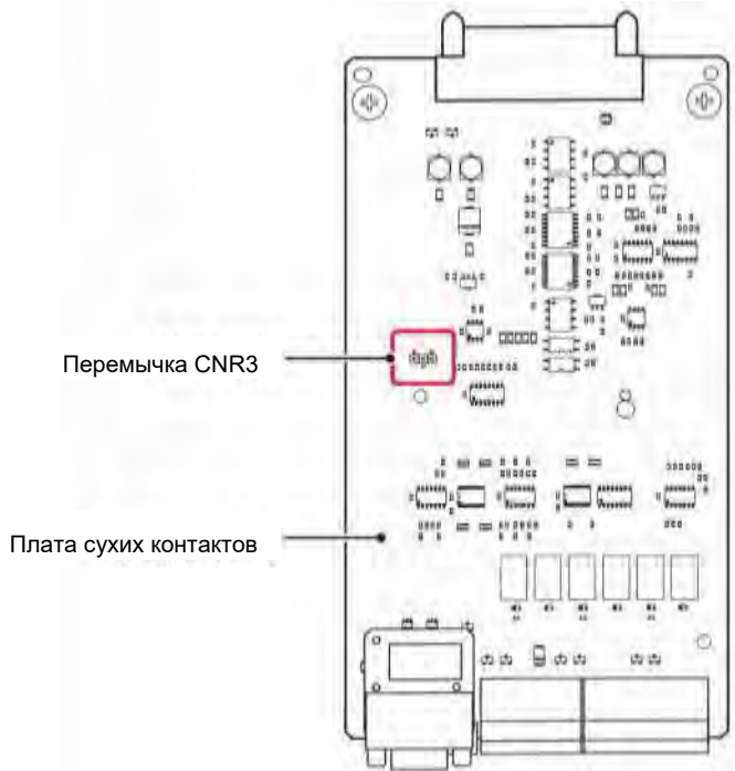
Рисунок 4-6: Расположение переключки CNR3
