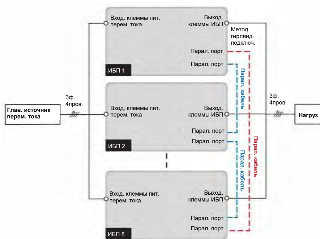
Рисунок 5-14: Схема подключения параллельных устройств к одной линии
