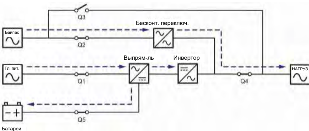
Рисунок 3-19: Схема ESO-режима, подключение одного ИБП к двум линиям питания
