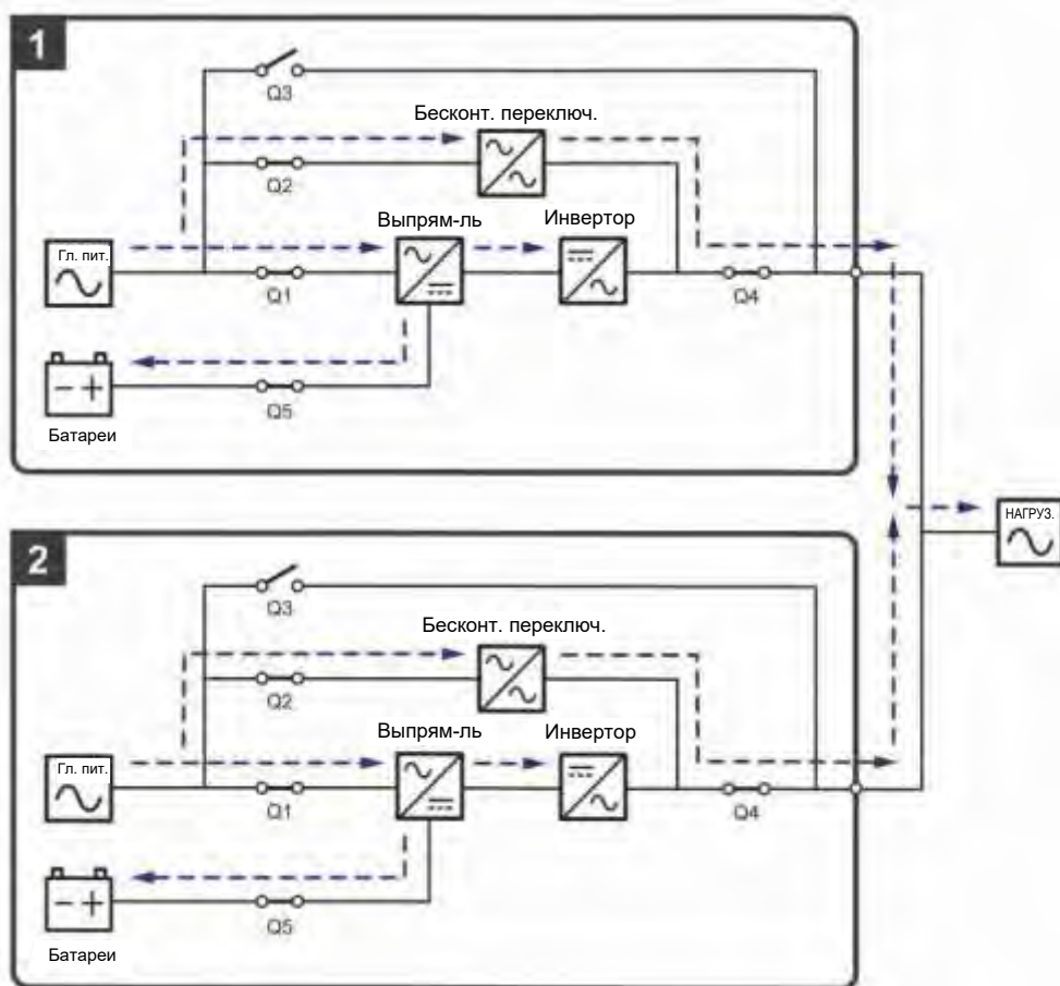
Рисунок 3-13: Схема ECO-режима, подключение к одной линии параллельных ИБП
