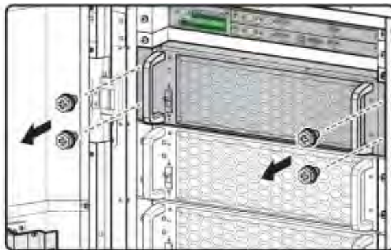
Рисунок 5-50: Снятие 4 винтов
