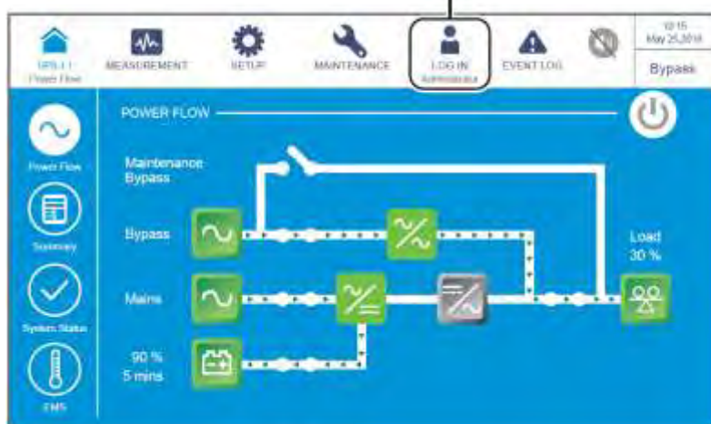
Рисунок 6-65: Экран байпасного режима и имя администратора
