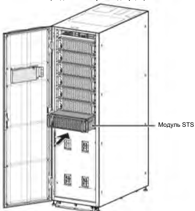
Рисунок 5-35: Установка STS-модуля в ИБП
