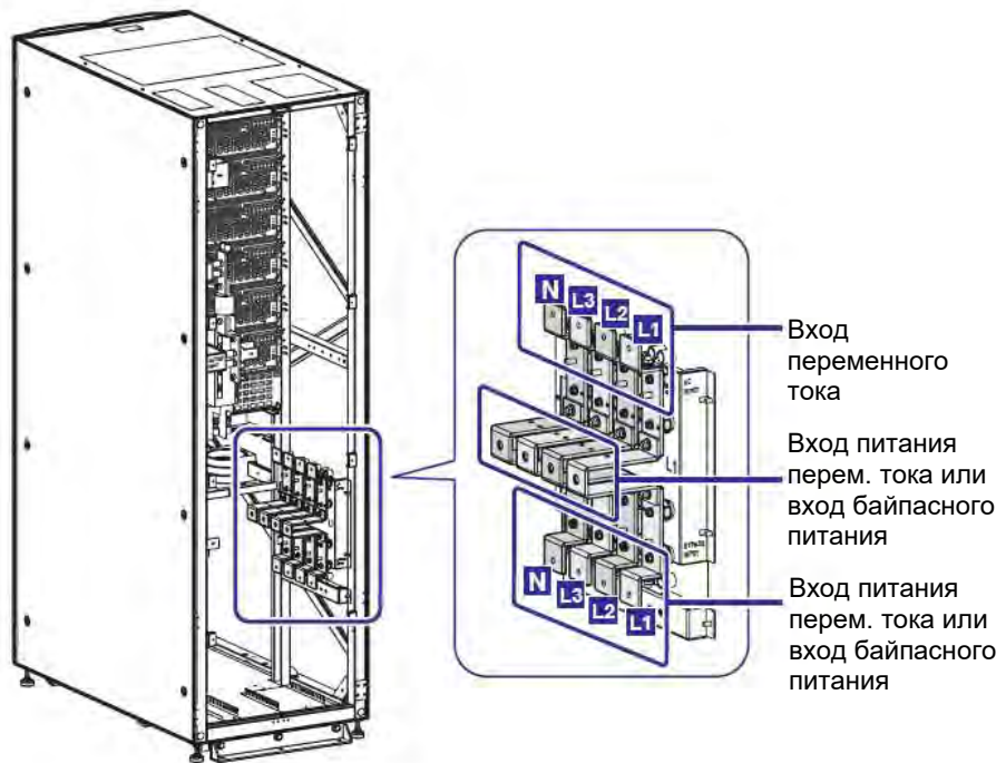
Рисунок 5-6: Клеммы: вход питания переменного тока и вход байпаса
