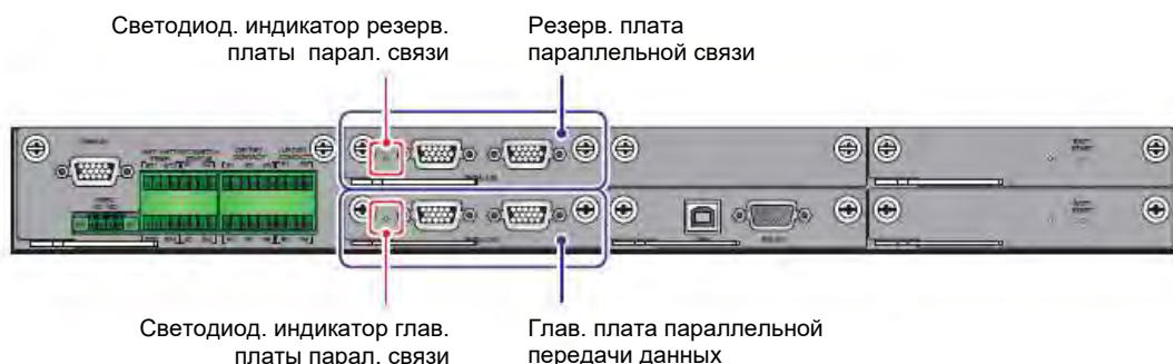
Рисунок 4-11: Расположение главной и резервной плат параллельной передачи данных и их светодиодных индикаторов
