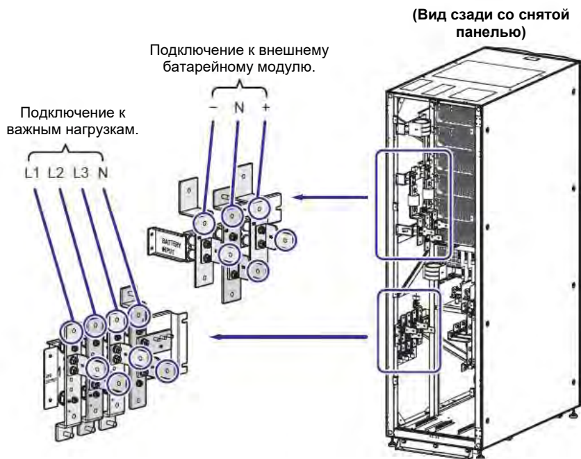
Рисунок 5-16: Схема верхнего подключения одного ИБП к одной линии. Шаг 2
