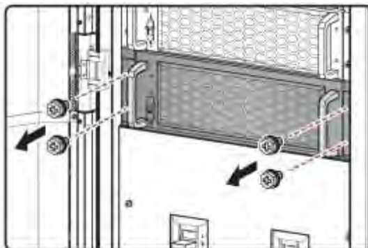
Рисунок 5-39: Снятие 4 винтов
