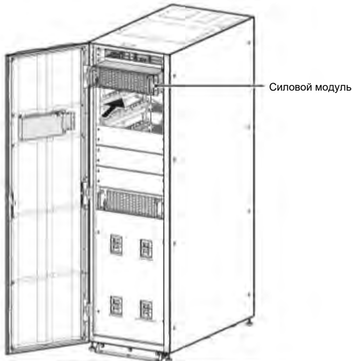
Рисунок 5-46: Установка силового модуля в ИБП
