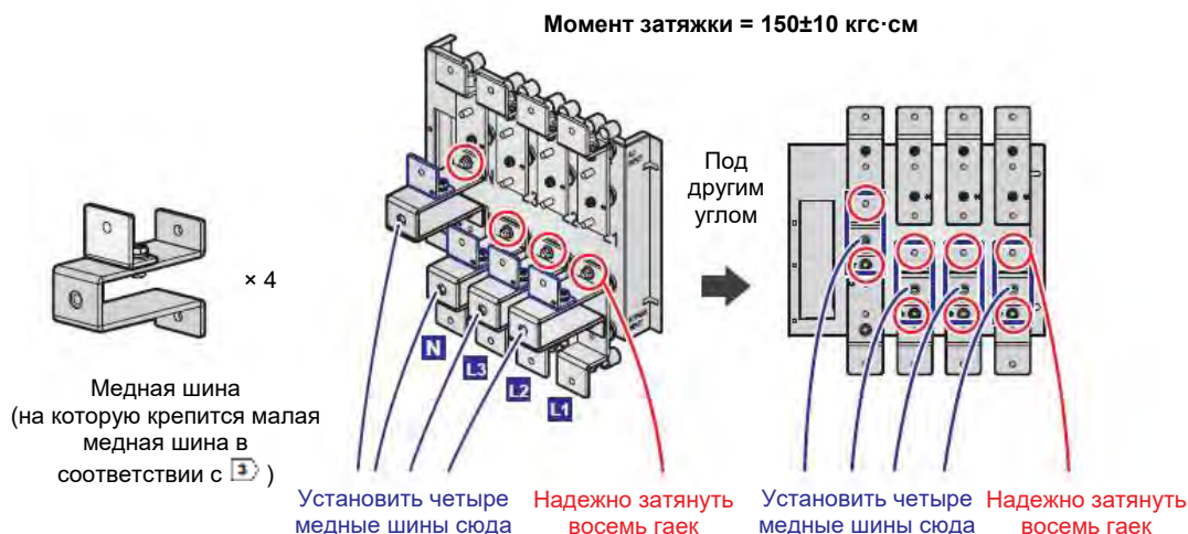
Рисунок 5-9: Установка четырех медных шин и восьми гаек при верхнем подключении к двум линиям питания
