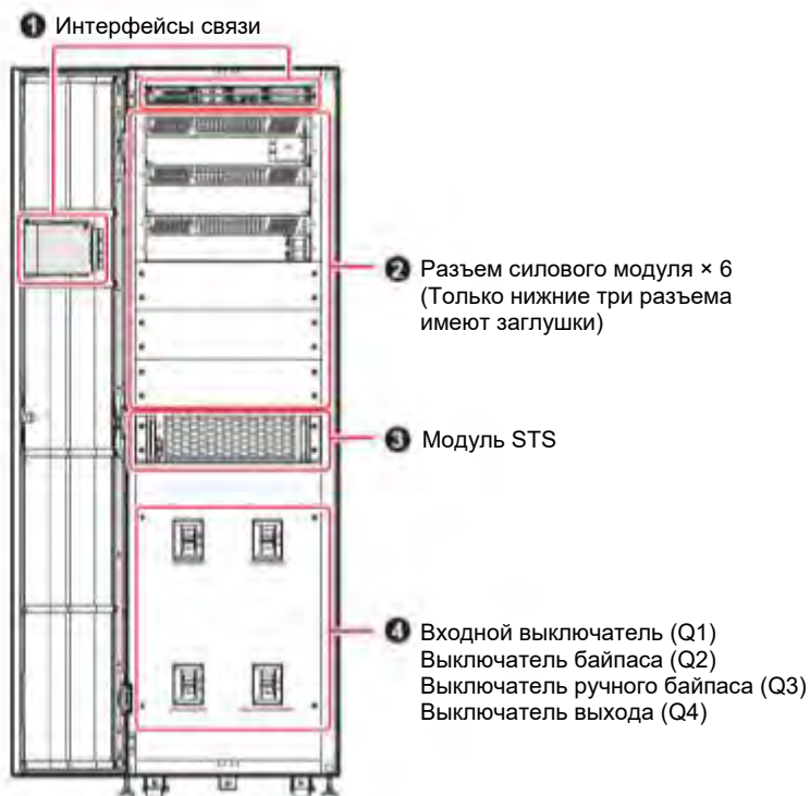
Рисунок 2-4: Вид ИБП изнутри (спереди с открытой дверцей)
