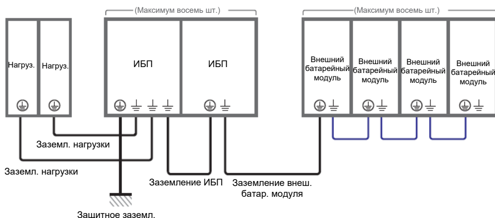
Рисунок 5-25: Схема заземления параллельных ИБП
