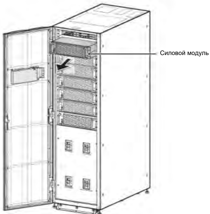
Рисунок 5-51: Демонтаж силового модуля
