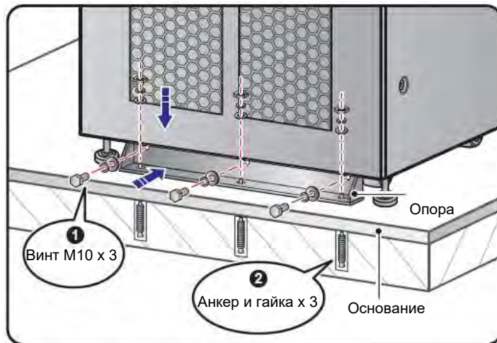
(Вид сзади)
