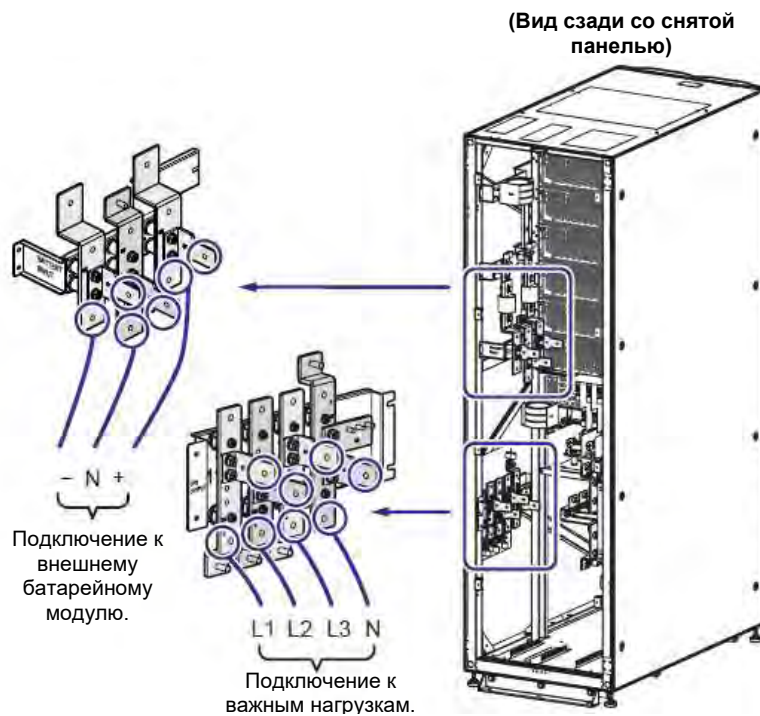
Рисунок 5-23: Схема нижнего подключения одного ИБП к двум линиям. Шаг 2
