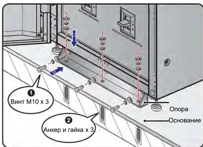
Рисунок 5-3: Установка передней выравнивающей опоры ИБП
