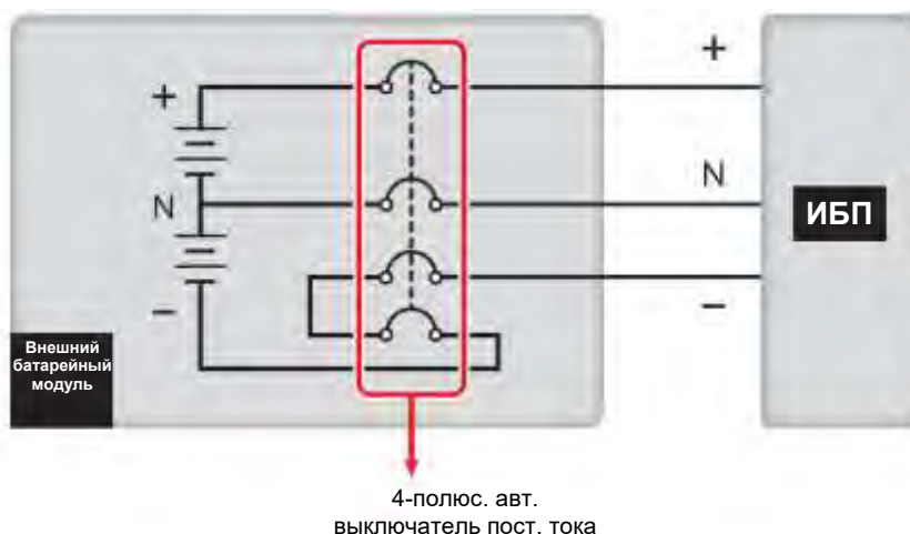
Рисунок 5-30: Установка 4-х полюсного выключателя постоянного тока
