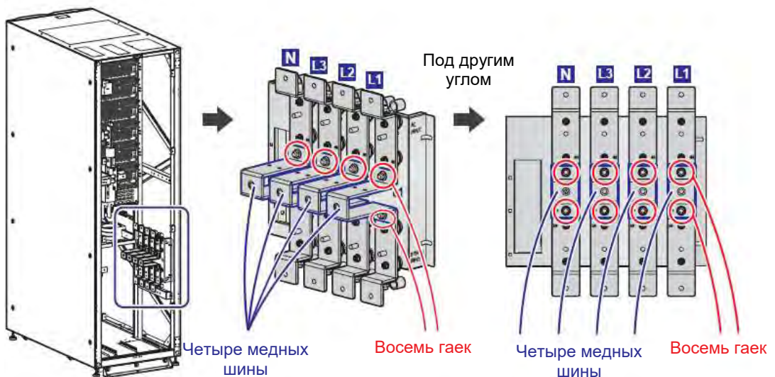
Рисунок 5-7: Снятие восьми гаек и четырех медных шин
