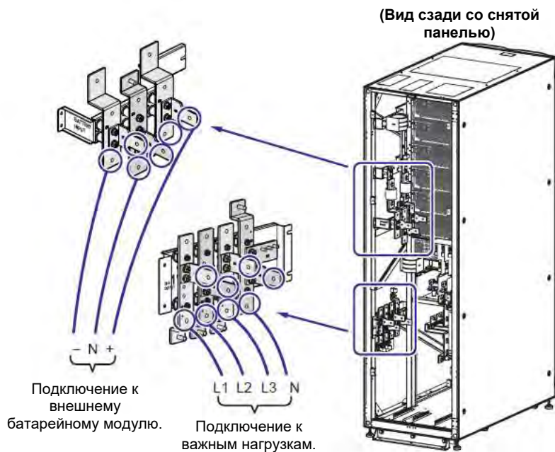
Рисунок 5-18: Схема нижнего подключения одного ИБП к одной линии. Шаг 2
