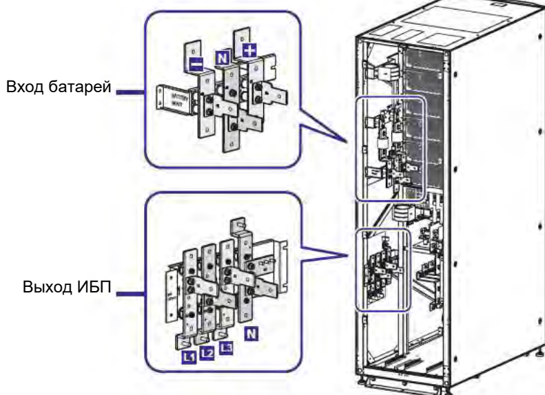
Рисунок 5-12: Клеммы: вход для подключения батарей и выход ИБП
