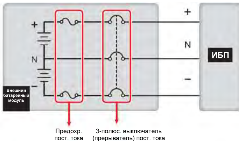
Рисунок 5-29: Установка 3-х полюсного автоматического выключателя или прерывателя постоянного тока с предохранителем
