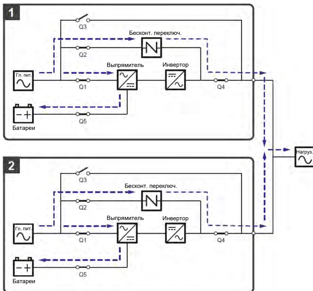
Рисунок 3-11: Схема байпасного режима, подключение к одной линии параллельных ИБП
