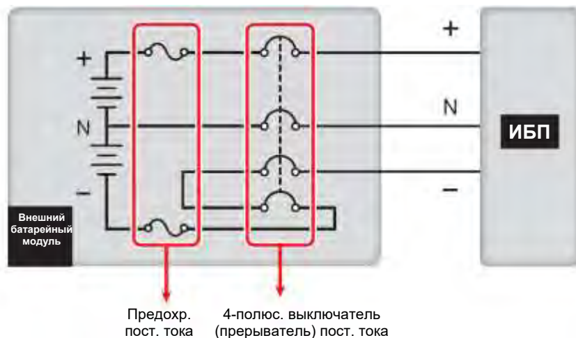
Рисунок 5-28: Установка 4-х полюсного автоматического выключателя или прерывателя постоянного тока с предохранителем
