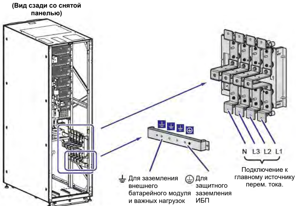
Рисунок 5-17: Схема нижнего подключения одного ИБП к одной линии. Шаг 1
