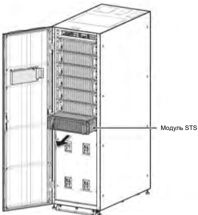
Рисунок 5-40: Демонтаж модуля STS
