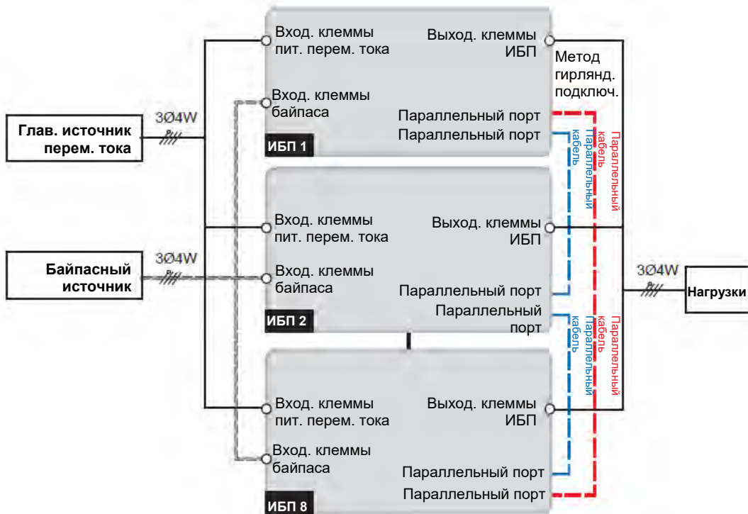
Рисунок 5-26: Схема подключения параллельных ИБП к двум линиям питания
