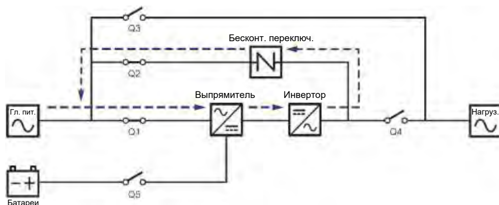
Рисунок 3-8: Схема режима повторного использования электроэнергии, подключение к одной линии одного ИБП
