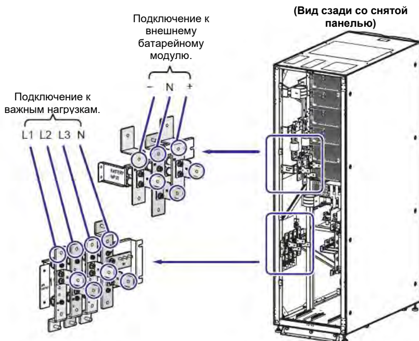
Рисунок 5-21: Схема верхнего подключения одного ИБП к двум линиям. Шаг 2
