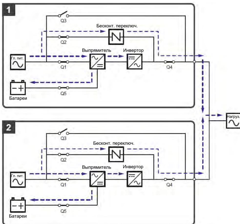
Рисунок 3-13: Схема ЭСО-режима, подключение к одной линии параллельных ИБП
