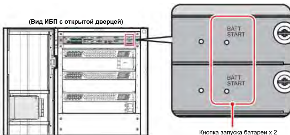
Рисунок 7-2: Расположение кнопок запуска батареи
