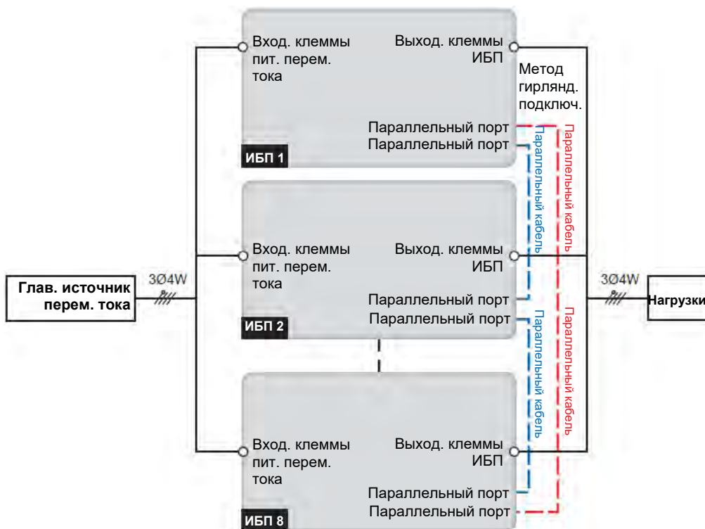
Рисунок 5-24: Схема подключения параллельных ИБП к одной линии
