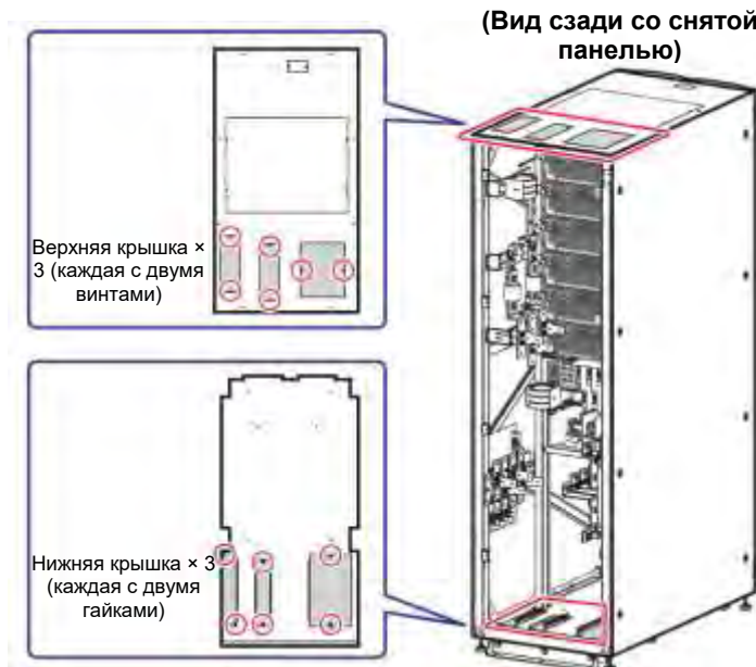
Рисунок 5-14: Расположение верхней и нижней панелей
