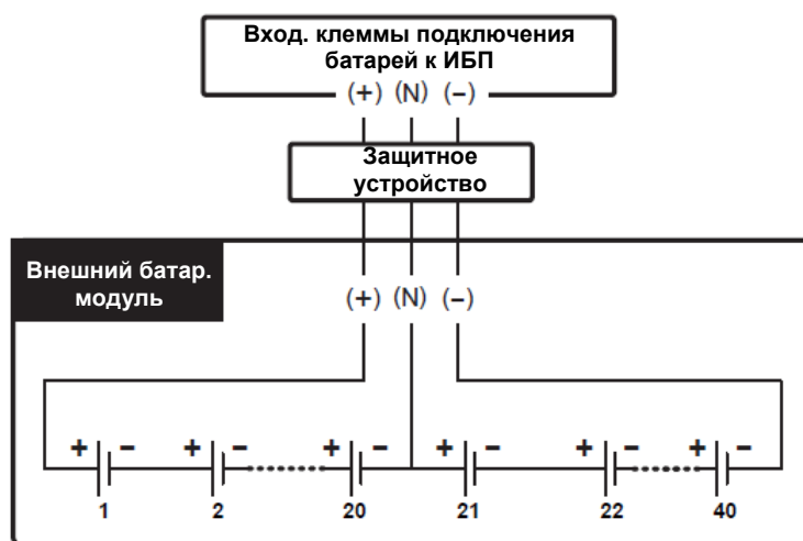
Рисунок 5-27: Подключение внешнего батарейного модуля
