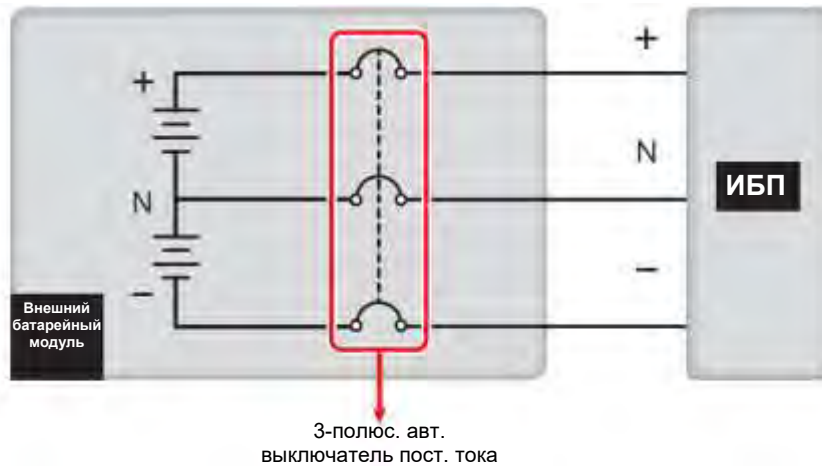
Рисунок 5-31: Установка 3-х полюсного выключателя постоянного тока
