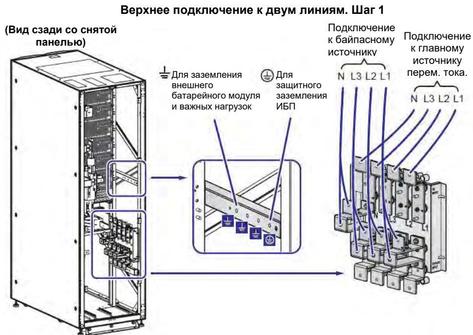
Рисунок 5-20: Схема верхнего подключения одного ИБП к двум линиям. Шаг 1
