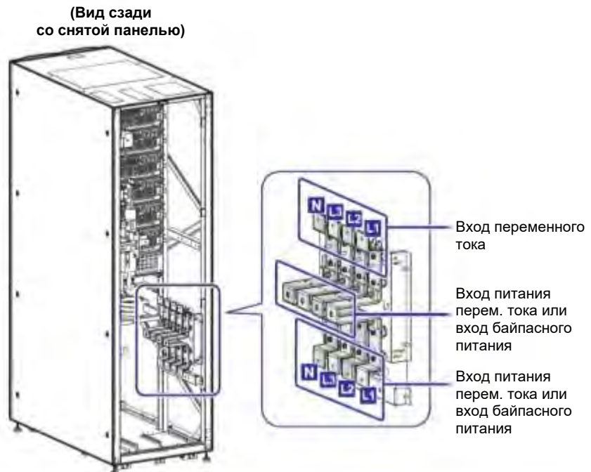
Рисунок 2-8: Клеммы: вход питания переменного тока и вход байпаса
