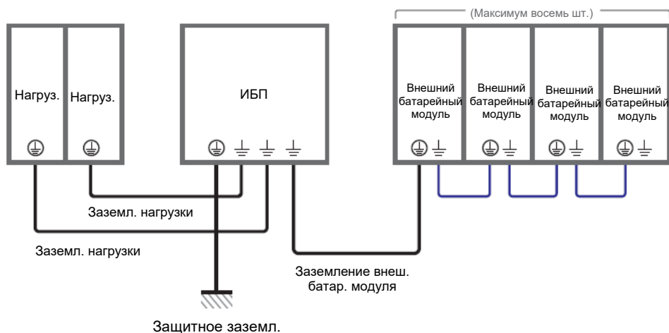
Рисунок 5-19: Схема заземления, один ИБП
