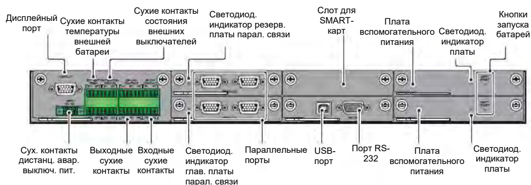
Рисунок 4-3: Функции интерфейсов связи
