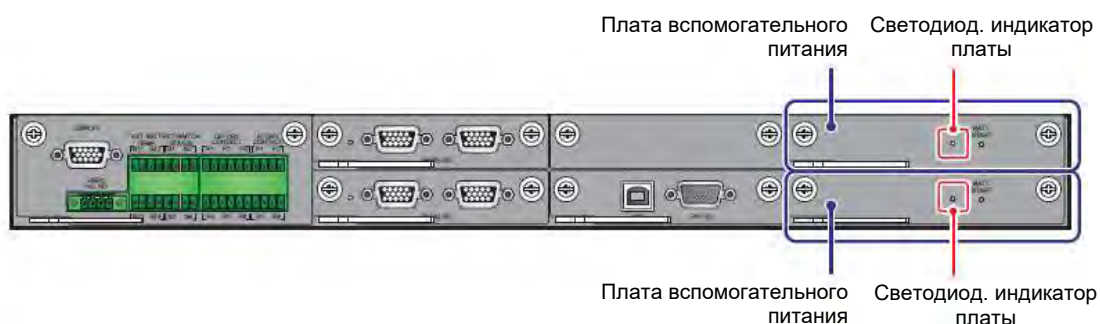
Рисунок 4-15: Расположение плат вспомогательного питания и их светодиодных индикаторов
