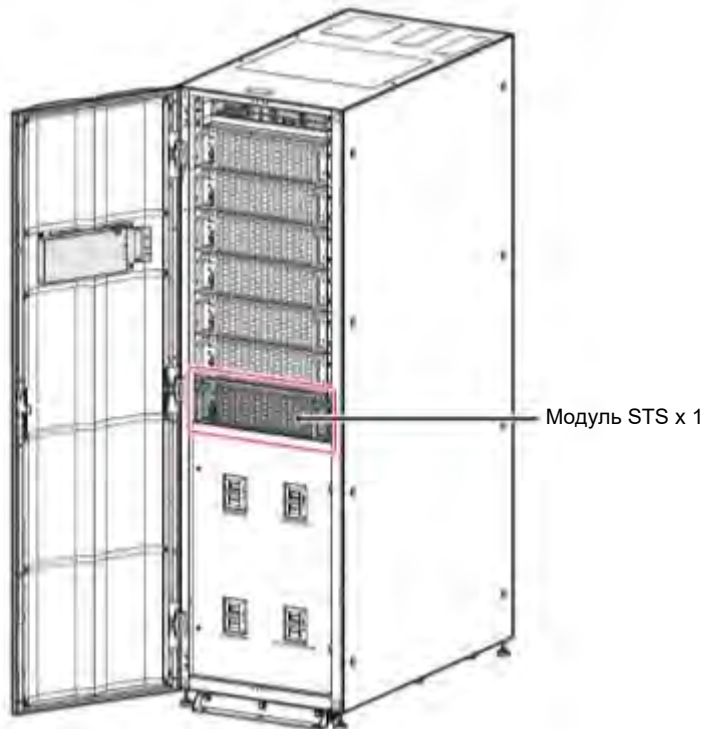
Рисунок 5-32: Расположение STS-модуля
