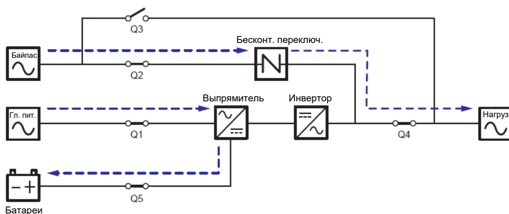
Рисунок 3-17: Схема байпасного режима, подключение одного ИБП к двум линиям питания
