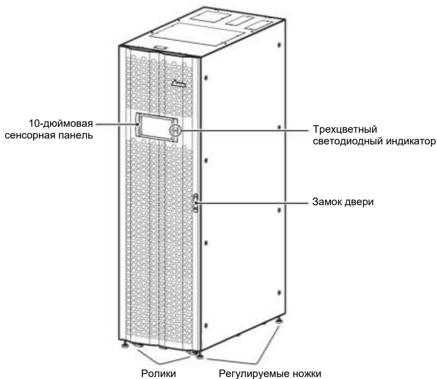
Рисунок 2-2: Вид ИБП спереди
