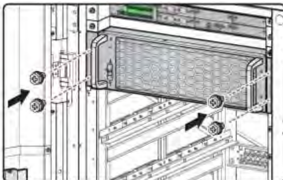
Рисунок 5-47: Крепление силового модуля в ИБП
