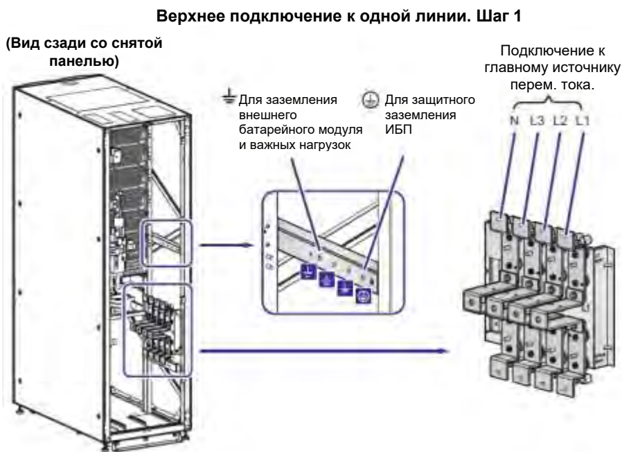
Рисунок 5-15: Схема верхнего подключения одного ИБП к одной линии. Шаг 1
