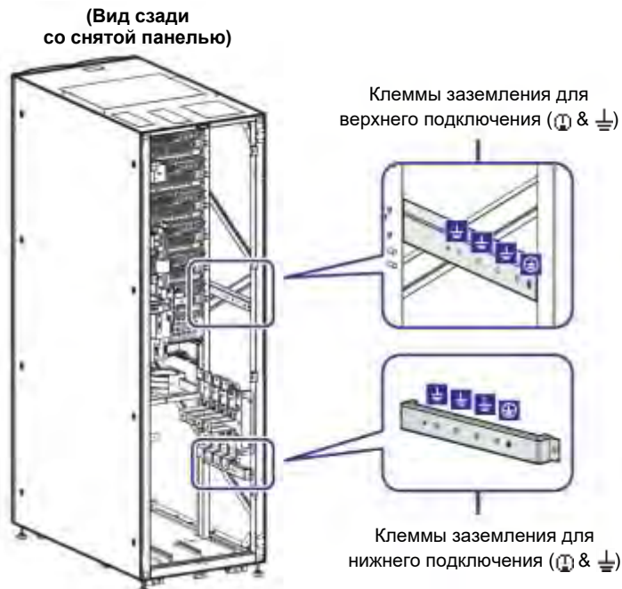
Рисунок 2-10: Клеммы заземления
