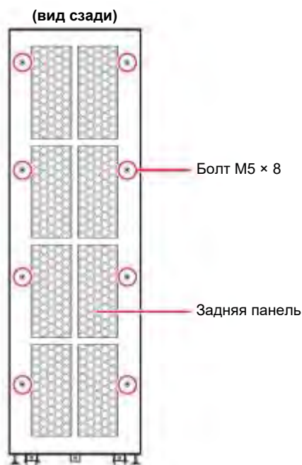
Рисунок 2-7: Расположение задней панели и винтов
