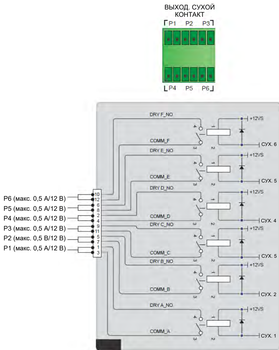
Рисунок 4-9: Схема выходных сухих контактов
