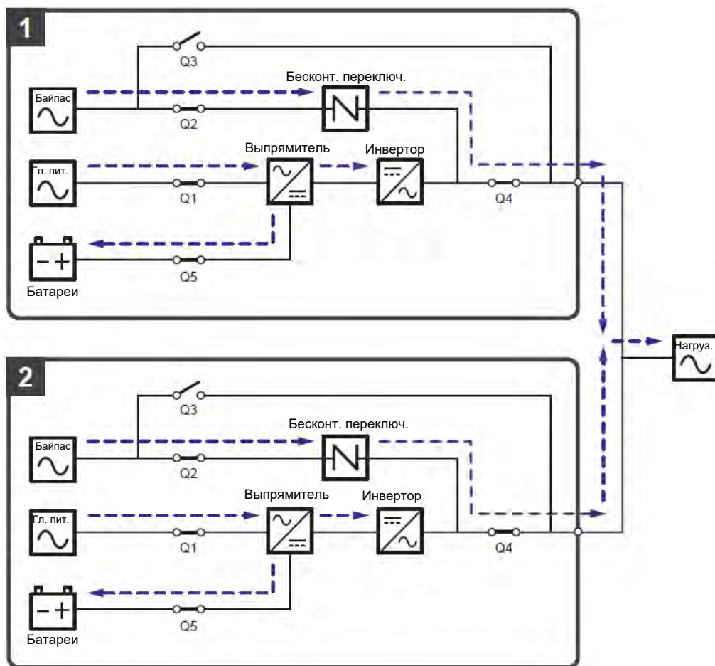
Рисунок 3-26: Схема ЕСО-режима, подключение к двум линиям, параллельных ИБП
