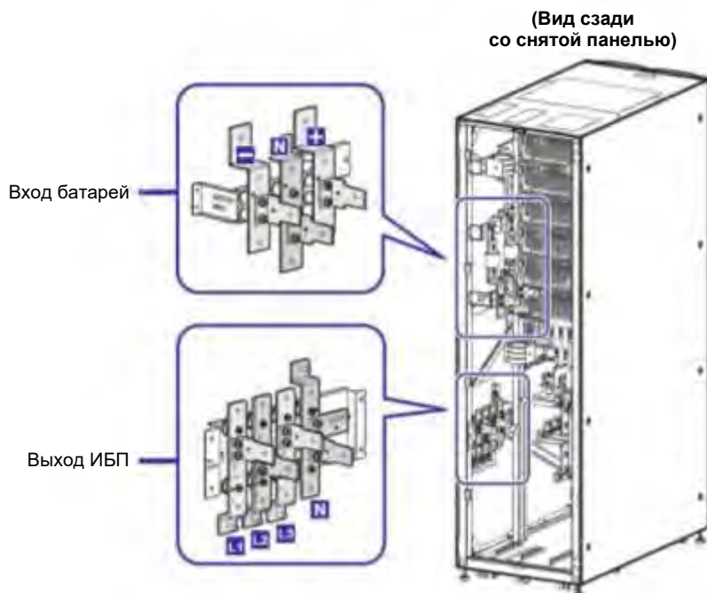
Рисунок 2-9: Клеммы: вход для подключения батарей и выход ИБП
