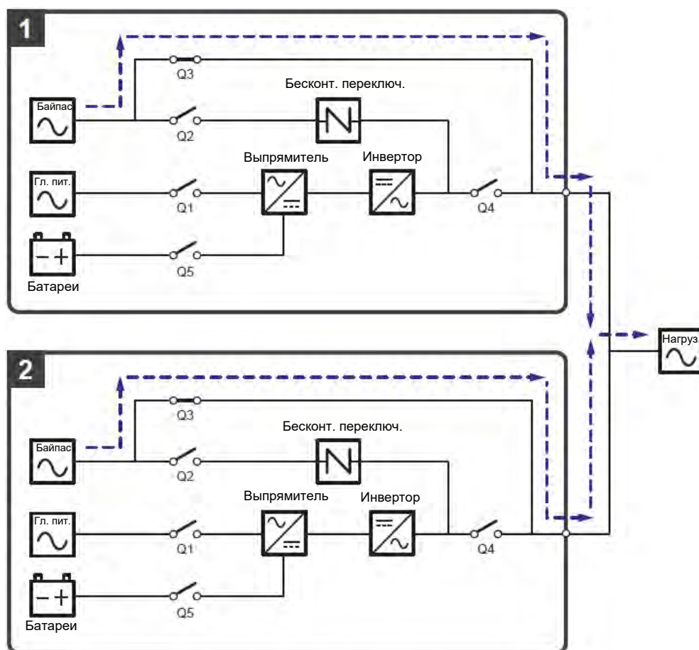
Рисунок 3-25: Схема ручного байпасного режима, подключение к двум линиям параллельных ИБП
