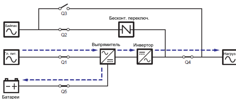
Рисунок 3-21: Схема энергосберегающего режима, подключение одного ИБП к двум линиям питания
