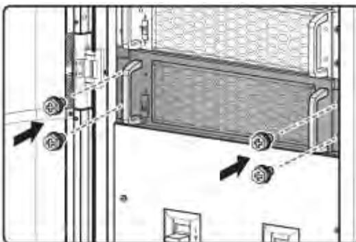
Рисунок 5-36: Крепление STS-модуля в ИБП
