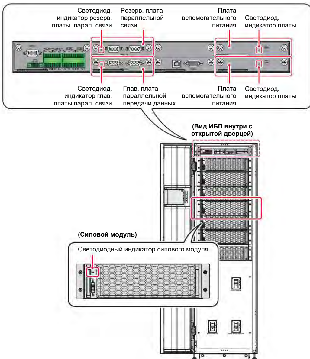
Рисунок 6-1: Расположение плат параллельной связи, вспомогательного питания, силовых модулей и соответствующих светодиодных индикаторов
