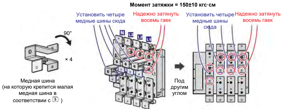
Рисунок 5-10: Установка четырех медных шин и восьми гаек при нижнем подключении к двум линиям питания
