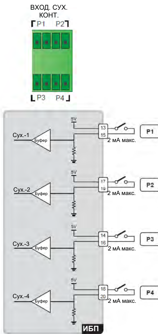
Рисунок 4-10: Схема входных сухих контактов
