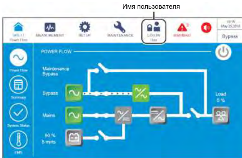
Рисунок 6-40: Главный экран и имя пользователя
