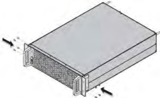
Рисунок 5-45: Установка двух кронштейнов
