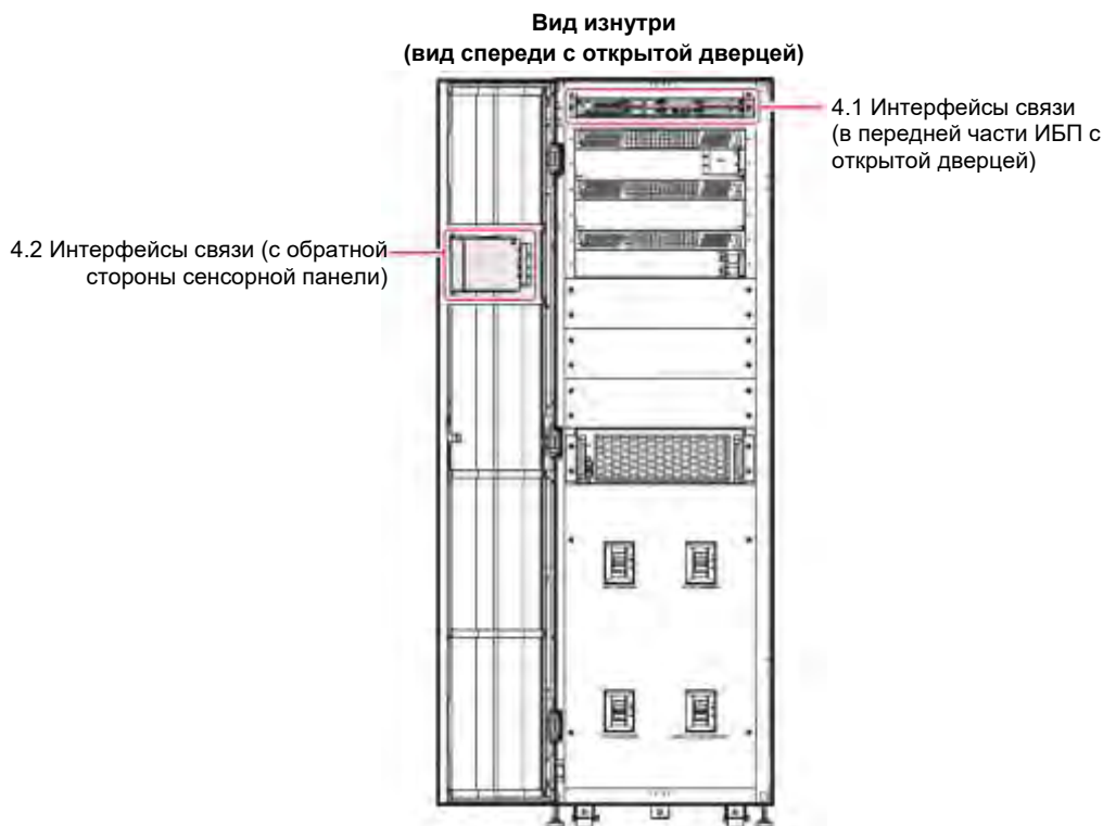
Рисунок 4-1: Расположение интерфейсов связи
