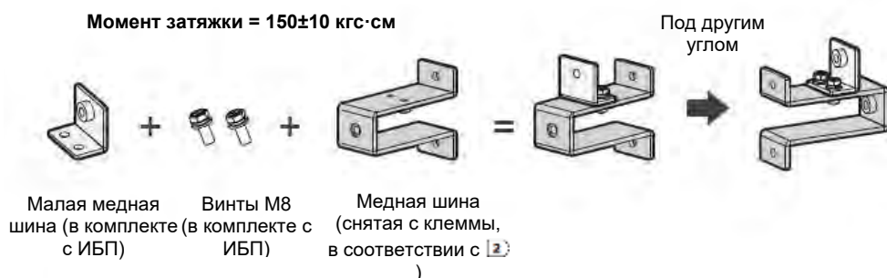
Рисунок 5-8: Крепление малой медной шины на снятую медную шину)
