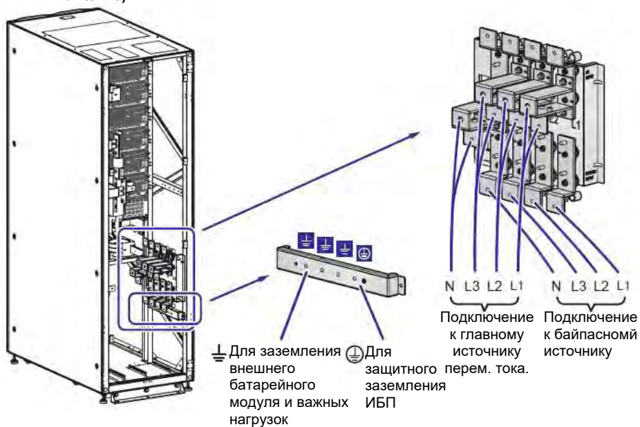
Рисунок 5-22: Схема нижнего подключения одного ИБП к двум линиям. Шаг 1
