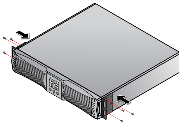
Рис. 3-1. Прикрепите монтажные уголки
