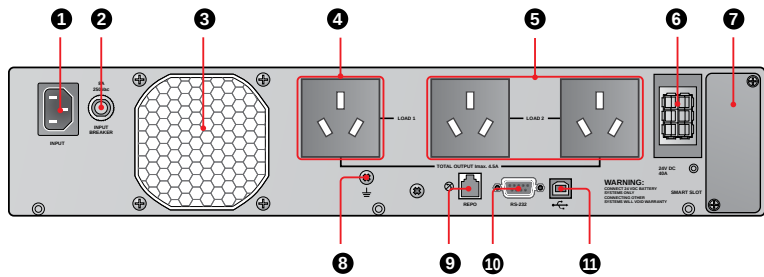
Задняя панель: UPS102R2RT0B0B2
