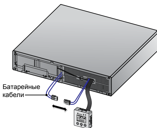
Рис. 8-4. Разъедините фиксатор разъёма и отсоедините батарейные кабели
