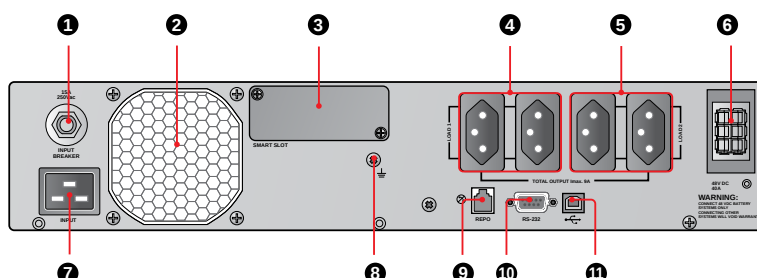
Задняя панель: UPS202R2RT0B0B1
