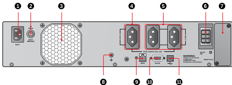
Задняя панель: UPS102R2RT0B0B1
