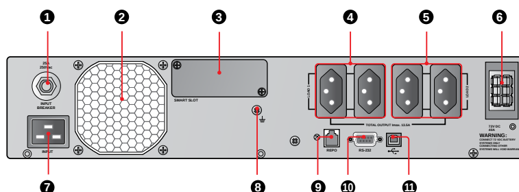
Задняя панель: UPS302R2RT0B0B1
