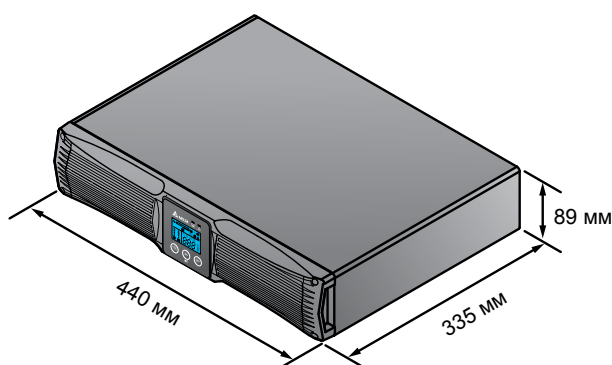
Рис. 2-1. Модель 1 кВА, внешний вид и размеры
