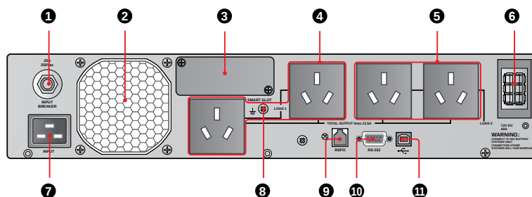
Задняя панель: UPS302R2RT0B0B2
