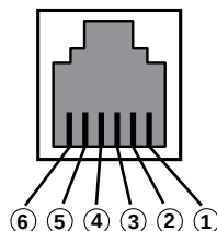
Рис. 7-2. Порт REPO (аварийное дистанционное отключение питания)
