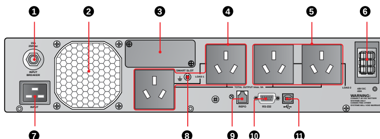
Задняя панель: UPS202R2RT0B0B2
