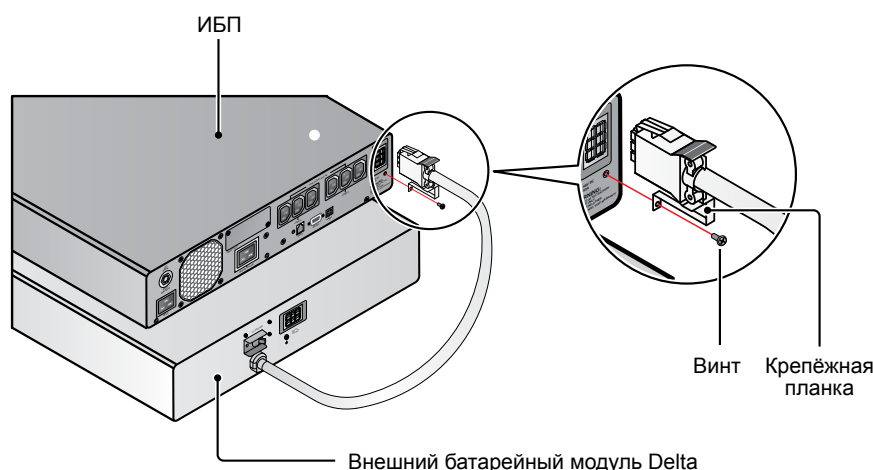
Рис. 4-2. Подключение внешнего батарейного модуля к ИБП
