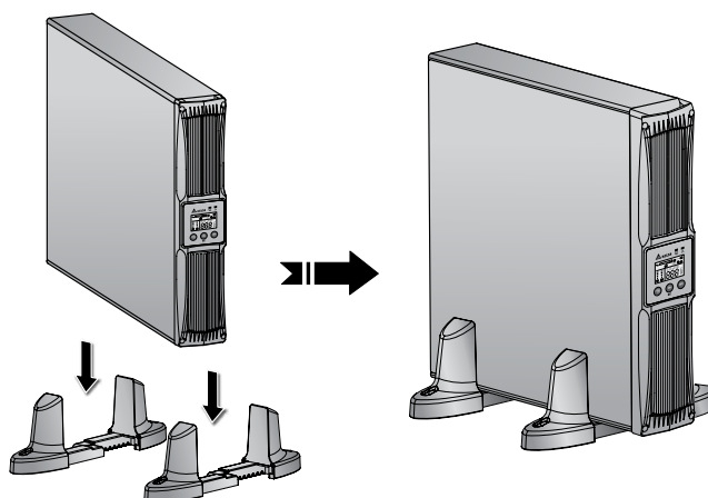
Рис. 3-10. Установите ИБП в опоры для вертикального монтажа
