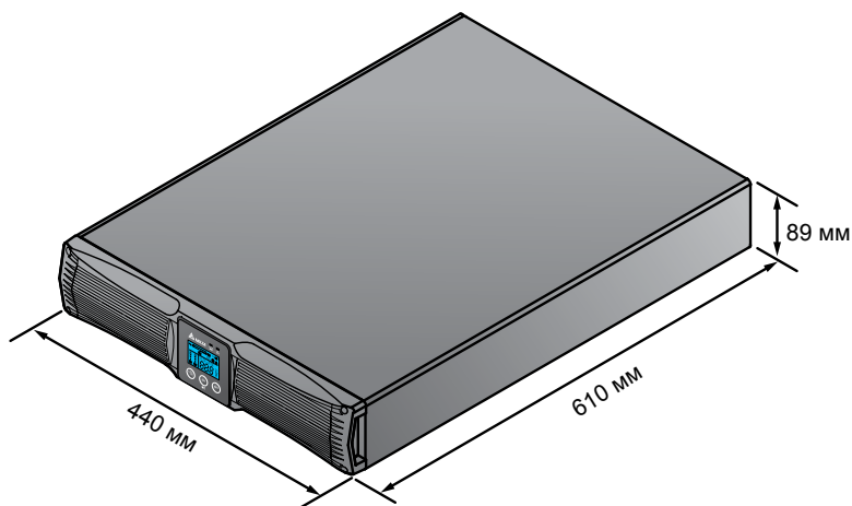
Рис. 2-3. Модель 3 кВА, внешний вид и размеры
