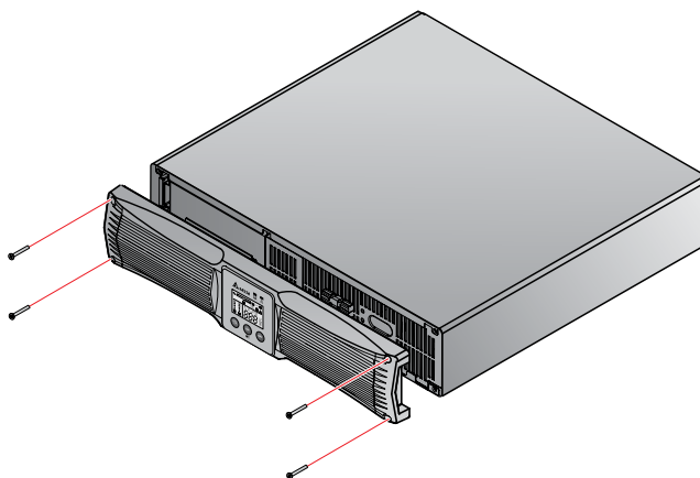
Рис. 8-1. Снимите пластмассовую переднюю панель
