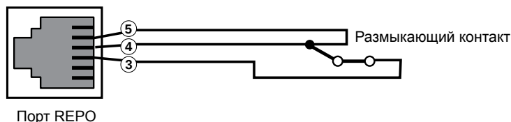
Рис. 7-3. Подключение порта REPO к выключателю с размыкающим контактом
