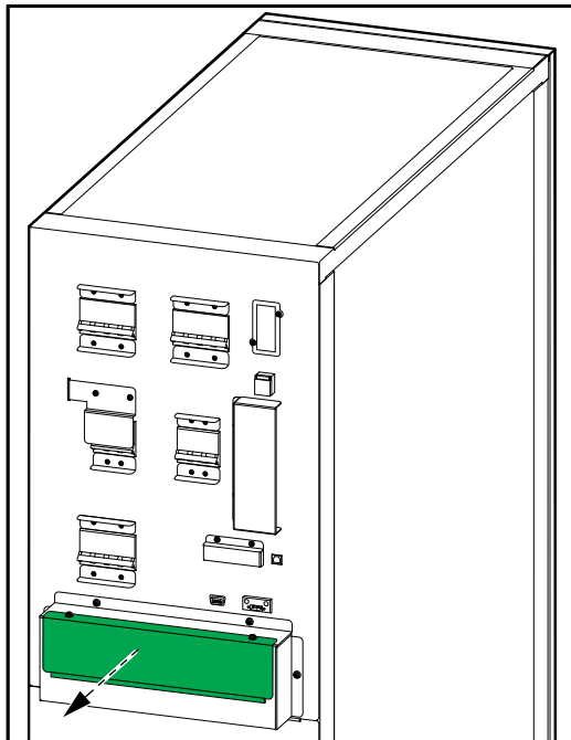
ИБП мощностью 20 кВА, вид сзади
