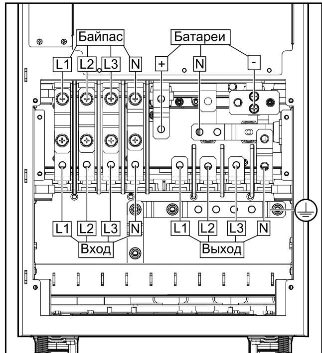
ИБП мощностью 100 кВА, вид сзади
