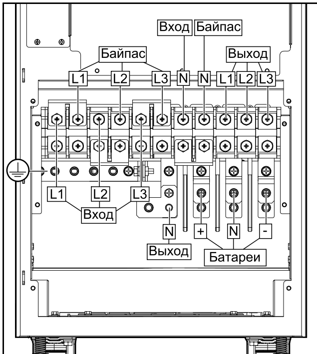
ИБП мощностью 60–80 кВА, вид сзади
