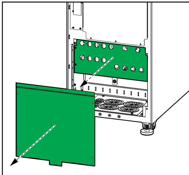
ИБП мощностью 100 кВА, вид сзади
