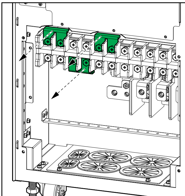
ИБП мощностью 60–80 кВА, вид сзади
