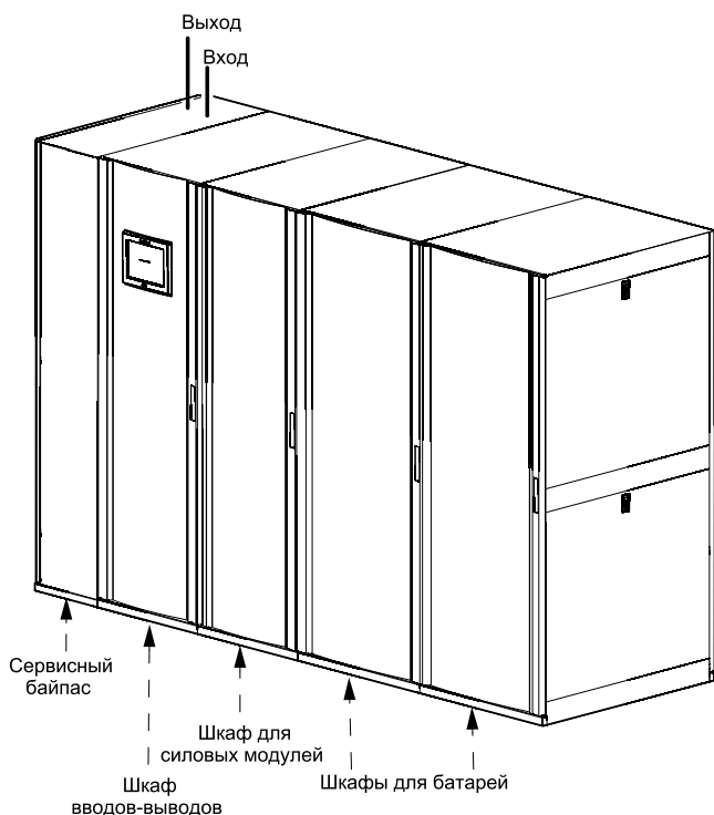
Верхний кабельный ввод с расположенными в ряд шкафами для аккумуляторных батарей
