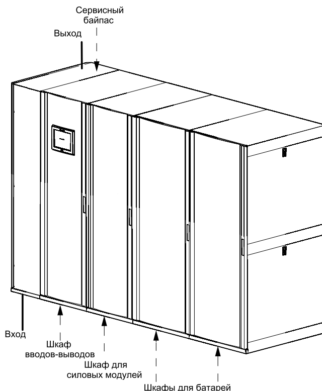
Нижний кабельный ввод с расположенными в ряд шкафами для аккумуляторных батарей
