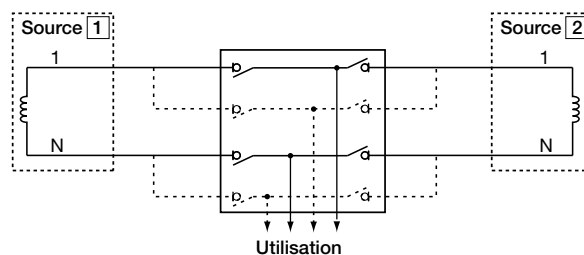
7.1.1.-4 Réseau monophasé avec neutre (phase-neutre) - 1BL*
