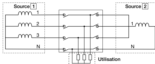
7.1.1.-6 Réseau triphasé avec neutre côté source [1] réseau monophasé avec neutre côté source [2] 41 NBL
