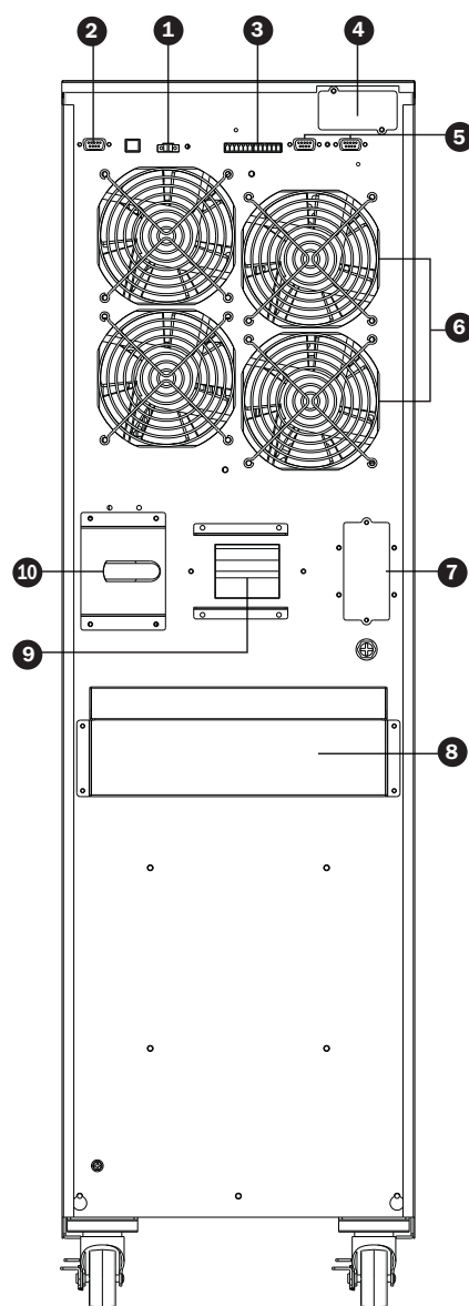
Схема 3. Задняя панель мод. SVT30KX
