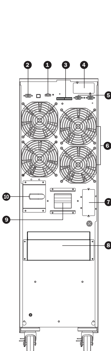
Схема 2. Задняя панель мод. SVT20KX
