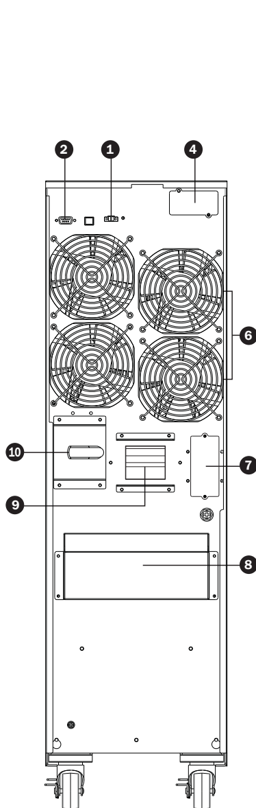
Схема 1. Задняя панель мод. SVT10KX
