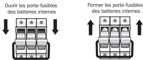
(Figure 4-4 : Ouvrir/Fermer les porte-fusibles des batteries internes)
