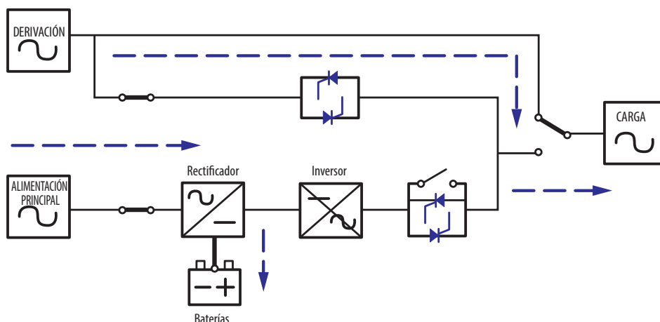
(Figura 5-5: Ruta de la Energía Eléctrica a través del UPS en Modo de Derivación Manual)
