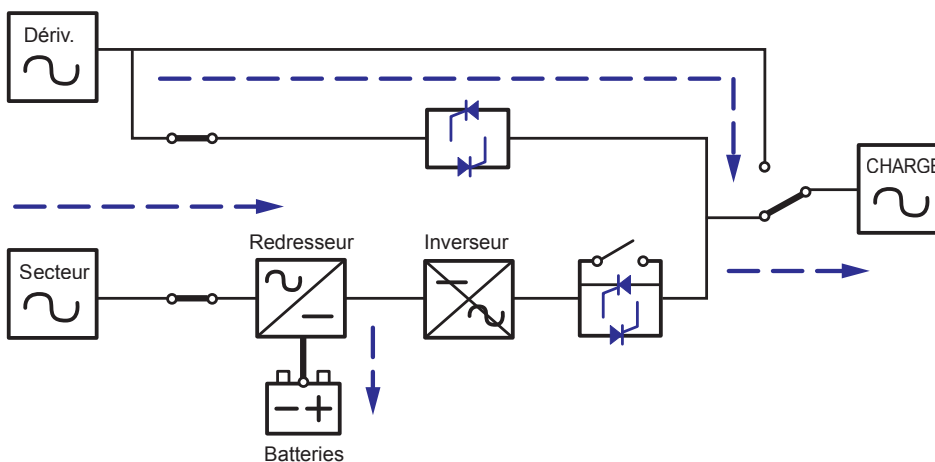
(Figure 5-5 : Trajet de l'énergie électrique dans l'onduleur en mode Dérivation)
