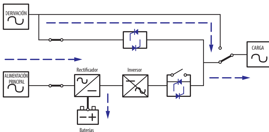
(Figura 5-5: Ruta de la Energía Eléctrica a través del UPS en Modo de Derivación)
