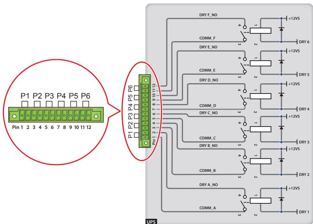
(Рис. 6-4. Выходной разъем с сухими контактами: распиновка и конструкция)
