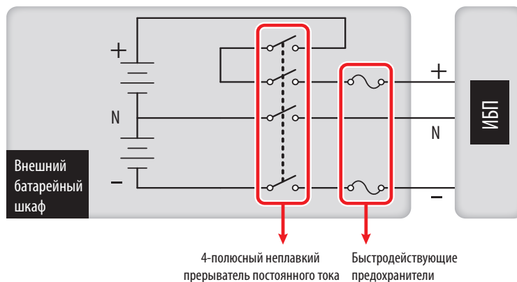
(Рис. 3-17. Установка 4-полюсного нелавкого прерывателя постоянного тока и быстродействующих плавких предохранителей (вариант I))
