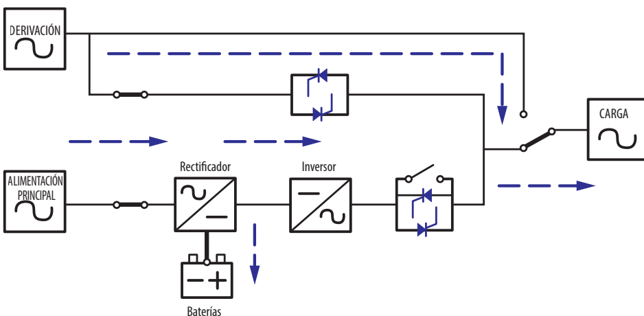
(Figura 5-3: Ruta de la Energía Eléctrica a través del UPS en Modo ECO)
