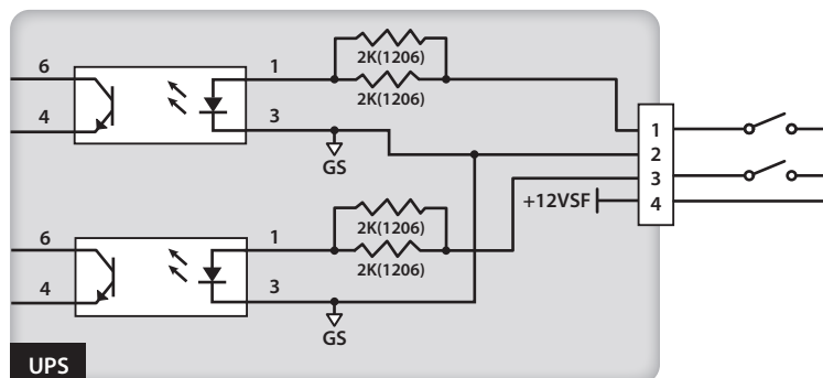
(Figure 6-6 : Configuration I du contact sec d'entrée)
