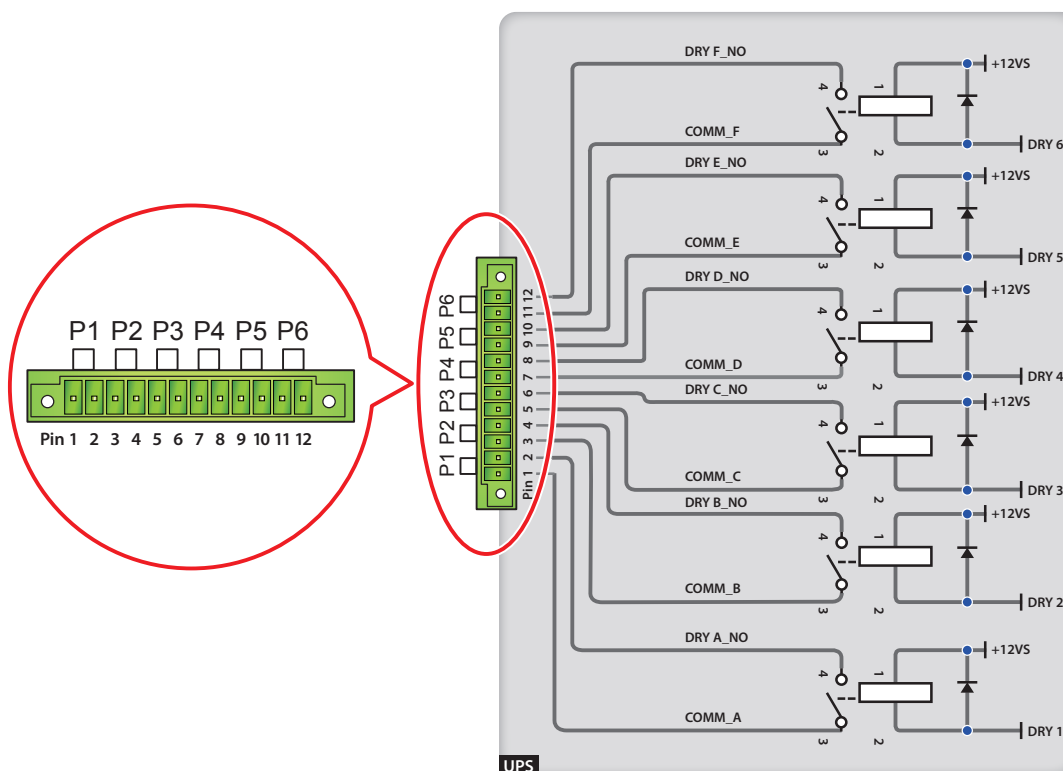
(Figura 6-4: Contactos Secos de Salida: definición de Pin y Diseño)
