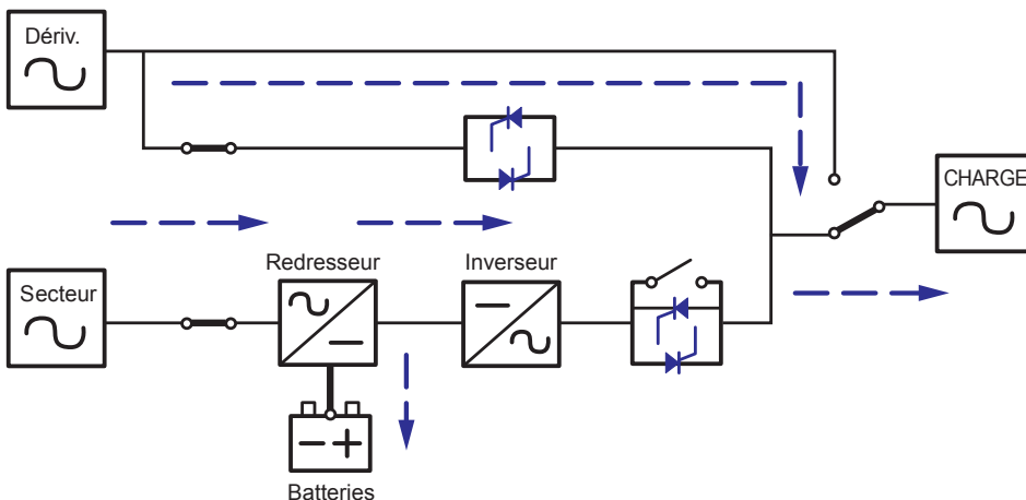
(Figure 5-3 : Trajet de l'énergie électrique dans l'onduleur en mode ECO)
