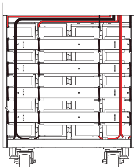
(Figura 3-6: instalación de la Batería)
