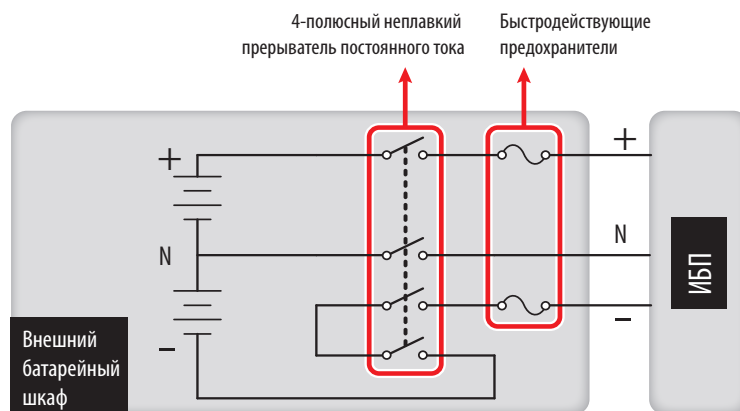
(Рис. 3-18. Установка 4-полюсного нелавкого прерывателя постоянного тока и быстродействующих плавких предохранителей (вариант II))
