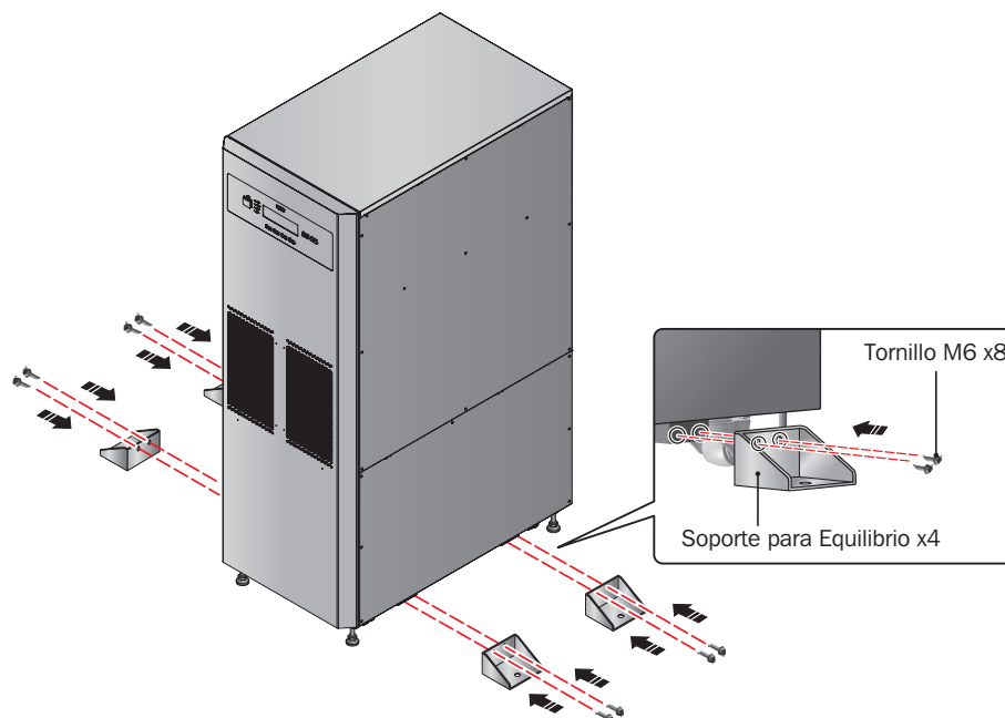
de(Figura 3-3: Instalación de los Soporte de Balance)
