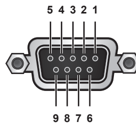
(Figura 6-3: Puerto RS-232)
