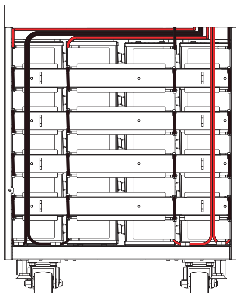
(Figure 3-6 : Installation de la batterie)
