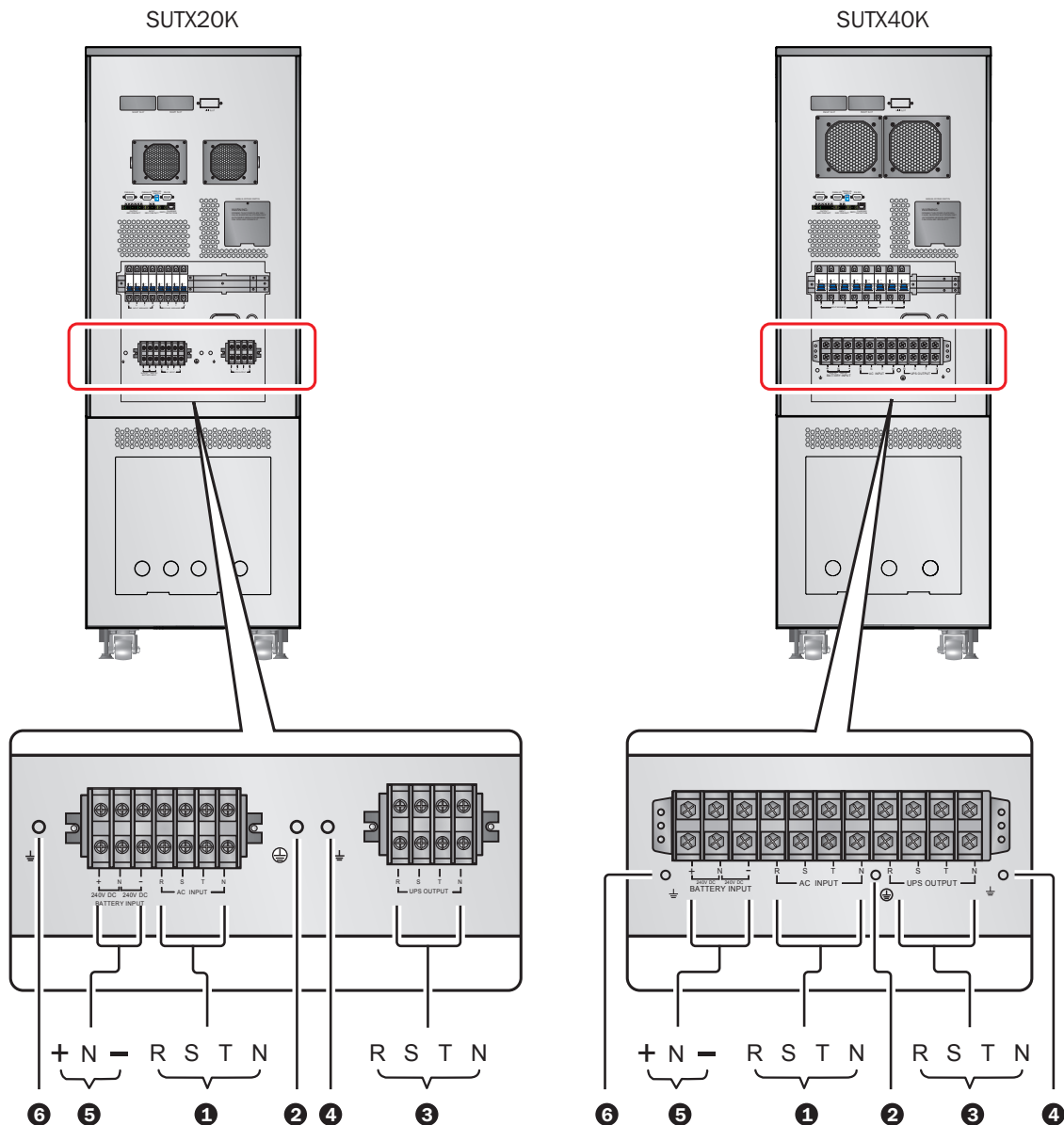
(Figura 3-5: Bloque de Terminales de Cableado)
