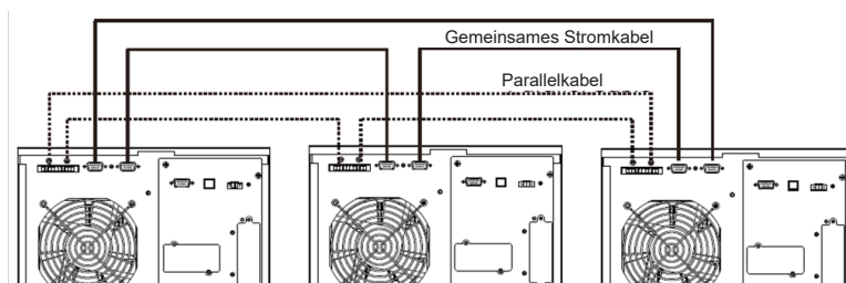
USV-Verkabelung Parallelsystem S3M60KX und S3M80KX
