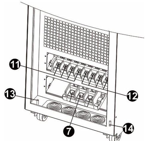
Vorderansicht S3M80KX bei geöffneter Tür Eingangs- und Ausgangsanschlüsse S3M60KX und S3M80KX
