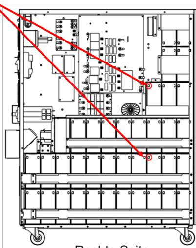
Rechte Seite S3M30KX/S3M40KX
