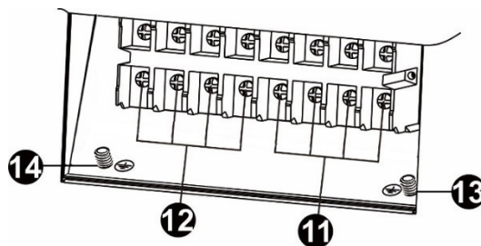
Bornes d'entrée/de sortie S3M30KX et S3M40KX
