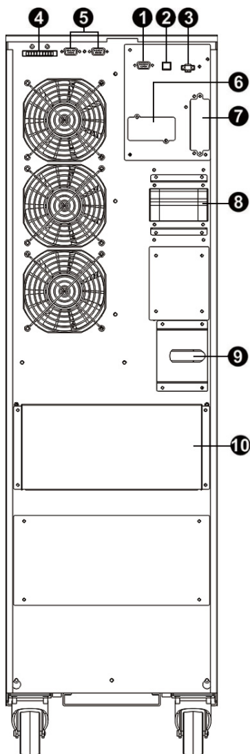
Panel Posterior del S3M30KX
