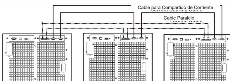
Cableado en Paralelo de Sistema UPS S3M60KX y S3M80KX
