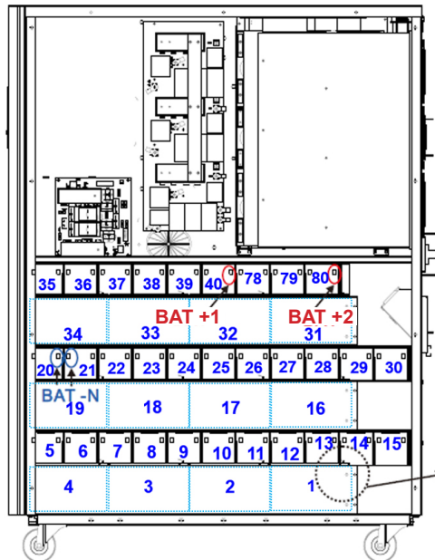
Left Side S3M30KX/S3M40KX
