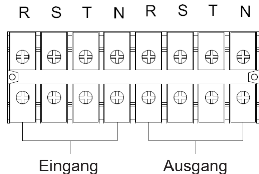
Verkabelungsdiagramm des Klemmenblocks für S3M30KX und S3M40KX Verkabelungsdiagramm des Klemmenblocks für S3M60K und S3M80K
