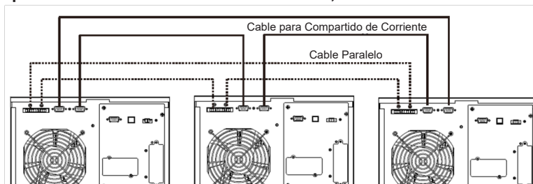
Cableado de UPS para Sistema en Paralelo UPS S3M30KX, S3M40KX S3M30KX/NIB y S3M40KX/NIB
