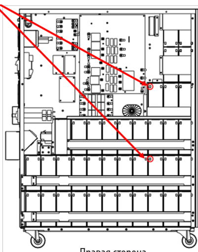
Правая сторона S3M30KX/S3M40KX
