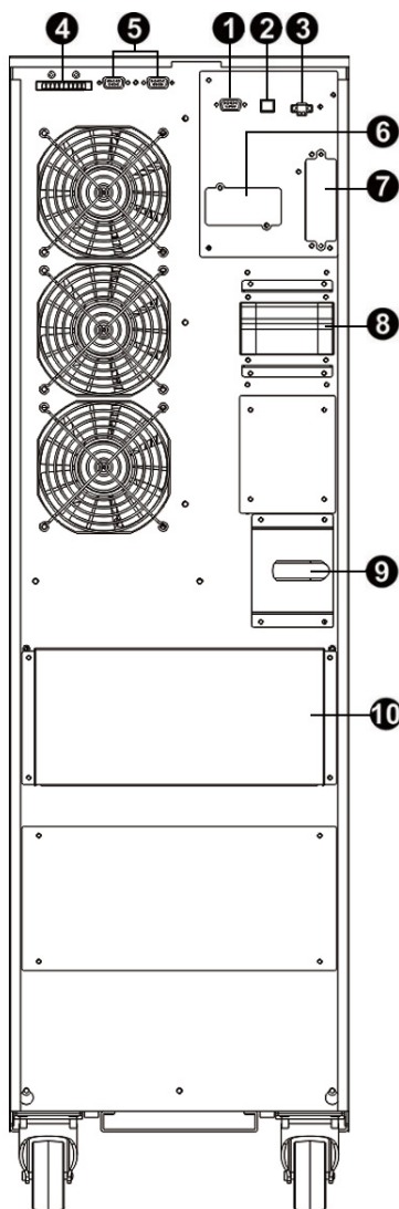
Panel Posterior del S3M40KX
