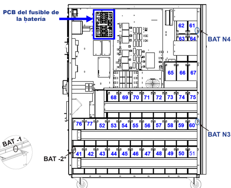
Lado Derecho S3M30KX/S3M40KX
