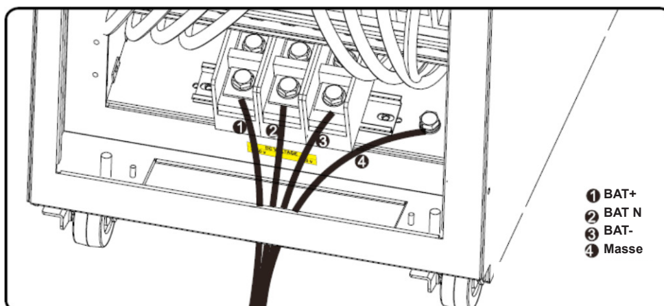
Raccordement de batteries externes pour les modèles S3M60KX et S3M80KX
