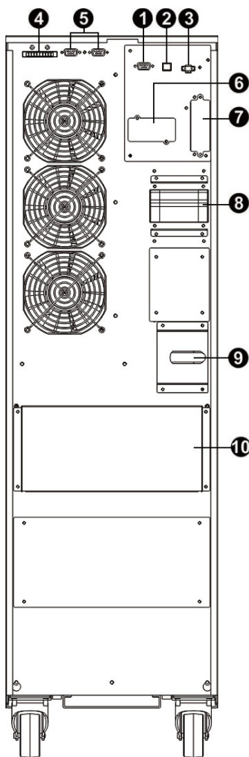
Panneau arrière du S3M40KX
