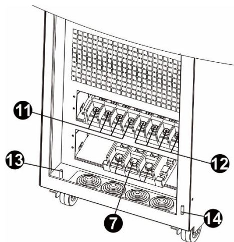
Terminales de Entrada y Salida del S3M60KX y S3M80KX
