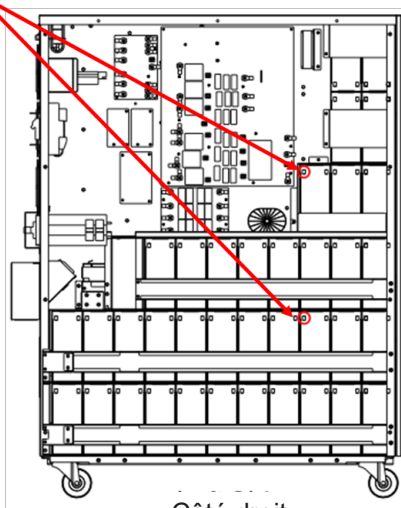
Côté droit S3M30KX/S3M40KX
