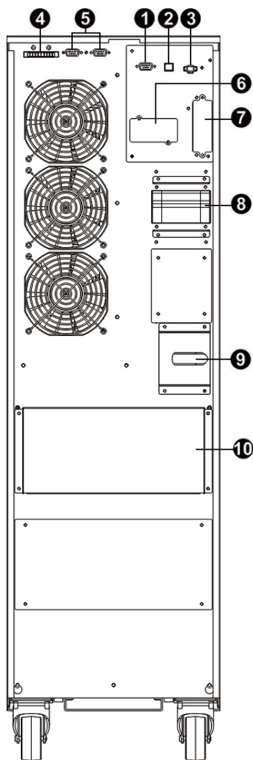
Panneau arrière du S3M30KX
