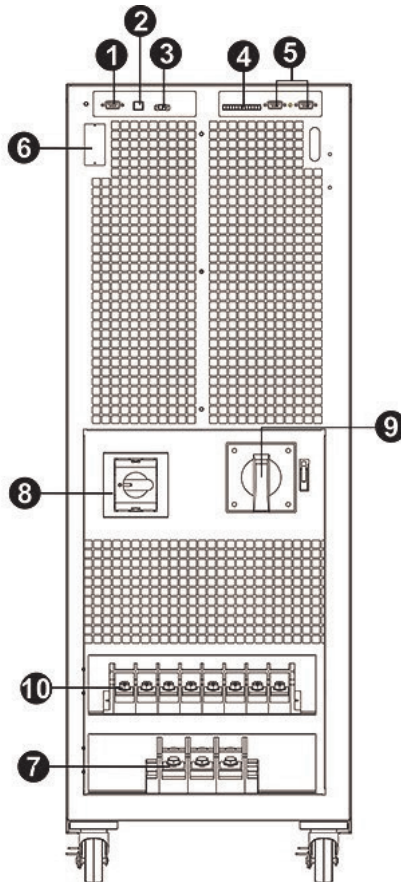
Vorderansicht S3M80KX bei geöffneter Tür Eingangs- und Ausgangsanschlüsse S3M60KX und S3M80KX
