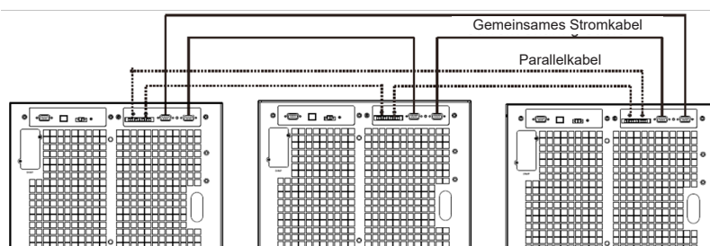
USV-Verkabelung Parallelsystem S3M60KX und S3M80KX
