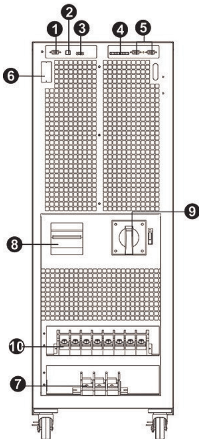
Vorderansicht S3M60KX bei geöffneter Tür
