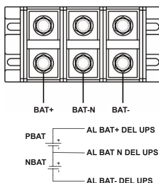
Cableado de Conexión de Batería de \pm 240V
