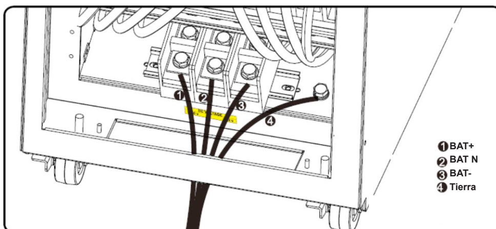
Conexión del Gabinete de Baterías Externas del S3M60KX y S3M80KX
