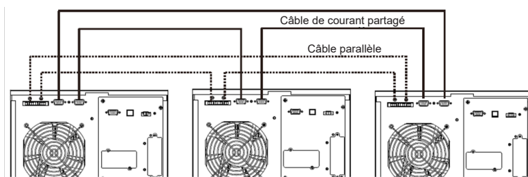
Câblage de mise en parallèle des onduleurs S3M60KX et S3M80KX
