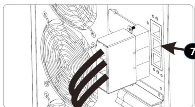
Conexión de Baterías Externas de S3M30KX/NIB y S3M40KX/NIB
