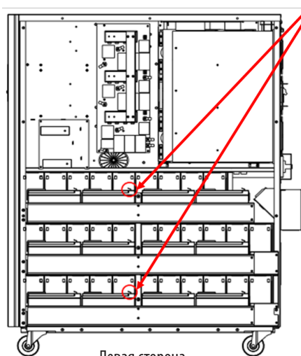
Левая сторона S3M30KX/S3M40KX
