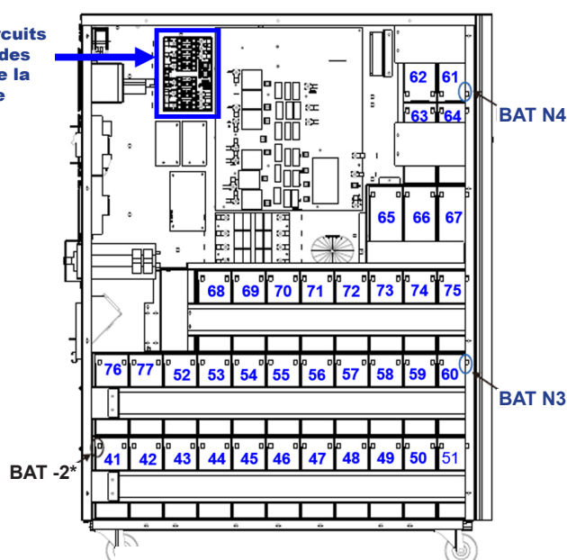
Côté droit S3M30KX/S3M40KX
