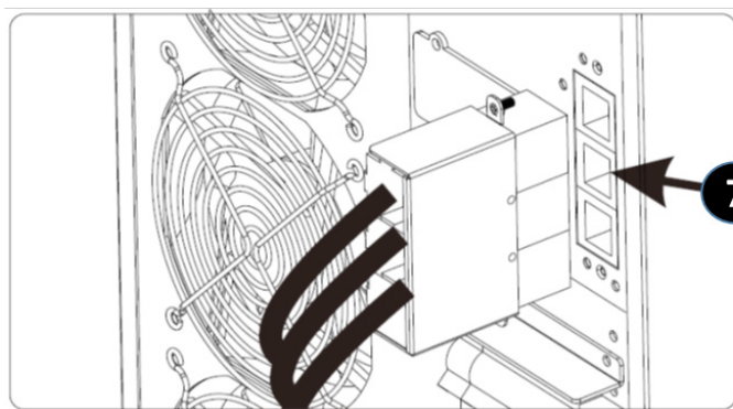
Подключение внешних батарей к ИБП мод. S3M30KX/NIB и S3M40KX/NIB
