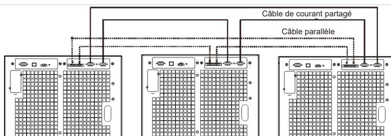
Câblage de mise en parallèle des onduleurs S3M60KX et S3M80KX
