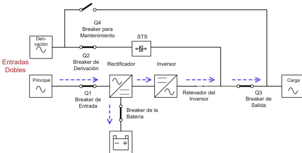
Diagramas del Modo en Línea
