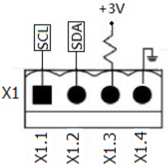
Abbildung 5.2 Anschluss Batterietemperaturdetektor
