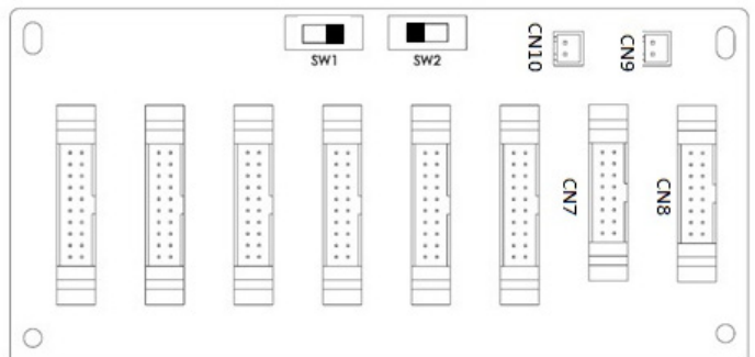
Abbildung 3.11 UPS 2 Parallele Platine
