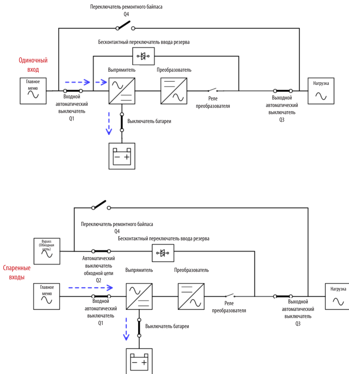
Схемы работы в режиме Standby (ожидание)
