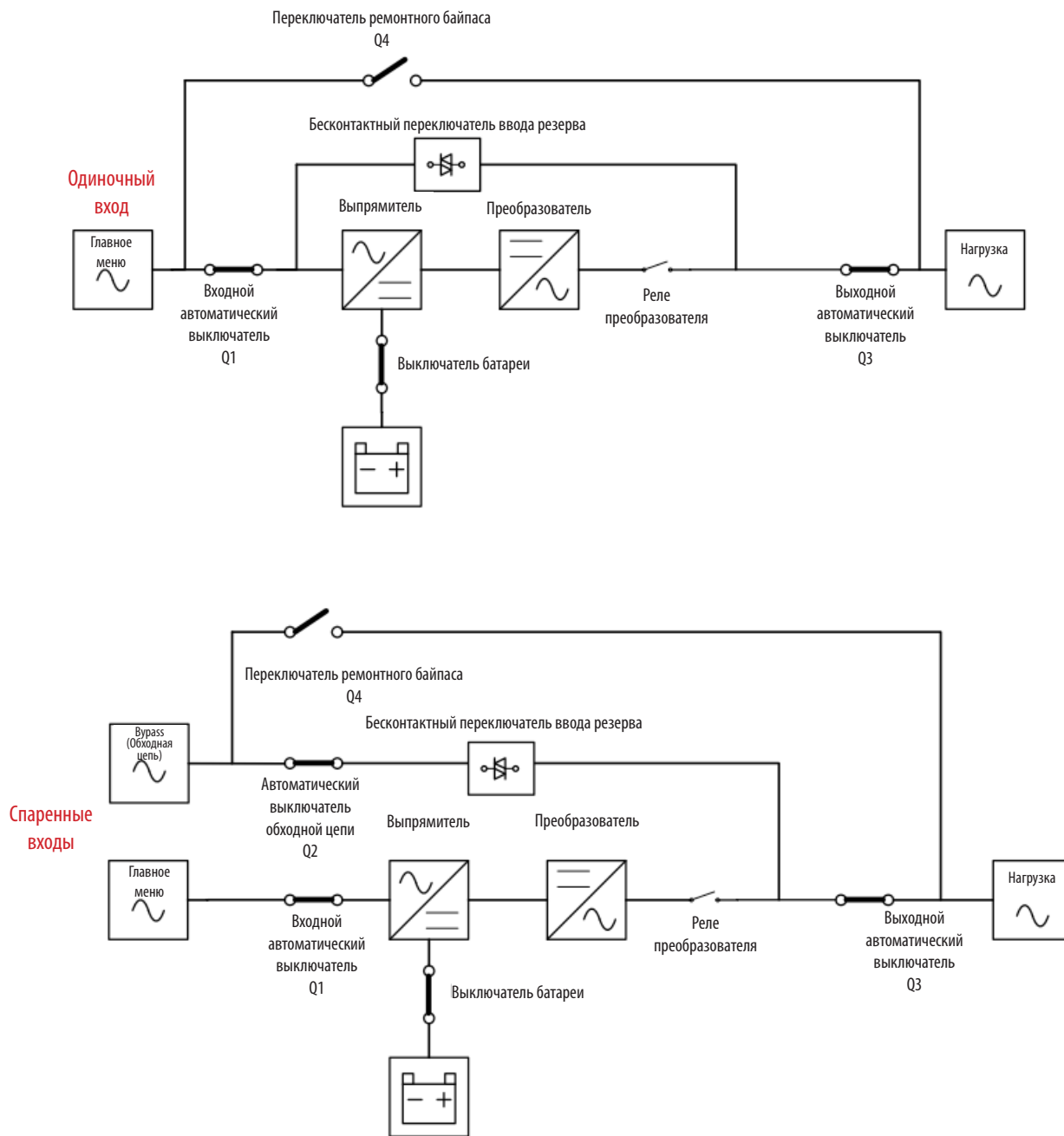
Схемы работы в режиме отключения
