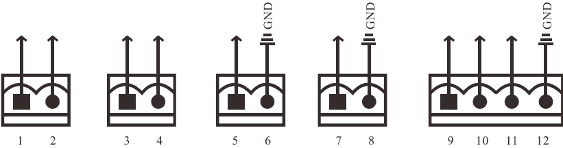
Figura 3-7 Clavijas de puertos de contacto seco
