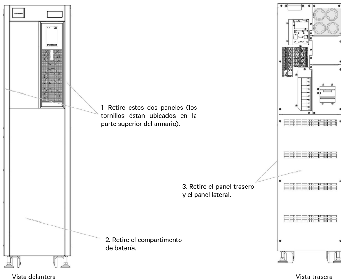
Figura 8-1 Retirada de las cubiertas correspondientes
