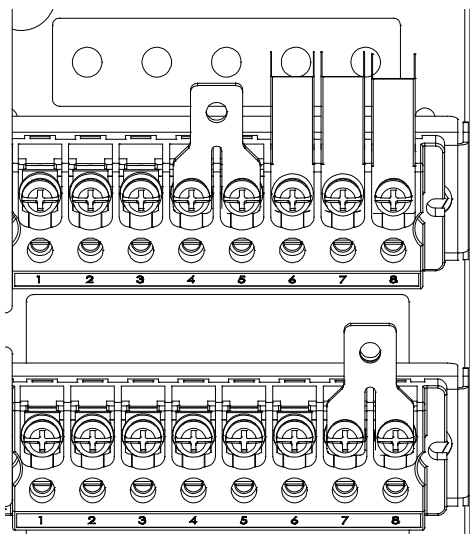
Figura 3-5 Entrada trifásica, salida trifásica; conexión del cable de configuración del bypass separado.
