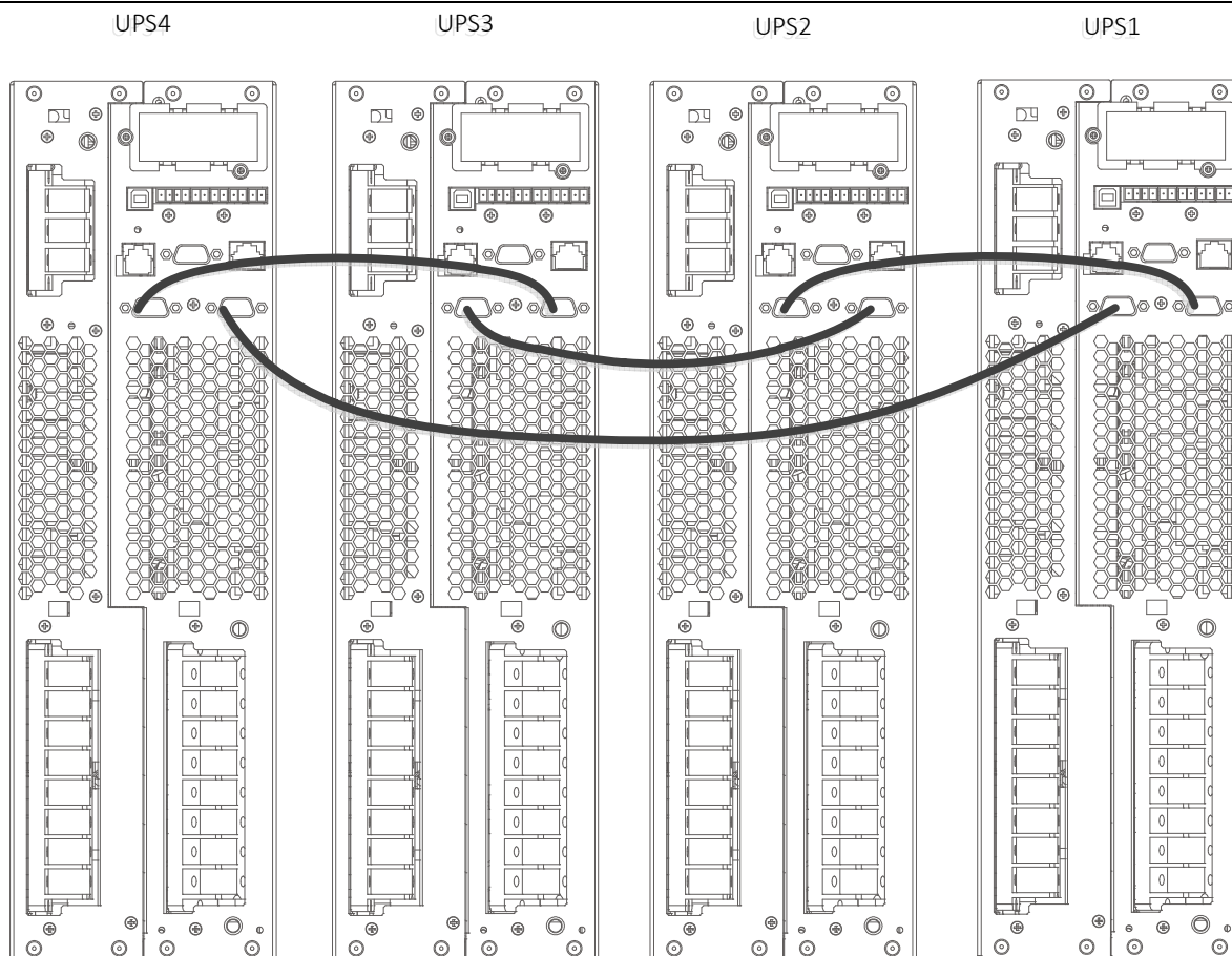
Figura 7-2 Conexiones del cable de señal paralelo (sistema paralelo)
