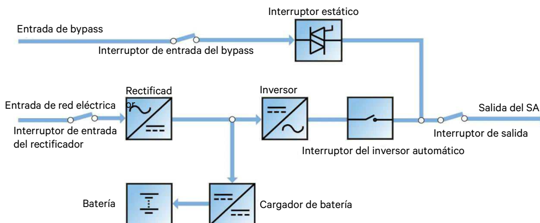
Figura 1-7 Diagrama de línea de modo operativo ECO
