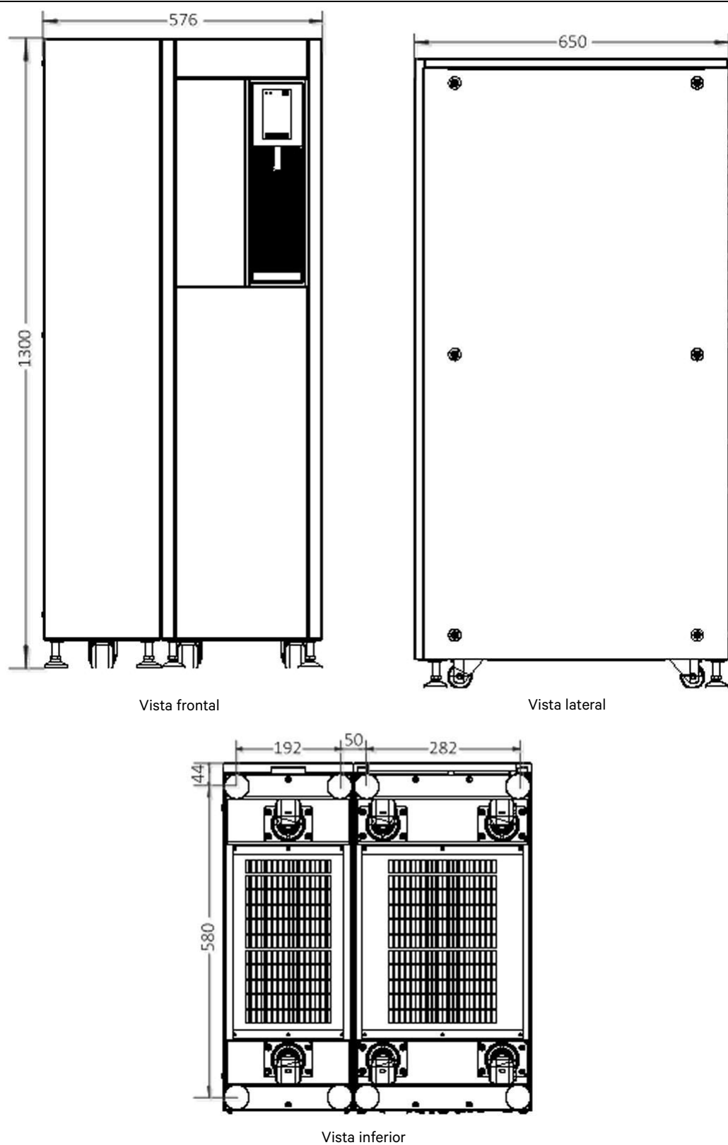
Figura 2-5 Vista frontal/lateral/inferior del SAI con armario lateral (unidad: mm)
