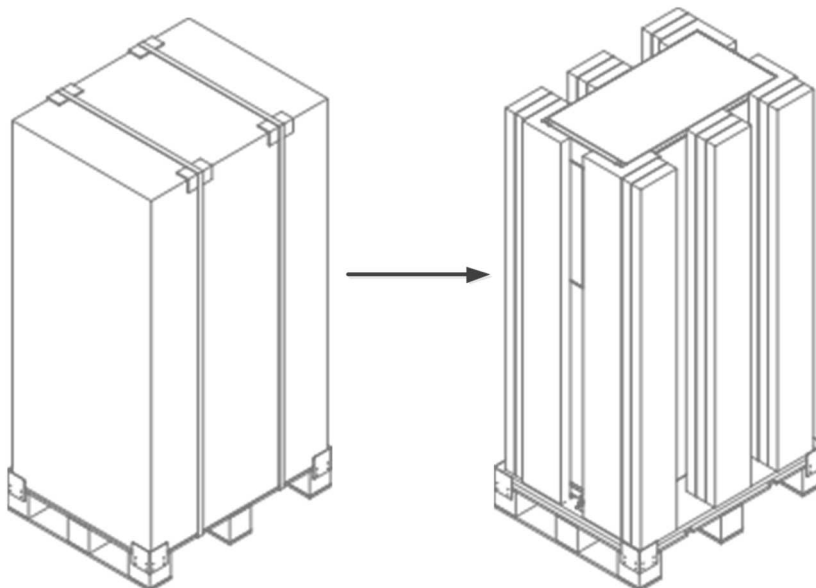
Retirada del cartón del SAI estándar
