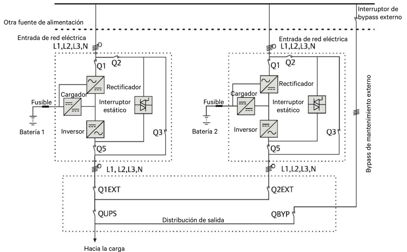
Figura 7-1 Diagrama de circuito del típico sistema en paralelo (con entrada común, baterías separadas y salida)
