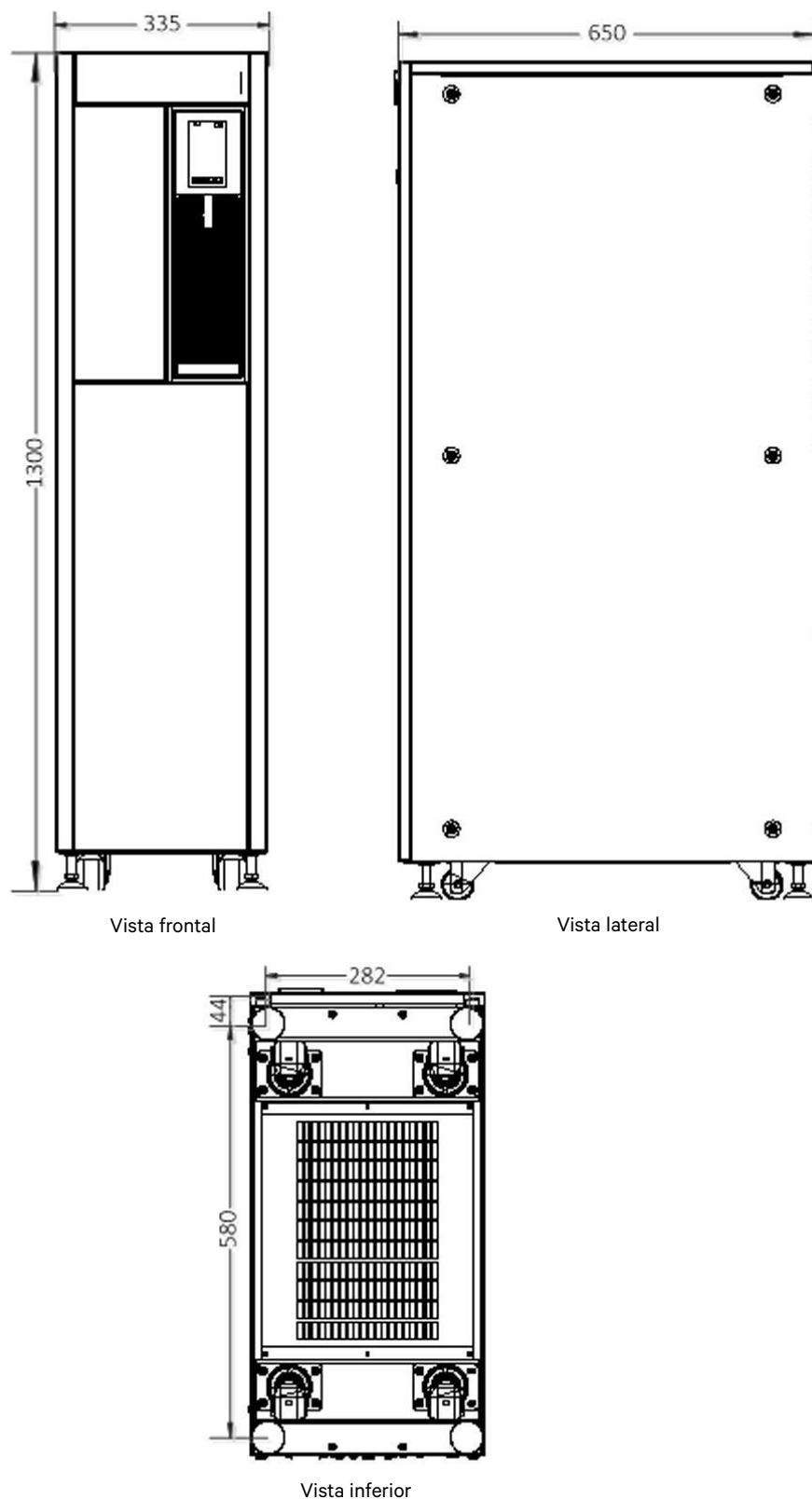
Figura 2-4 Vista frontal/lateral/inferior del SAI estándar (unidad: mm)
