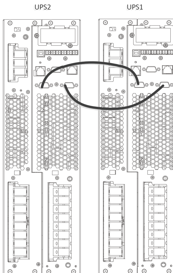
Figura 7-5 Conexiones de cable de LBS
