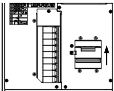
Figura 5-13 Movimiento del deflector hacia arriba
