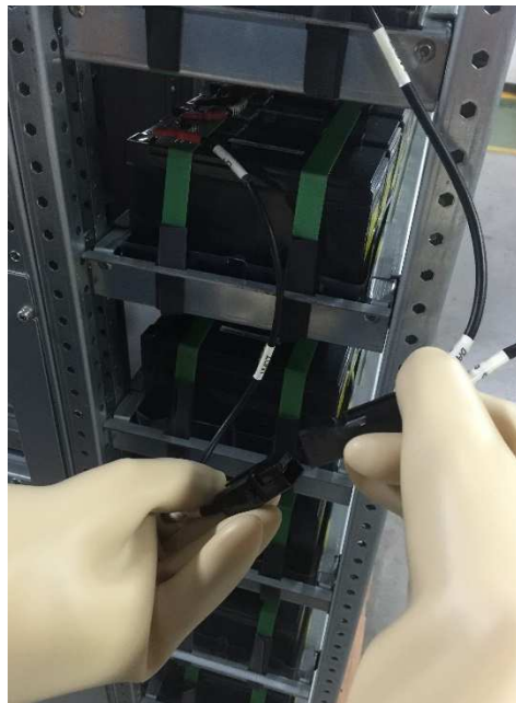
Figura 6-2 Diagrama esquemático para desconectar los terminales de batería interna.
