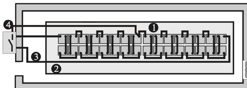
Figura 6-1 Diseño de la sala de baterías
