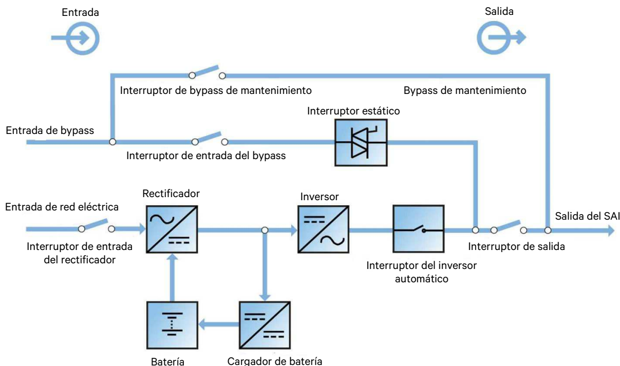
Figura 1-1 Diagrama de bloques que ilustra el principio operativo del módulo individual del SAI.
