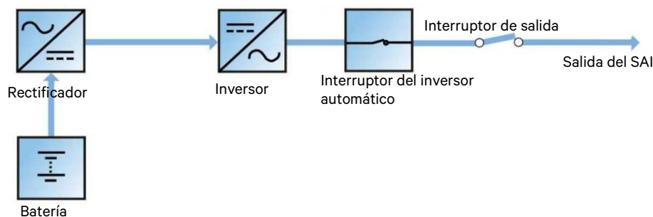
Figura 1-4 Diagrama de línea de modo operativo de batería
