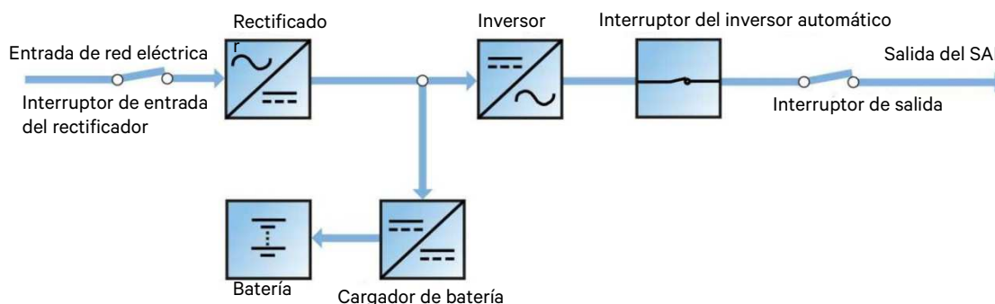
Figura 1-3 Diagrama de línea de modo operativo normal
