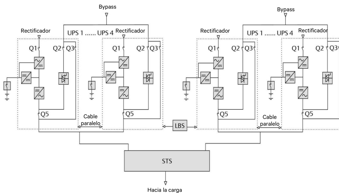
Figura 7-4 Sistema LBS (módulo en paralelo)
