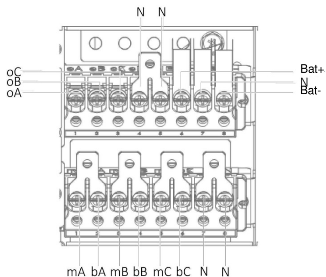
Figura 3-2 Terminales de conexión de cable de alimentación (vista trasera)
