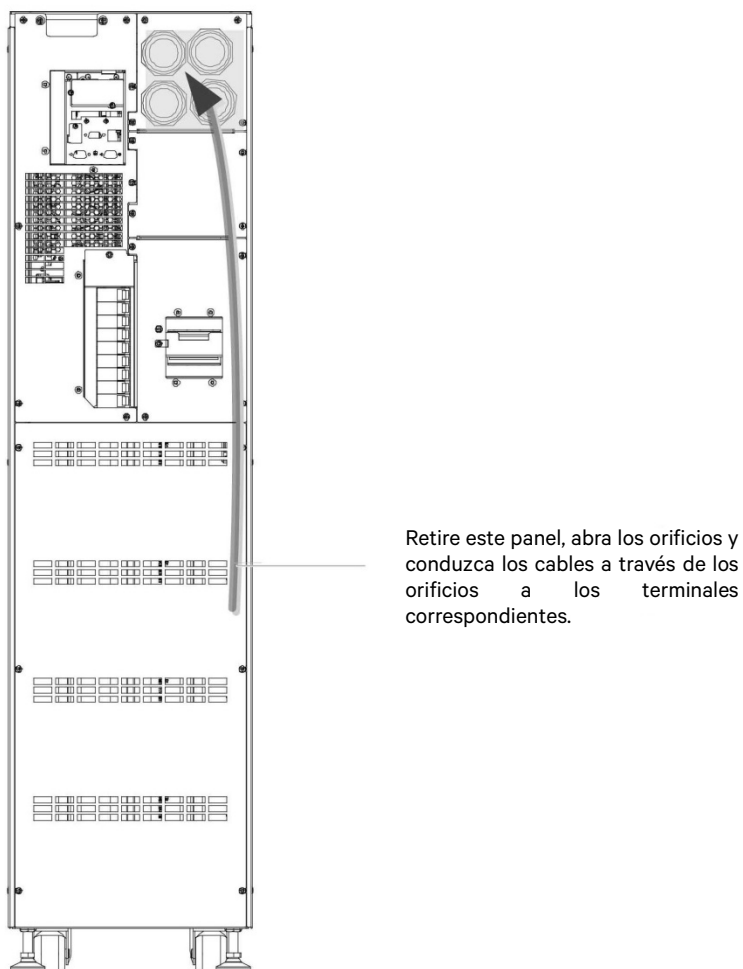
Figura 3-2 Terminales de conexión de cable de alimentación (vista trasera)
