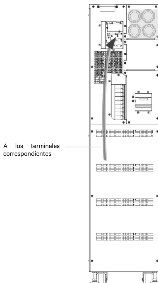
Figura 3-10 Colocación de cables de señal (acceso a cable trasero).
