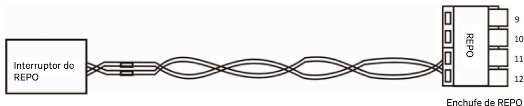
Figura 3-8 Conexión del cable de REPO
