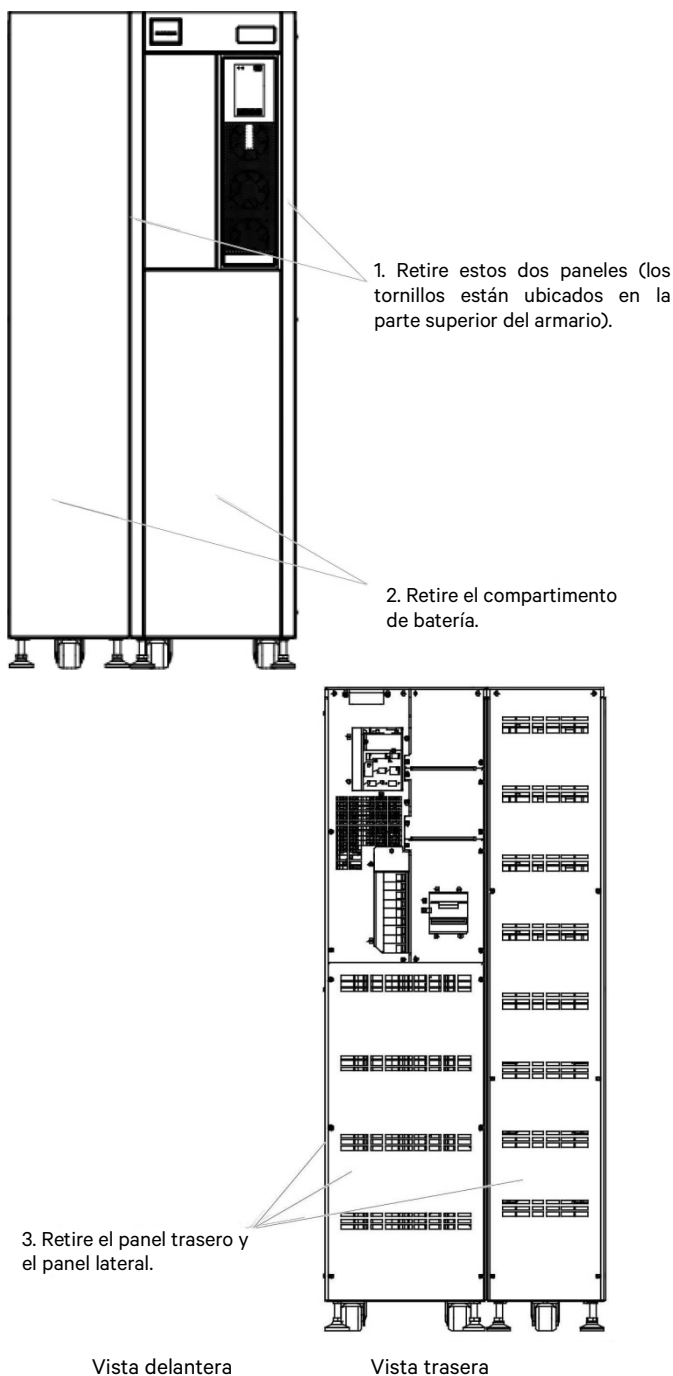
Figura 8-3 Retirada de las cubiertas correspondientes
