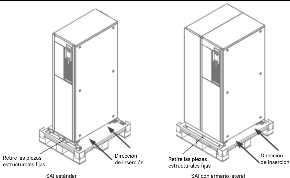
Figura 2-2 Retirada del palé inferior
