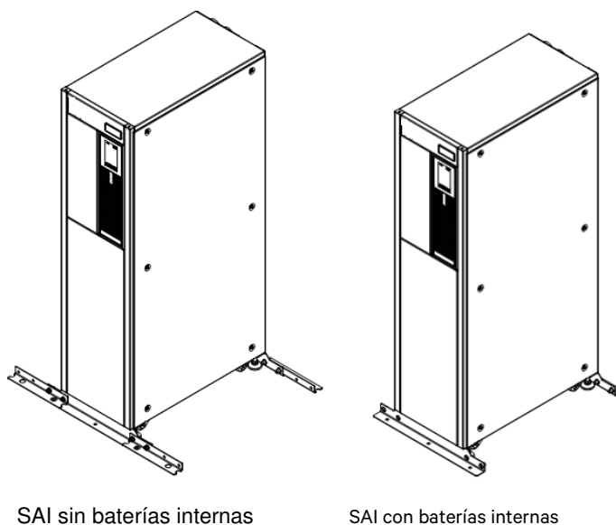
Figura 2-3 Instalación completa
