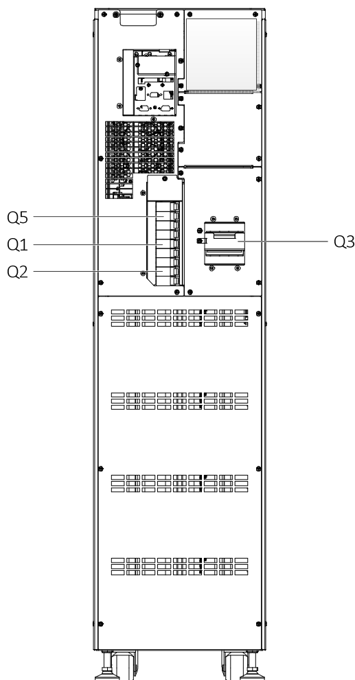
Figura 5-1 Interruptor de suministro de alimentación del SAI
