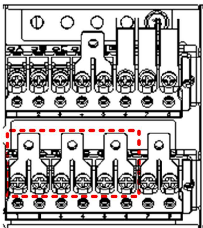
Figura 8-18 Entrada trifásica y salida monofásica, configuración de bypass separado (1)
