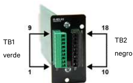
Figura 8-8 Ubicación y numeración de las clavijas
