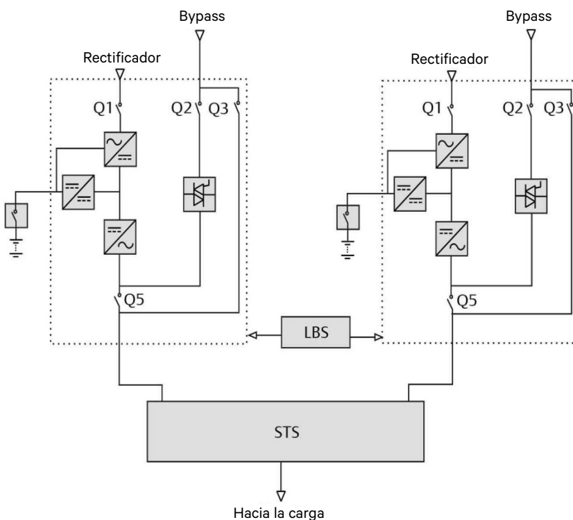
Figura 7-3 Sistema LBS (módulo SAI)
