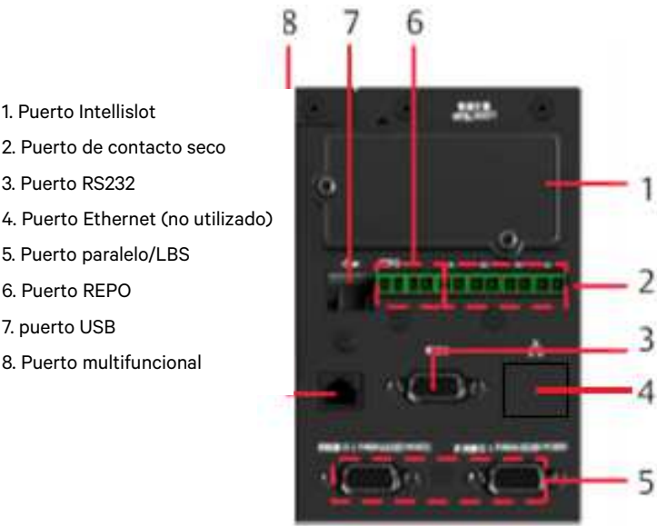
Figura 3-6 Ilustración de los puertos de la caja de comunicación
