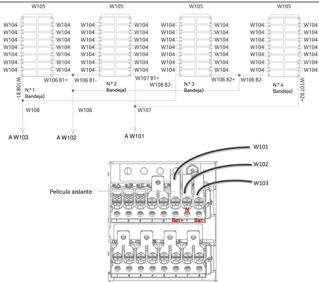
Figura 8-2 Instalación de baterías internas del SAI estándar
