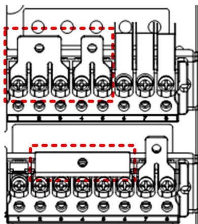
Figura 8-19 Entrada trifásica y salida monofásica, configuración de bypass separado (2)
