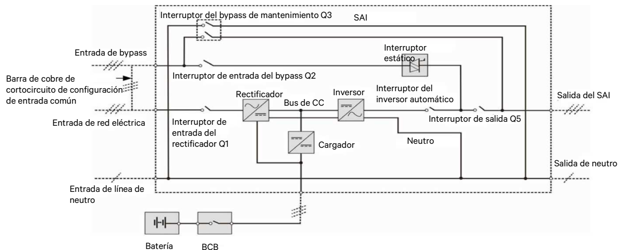
Figura 1-2 Configuración de interruptor de suministro de alimentación del SAI
