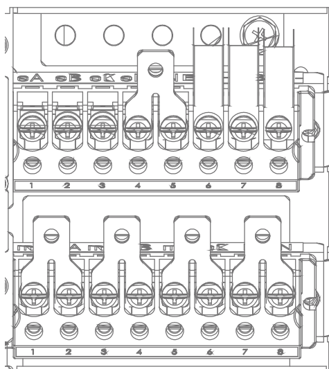
Figura 3-4 Entrada trifásica y salida trifásica, conexión del cable de configuración de entrada común (ajustes predeterminados de fábrica)
