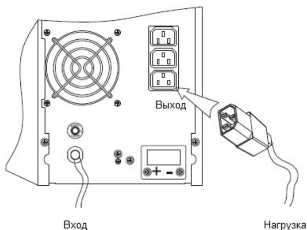
Схема подключения для моделей 1кВА - 3кВА
