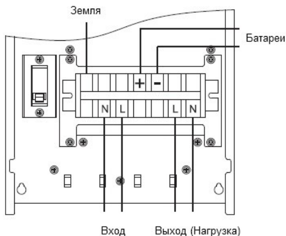
Схема подключения для моделей 6кВА и 10кВА
