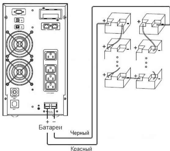
Схема подключения внешних батарей для ИБП 1кВА - 3кВА
