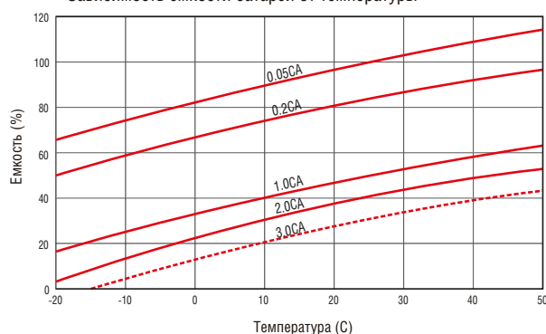
Зависимость емкости батареи от температуры
