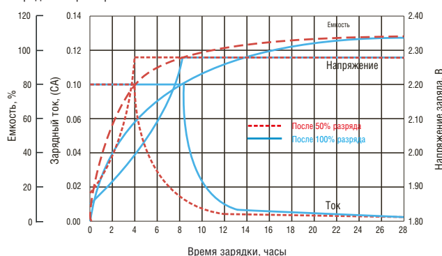
Зарядные характеристики
