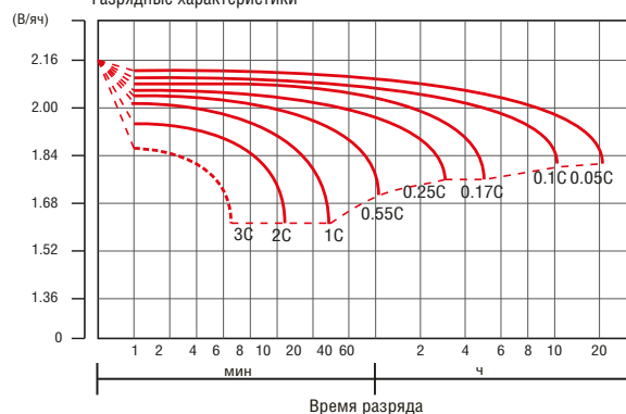
Разрядные характеристики
