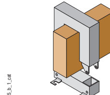
ТТ с окном для кабеля и разъемным сердечником
