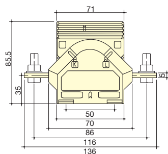
TRB 135 (для 125 и 150 A)
