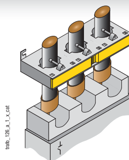
Трехфазный ТТ с окном для кабеля или шины
